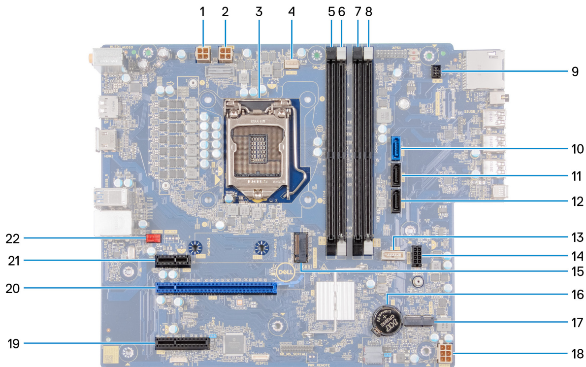
Figur 1. Komponenter på moderkortet
