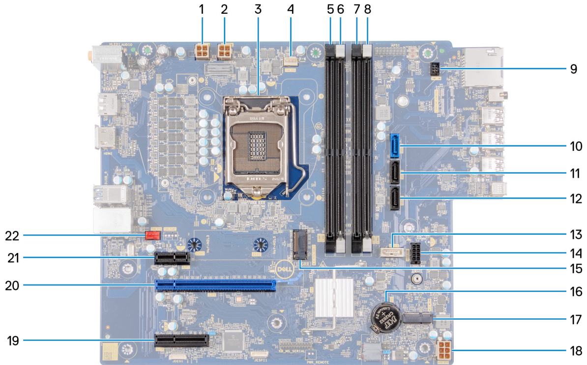
그림 2. 시스템 보드 구성 요소
