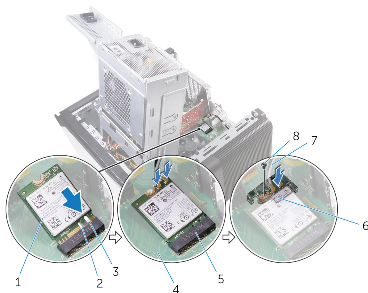
Obrázok 39. Spätná montáž karty bezdrôtovej komunikácie
