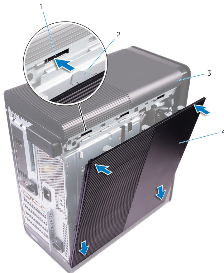
Figura2. Voltar a colocar a tampa do lado direito
