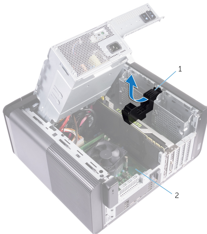
Figura22. Retirar o suporte da placa gráfica de tamanho completo
