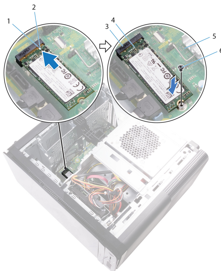
Figura16. Voltar a colocar a unidade de estado sólido
