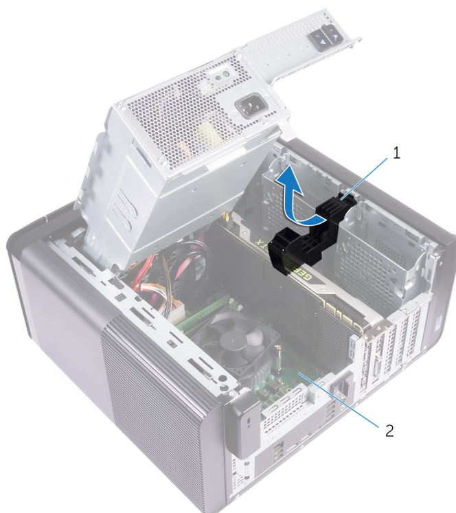
図 22. フルレンジグラフィックスカードブラケットの取り外し
