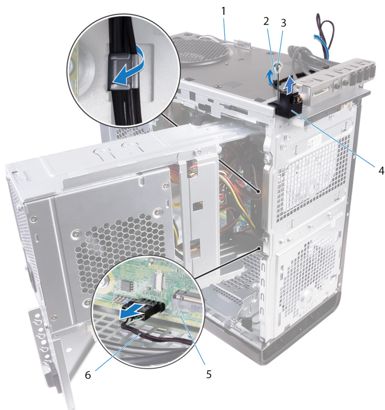
26. ábra. Bekapcsológomb-modul kábelének leválasztása
