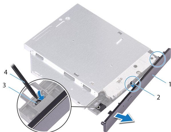
9. ábra. Az optikai meghajtó előlapjának eltávolítása
