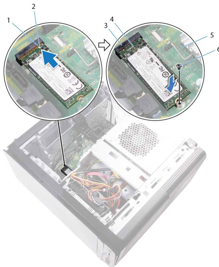
16. ábra. Az SSD meghajtó visszahelyezése
