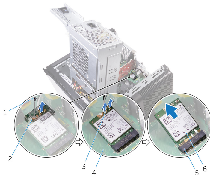
38. ábra. A vezeték nélküli kártya eltávolítása
