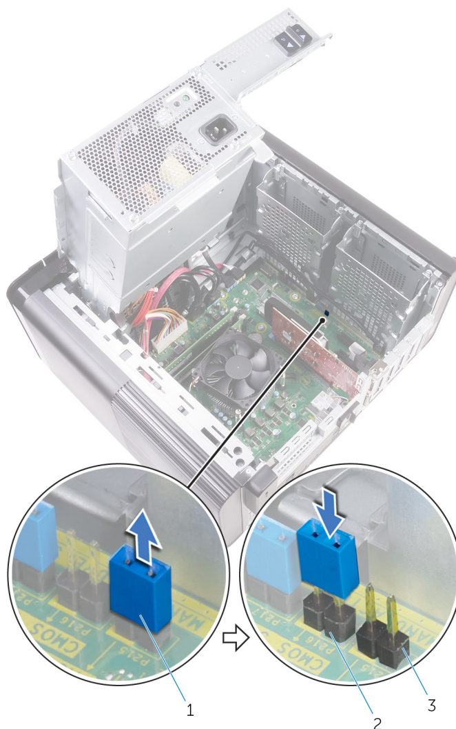
Figure 43. Effacement des paramètres CMOS
