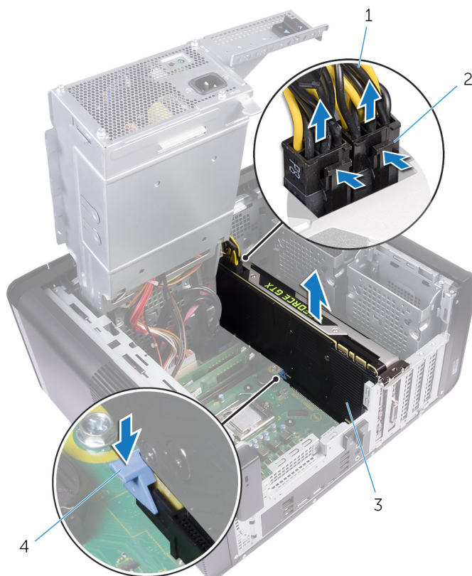
Figure 23. Retrait des câbles d'alimentation
