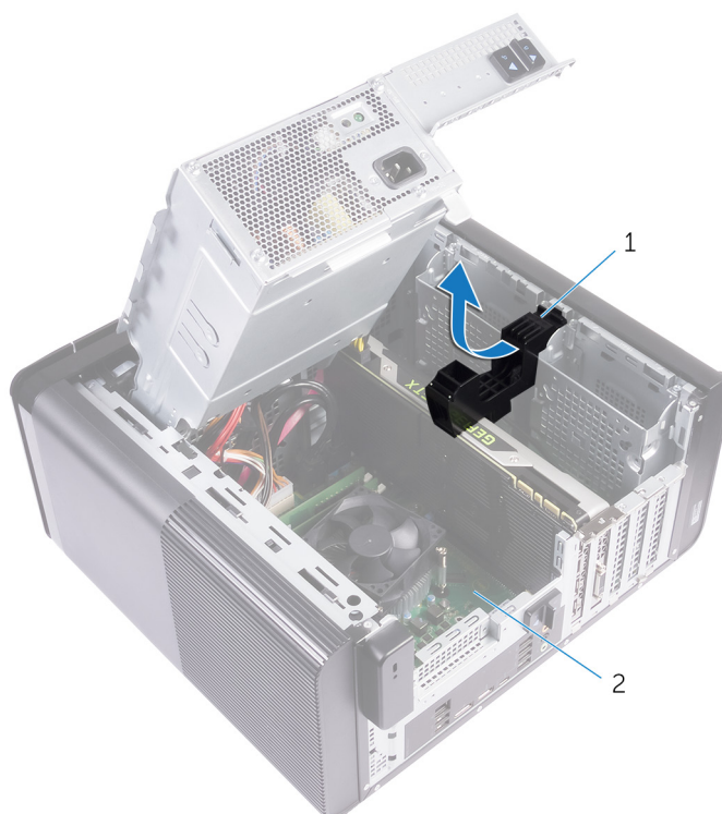
Figure 22. Retrait du support de la carte graphique pleine longueur
