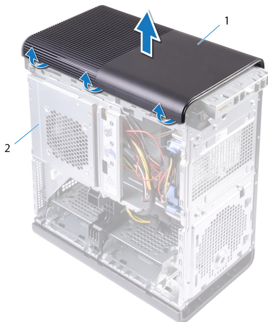
Figure 10. Retrait du capot supérieur de l'ordinateur.
