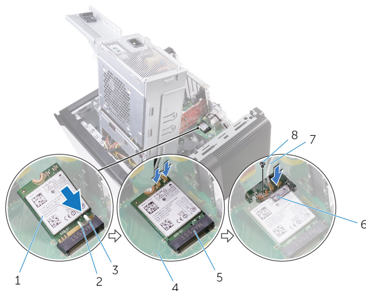
Figure 39. Remise en place de la carte sans fil
