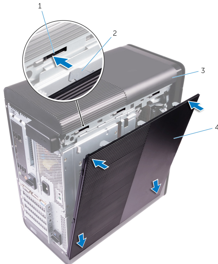
Figure 2. Remise en place du panneau latéral droit
