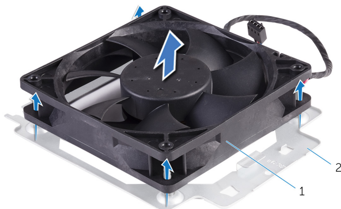
Figure 35. Retrait du ventilateur du châssis
