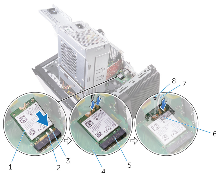
Abbildung 39. Wiedereinbauen der Wireless-Karte
