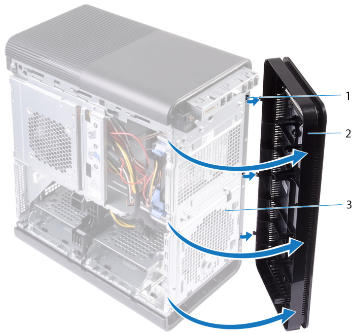
Abbildung 4. Entfernen der Frontverkleidung
