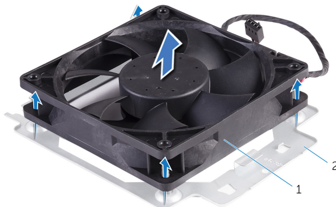
Figura 37. Scoaterea ventilatorului carcasei
