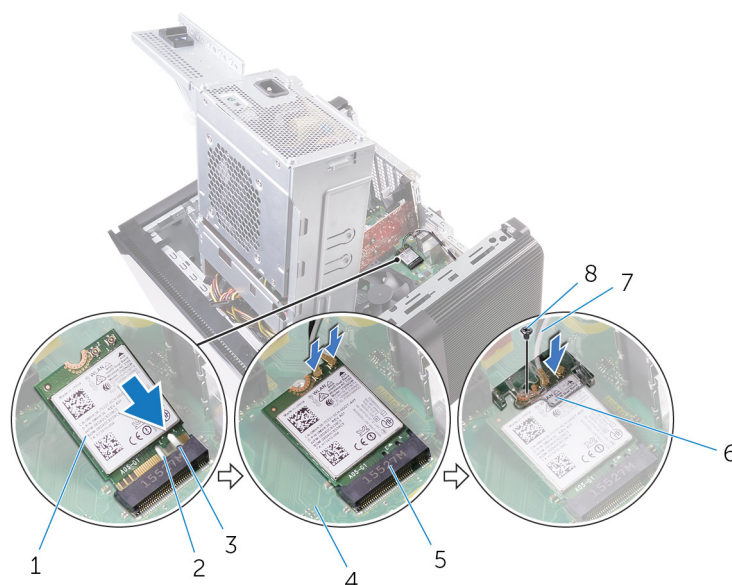
Figura 41. Remontarea cardului wireless
