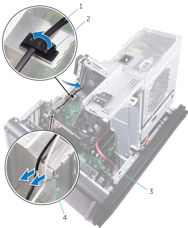
Afbeelding 42. De antennekabels ontkoppelen
