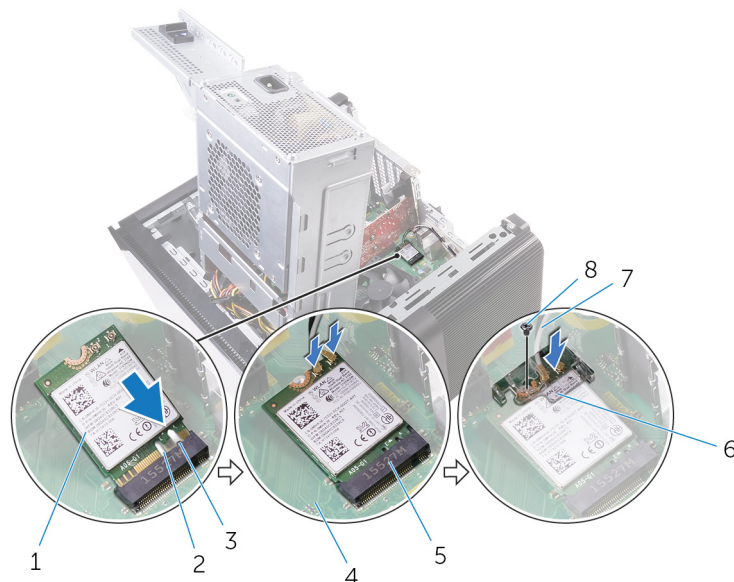
Afbeelding 41. De draadloze kaart vervangen
