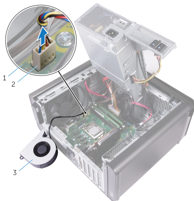
Afbeelding 33. De ventilorkabel verwijderen
