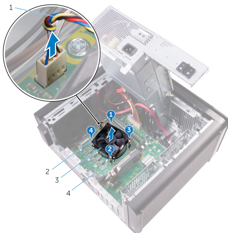
Obrázek 35. Demontáž ventilátoru procesoru a chladiče
