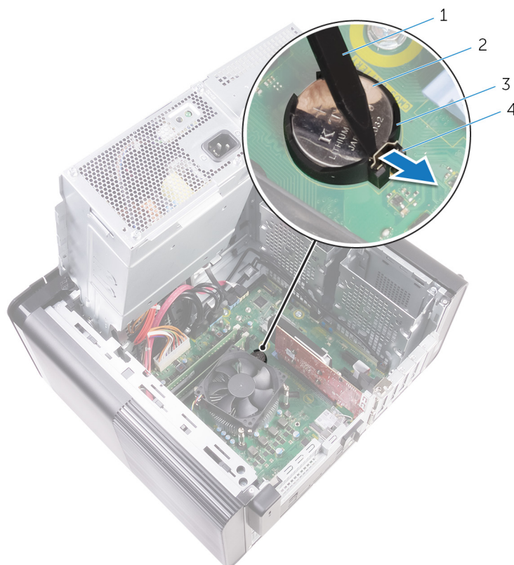
Obrázek 22. Demontáž knoflíkové baterie
