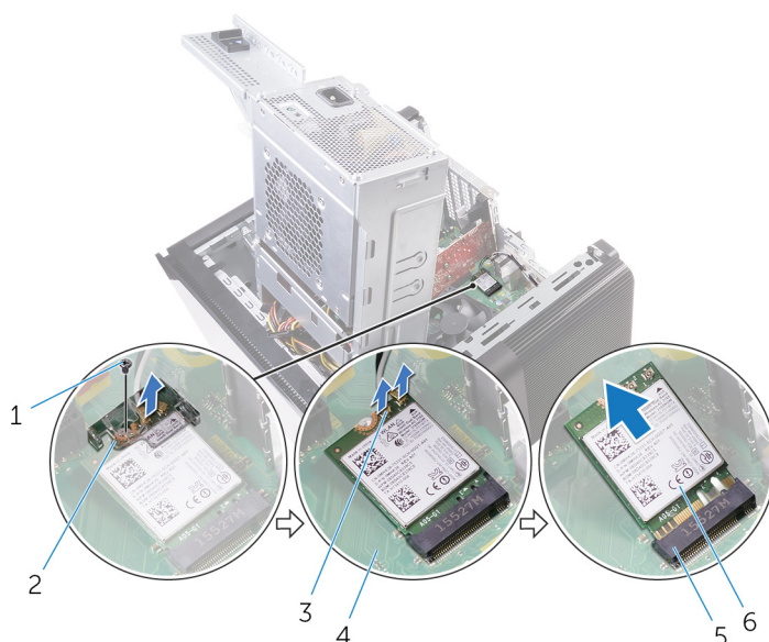
Obrázok 40. Demontáž karty bezdrôtovej komunikácie
