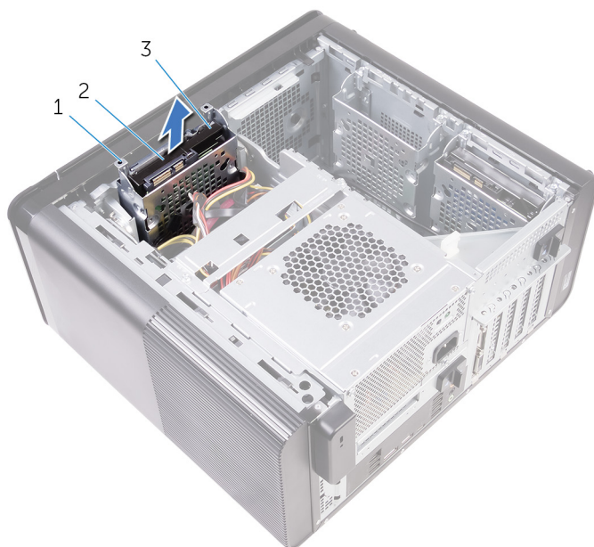
Figura15. Retirar o suporte da unidade de disco rígido
