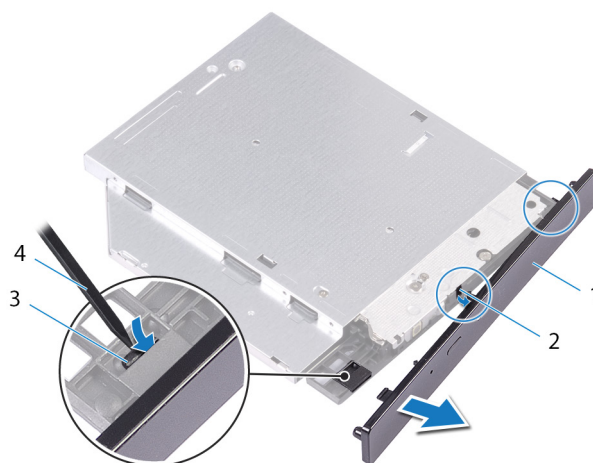
Figura9. Retirar a moldura da unidade ótica
