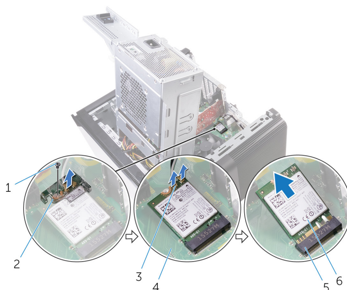
Figura40. Retirar a placa de rede sem fios
