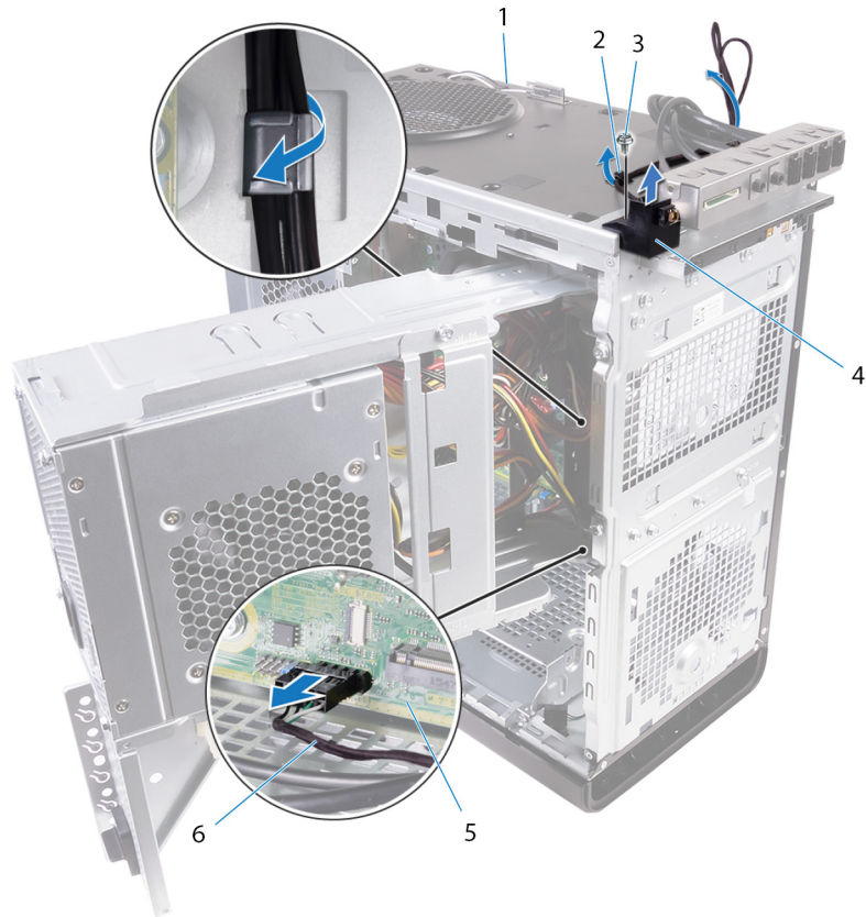
Figura28. Desligar o cabo do módulo do botão de alimentação
