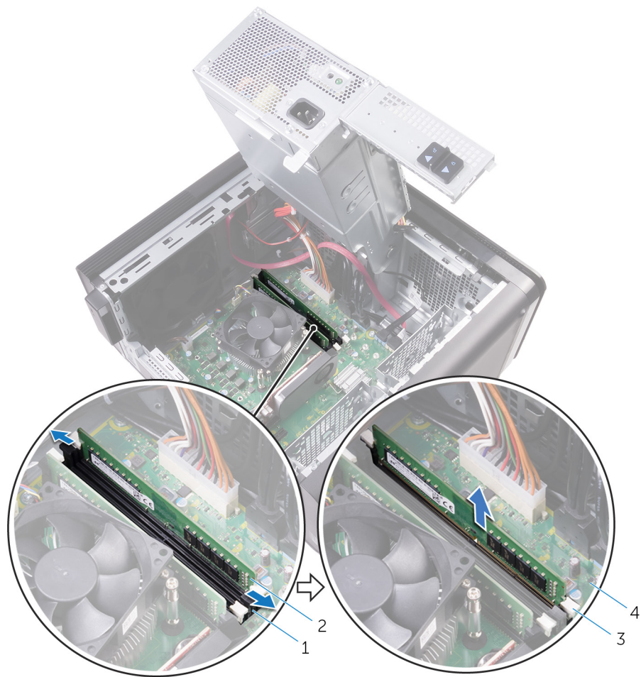
図 26. メモリモジュールの取り外し
