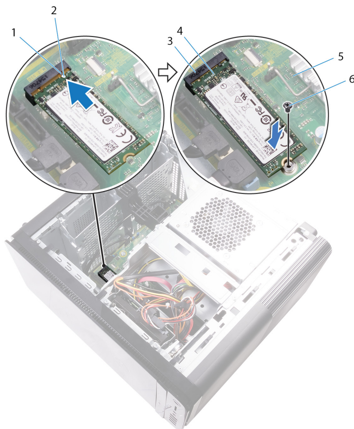
図 18. ソリッドステートドライブの取り付け
