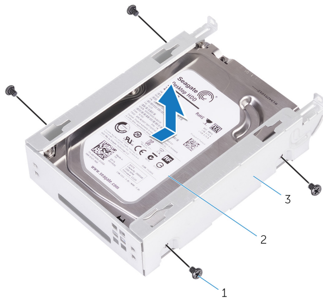
図 16. ブラケットからのハードドライブの取り外し
