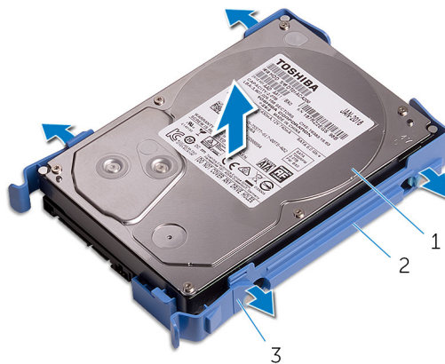
13. ábra. A merevlemez eltávolítása a tartókeretből
