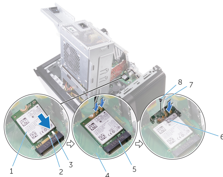
41. ábra. A vezeték nélküli kártya visszahelyezése
