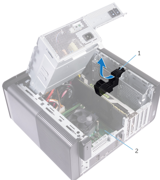
24. ábra. A teljes hosszúságú videokártya tartókeretének eltávolítása
