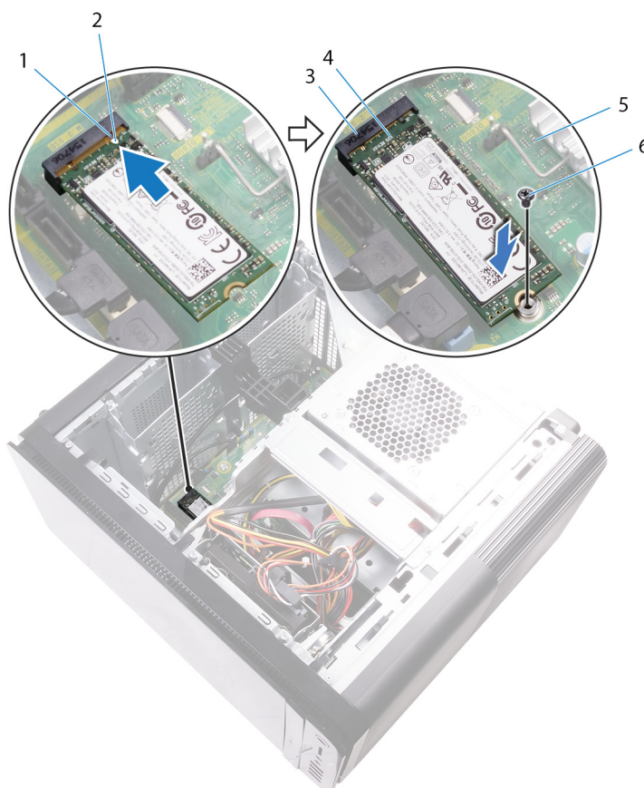
18. ábra. Az SSD meghajtó visszahelyezése
