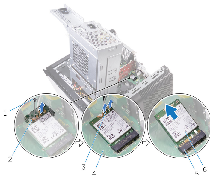
40. ábra. A vezeték nélküli kártya eltávolítása
