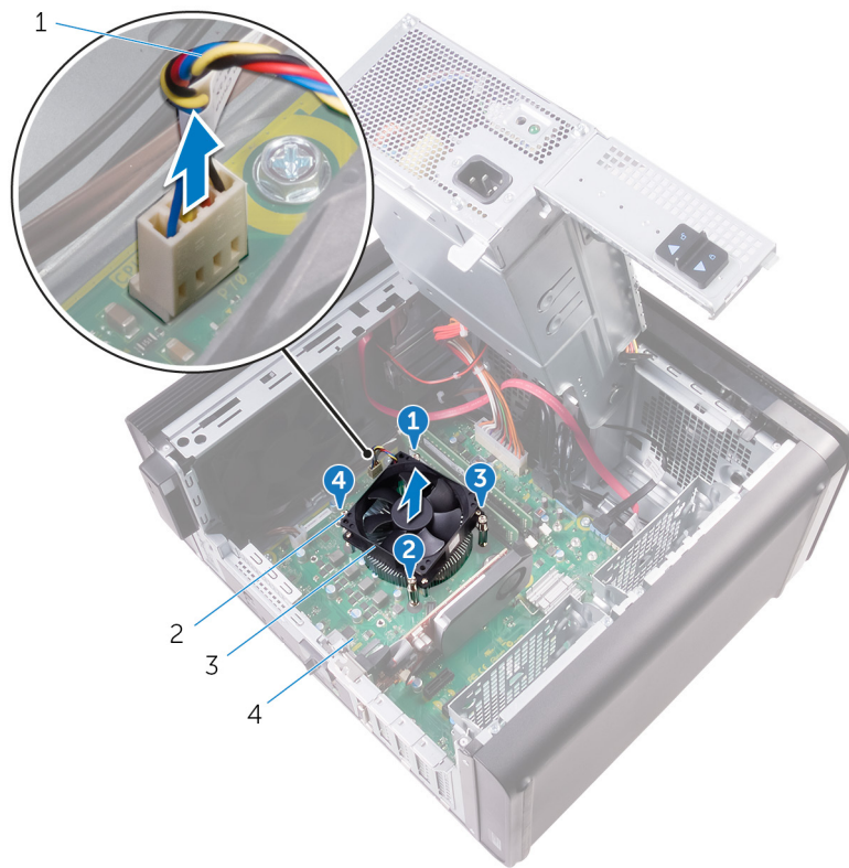
Abbildung 35. Entfernen von Prozessorlüfter und Kühlkörper
