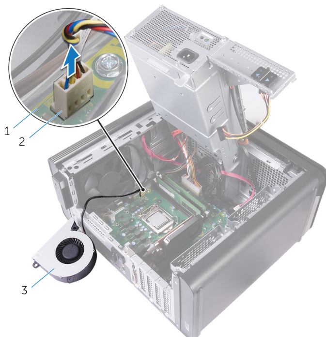
Рисунок 29. Отсоединение кабеля вентилятора
