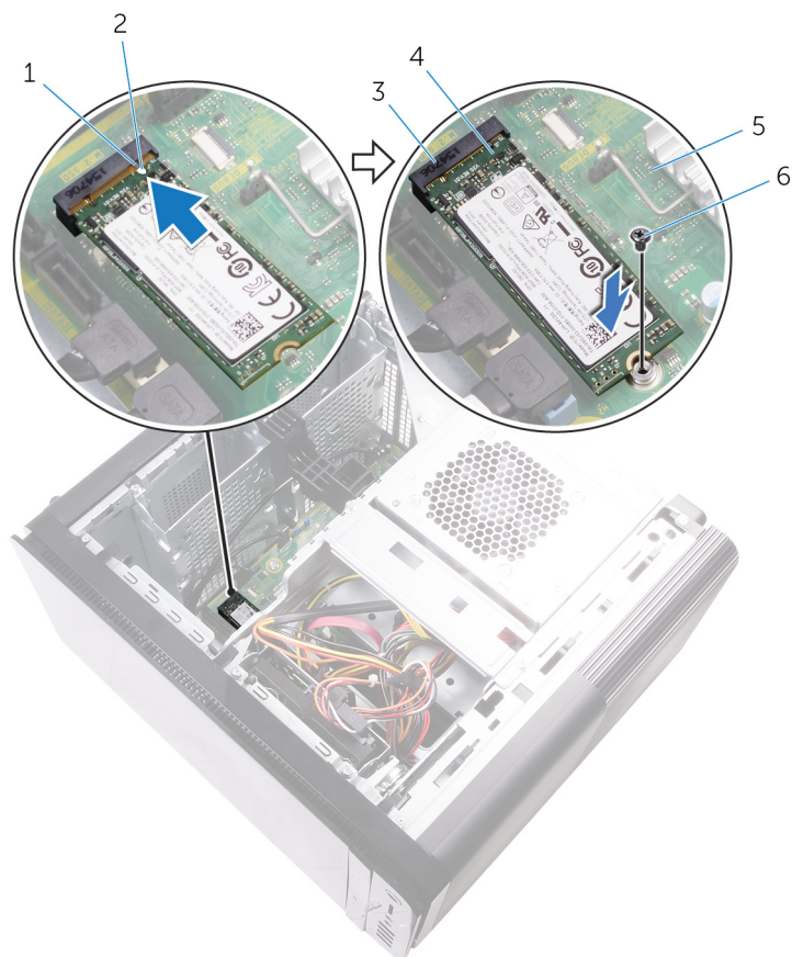
Рисунок 14. Установка твердотельного накопителя
