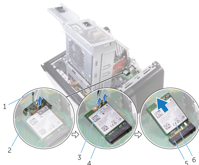
Рисунок 36. Извлечение платы беспроводной сети
