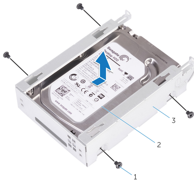
Rysunek 12. Wyjmowanie dysku twardego ze wspornika
