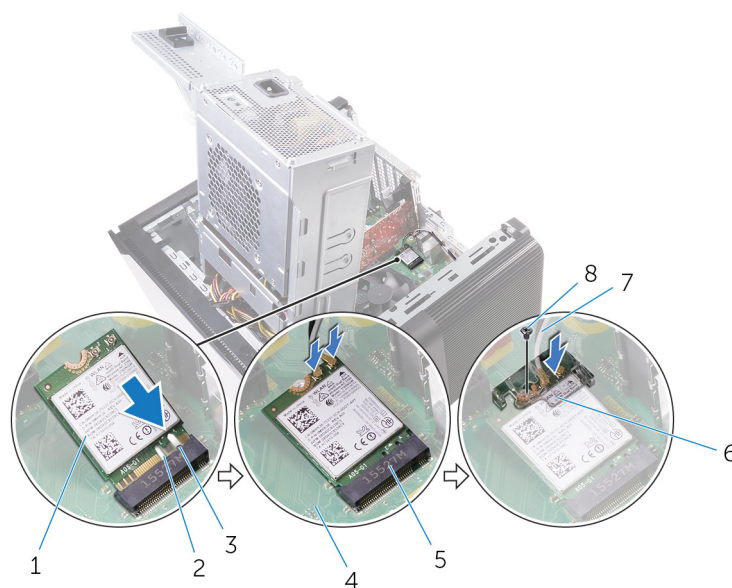
Rysunek 37. Instalowanie karty sieci bezprzewodowej
