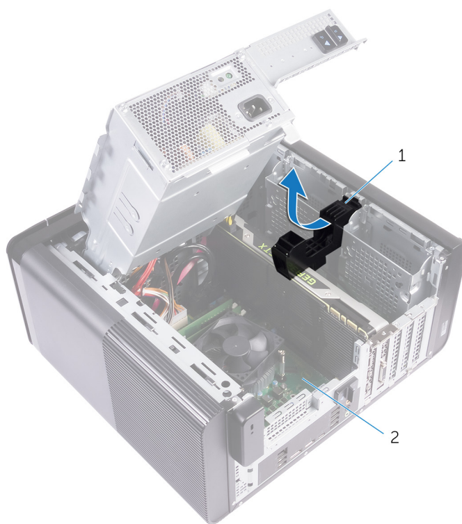
図 20. グラフィックスカードブラケットの取り外し
