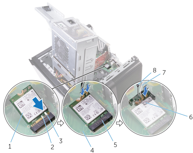
Abbildung 37. Wiedereinbauen der Wireless-Karte
