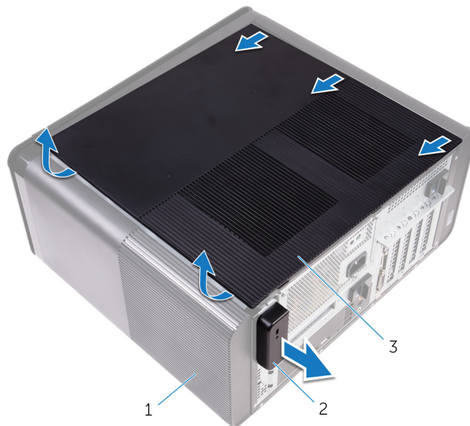
Abbildung 1. Entfernen der rechten Abdeckung
