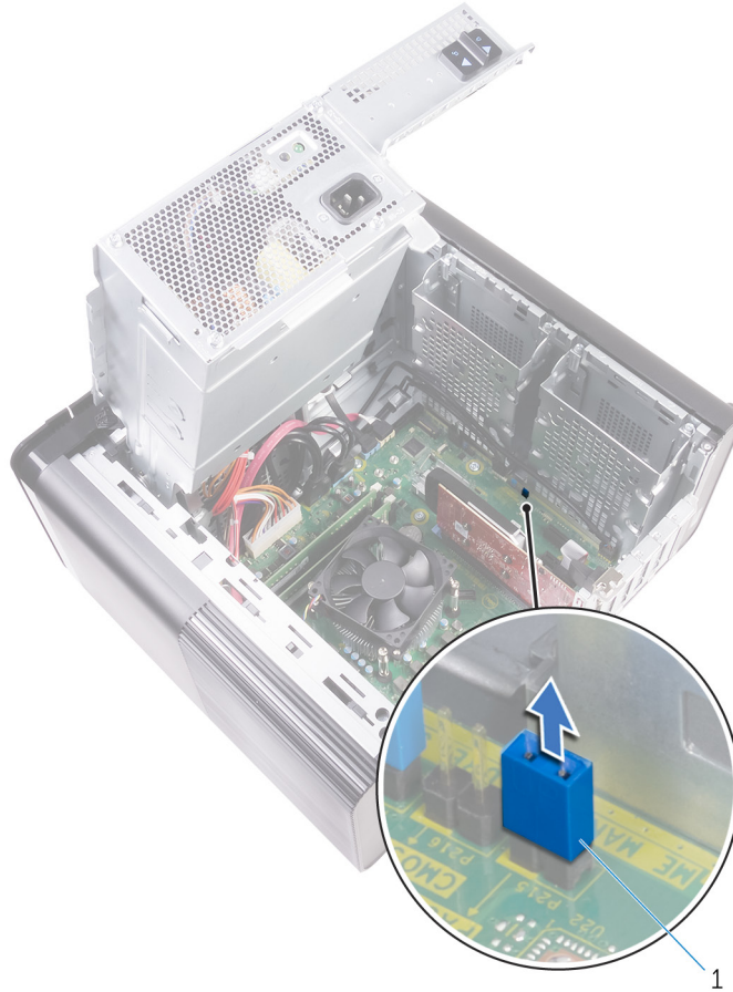
Abbildung 42. Entfernen des Jumper-Steckers
