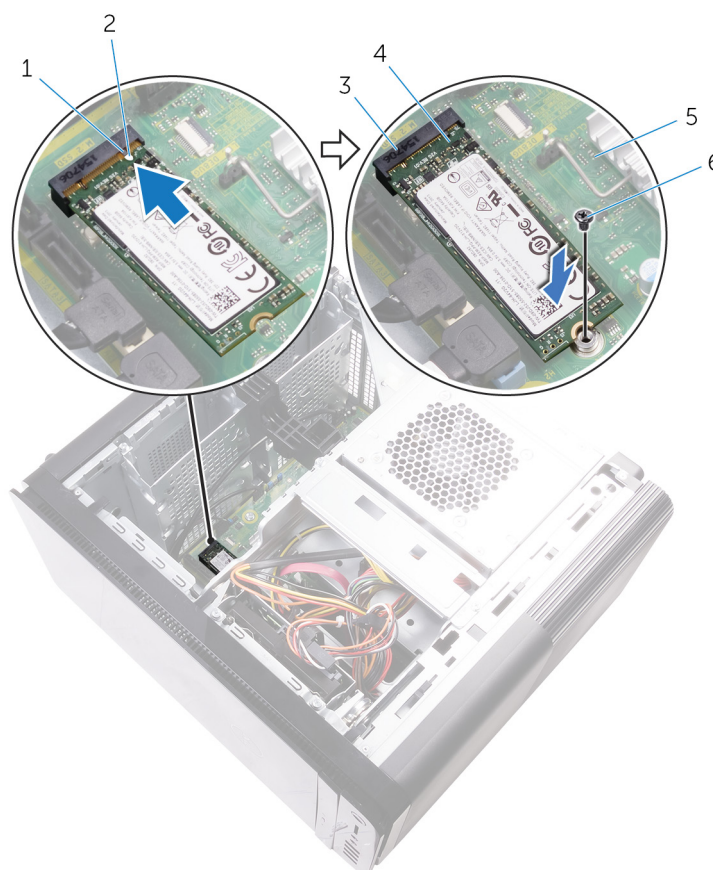
Abbildung 14. Wiedereinbauen des SSD-Laufwerks
