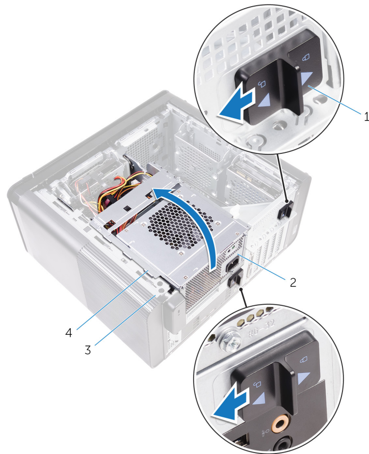
Abbildung 15. Drehen der Netzteilereinheit
