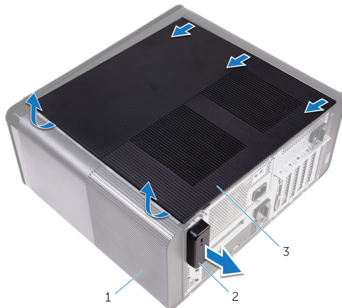
Abbildung 1. Entfernen der rechten Abdeckung
