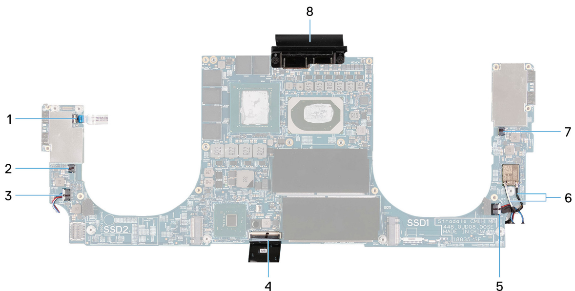
Figura 1. Cavi della scheda di sistema
