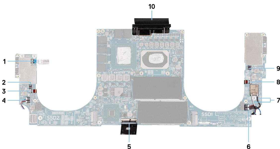
Figura2. Cabos da placa de sistema
