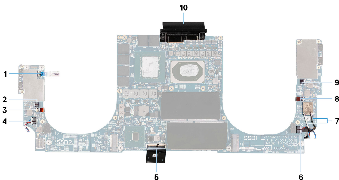
Figura1. Cabos da placa de sistema
