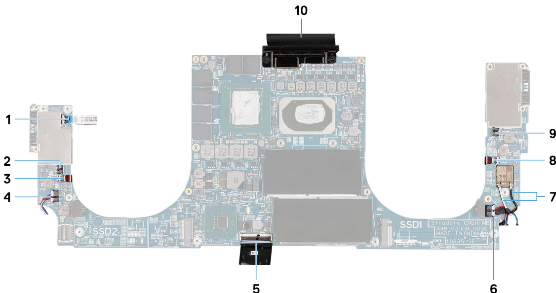
Afbeelding 1. Stroomkaartkabels
