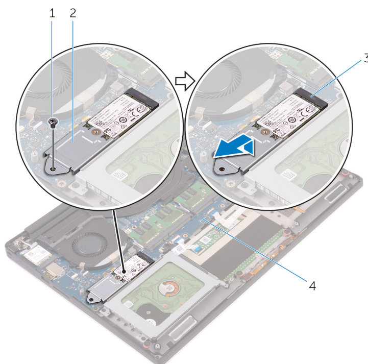
Figura 11. Como remover a placa da unidade de estado sólido
