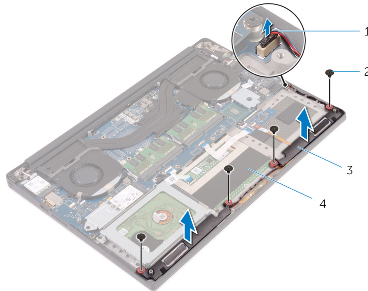
Figura 15. Como remover os alto-falantes
