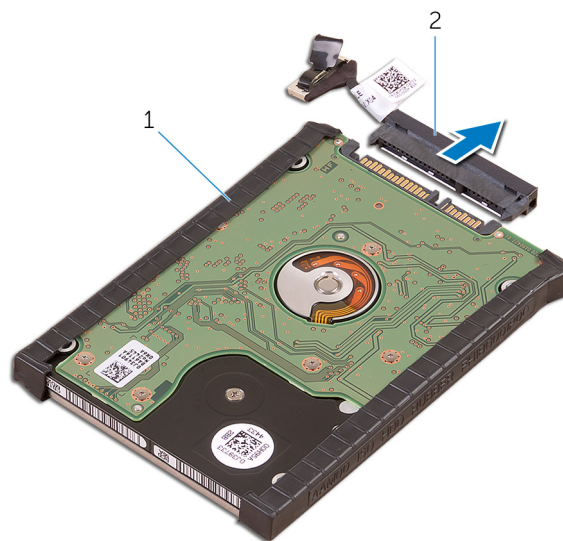
Figura 9. Como desconectar a placa intermediária do disco rígido do conjunto do disco rígido
