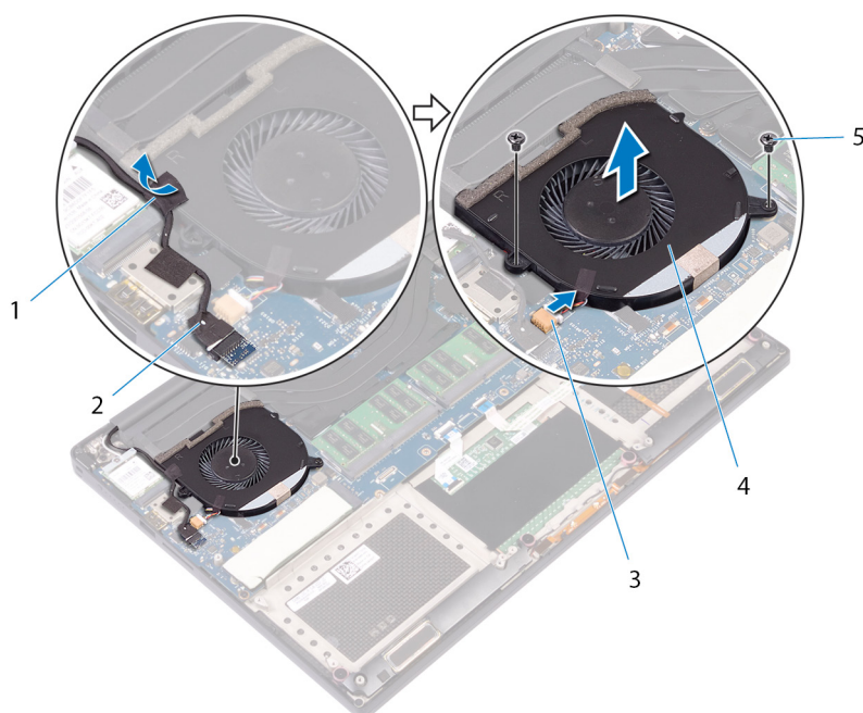
Figura 18. Como remover o ventilador direito
