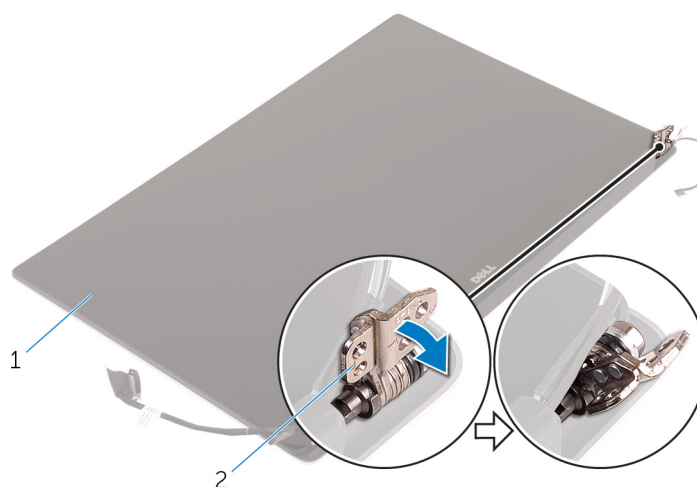
Figura 33. Como girar a dobradiça da tela
