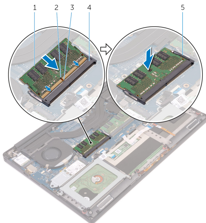
Figura 6. Imagem: como substituir os módulos de memória
