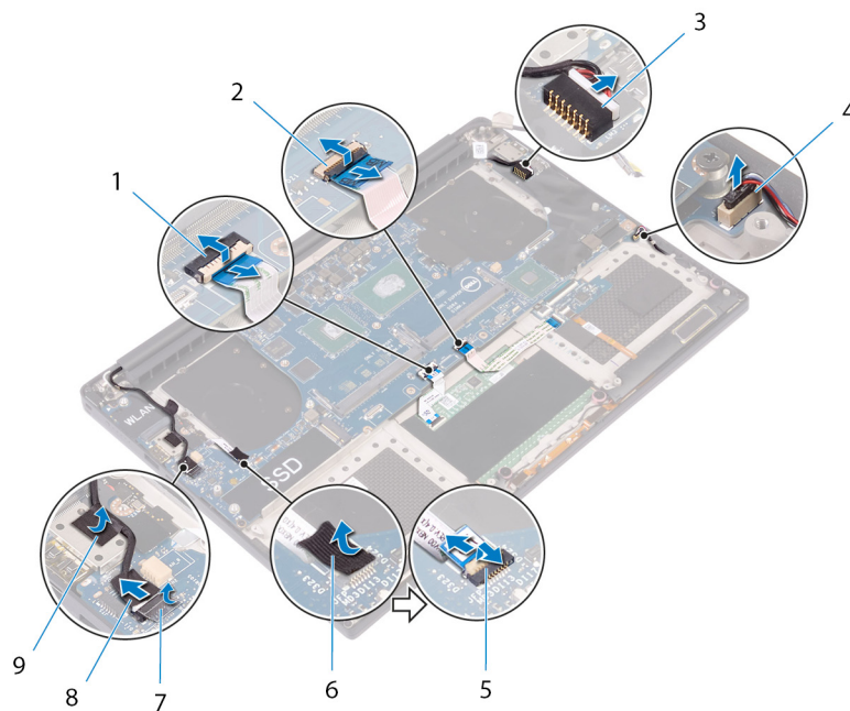
Figura 22. Como desconectar os cabos
