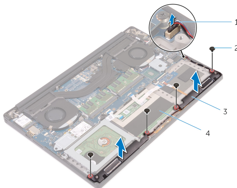
Figura 13. Rimozione degli altoparlanti
