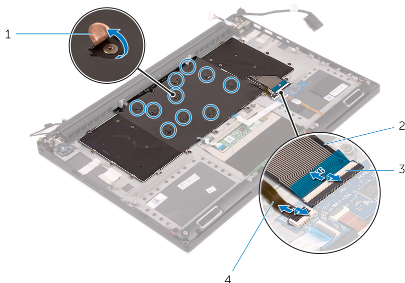
Figura 26. Scollegamento del cavo della tastiera e del cavo di retroilluminazione della tastiera.
