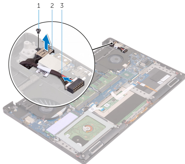
Figura 31. Rimozione della porta dell'adattatore di alimentazione
