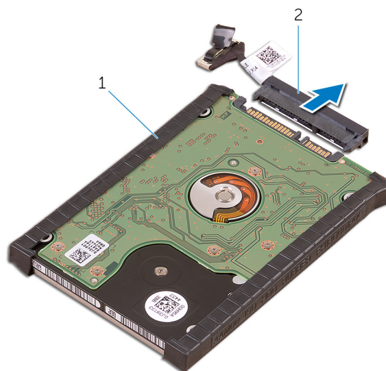
Figura 7. Scollegamento dell'interposer del disco rigido dal gruppo disco rigido
