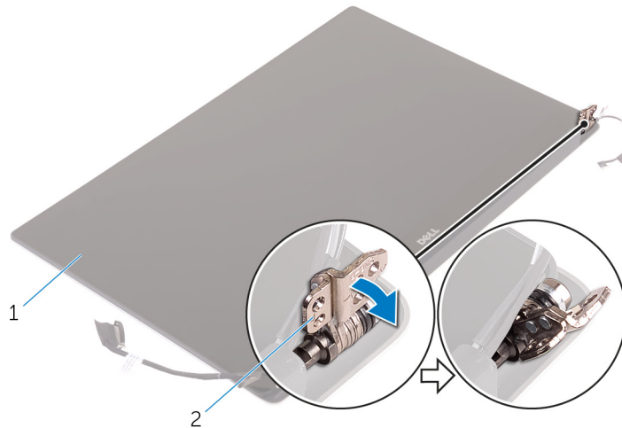
Figura 32. Capovolgimento dei cardini dello schermo
