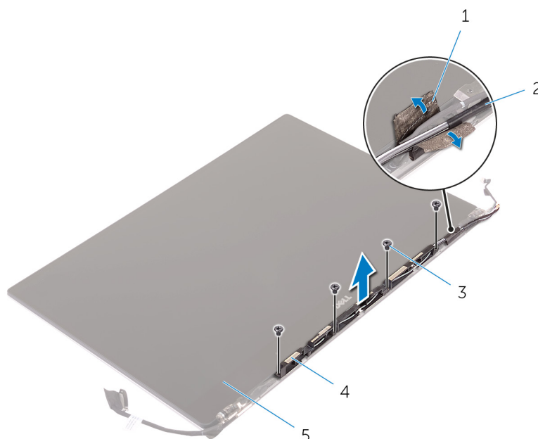
Figura 36. Rimozione del modulo dell'antenna
