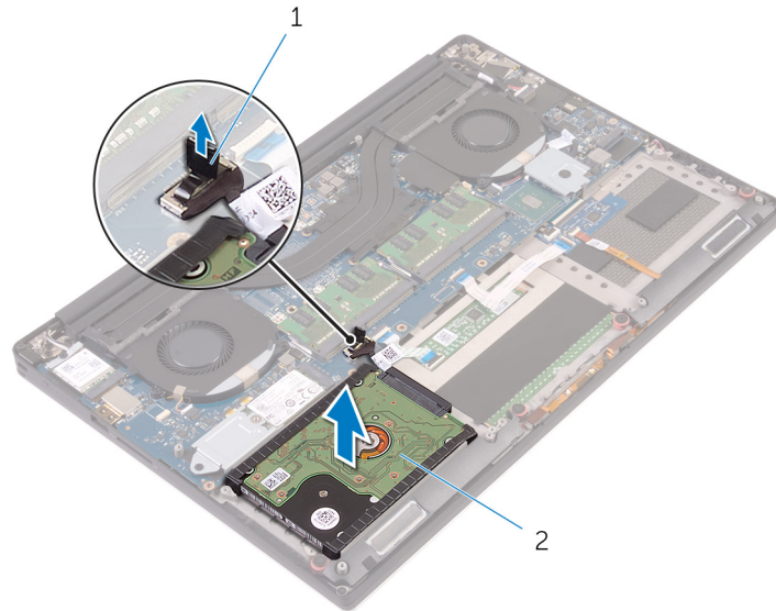
Figura 6. Scollegamento del cavo del disco rigido dalla scheda di sistema
