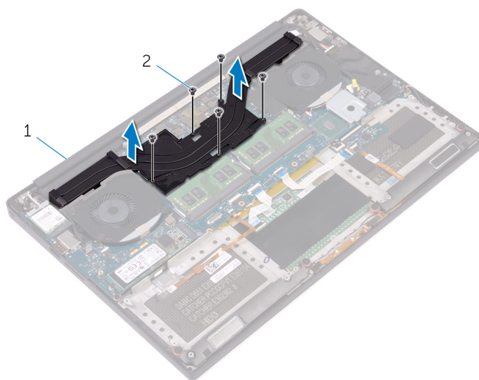
Figura 18. Rimozione del gruppo dissipatore di calore
