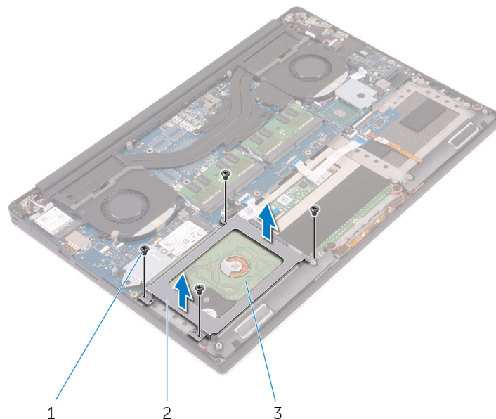
Figura 5. Rimozione della gabbia del disco rigido
