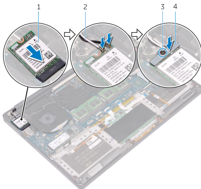
Figura 15. Ricollocamento della scheda per reti senza fili.
