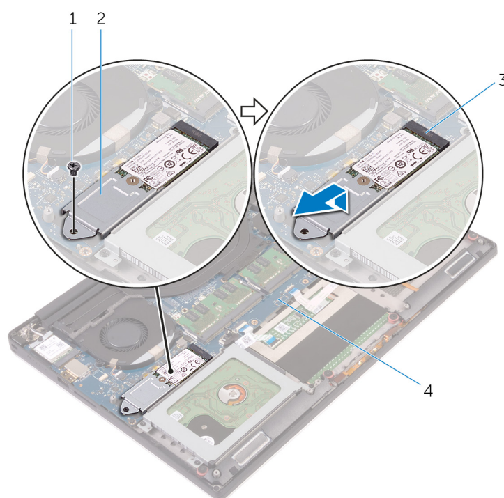
Figura 9. Rimozione del gruppo dell'unità a stato solido
