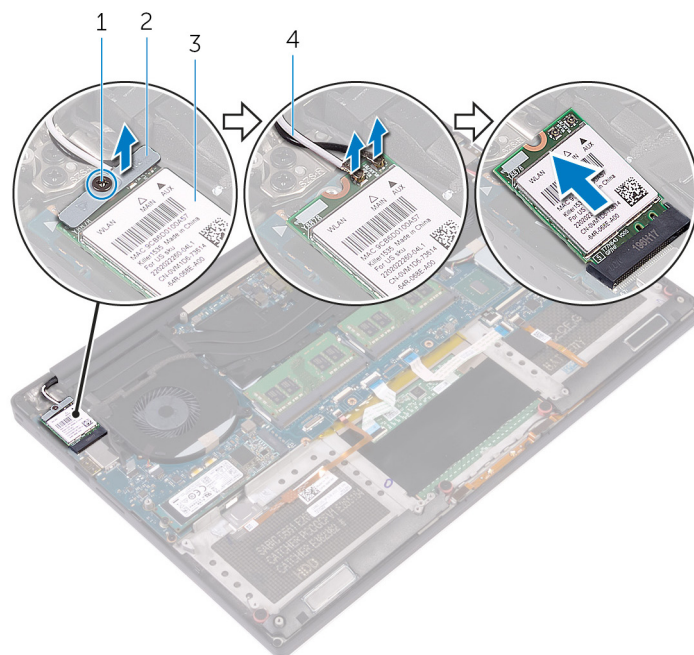
Figura 14. Rimozione della scheda per reti senza fili
