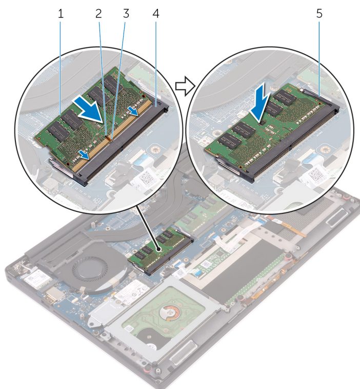
Figura 20. Ricollocamento dei moduli di memoria
