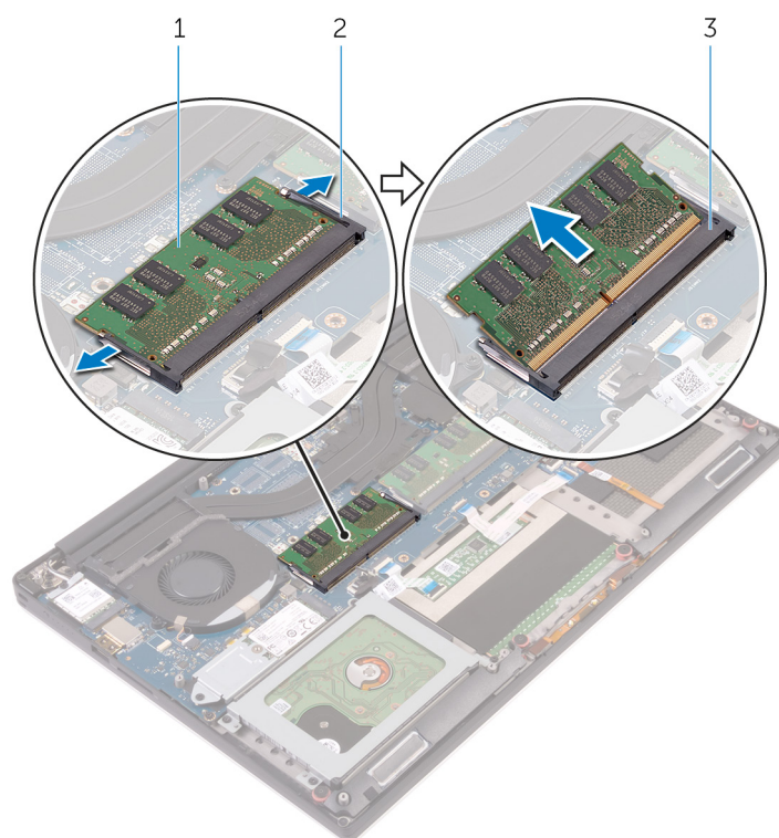
Figura 19. Rimozione dei moduli di memoria
