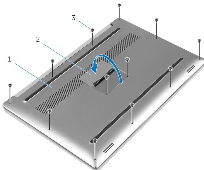
Rysunek 1. Wymontowywanie pokrywy dolnej
