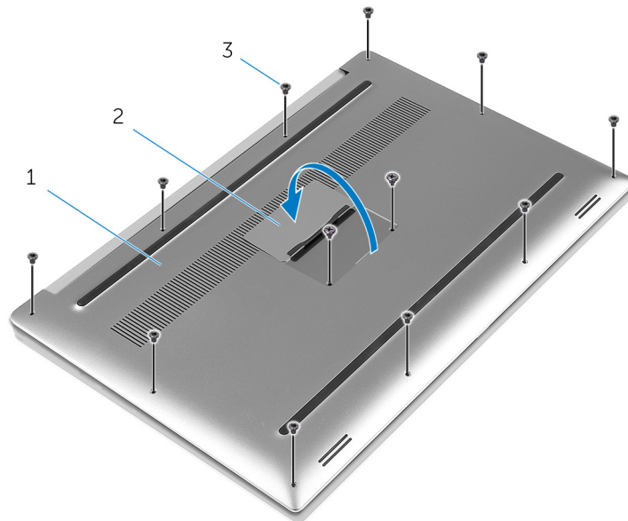
Figura 1. Rimozione del coperchio della base
