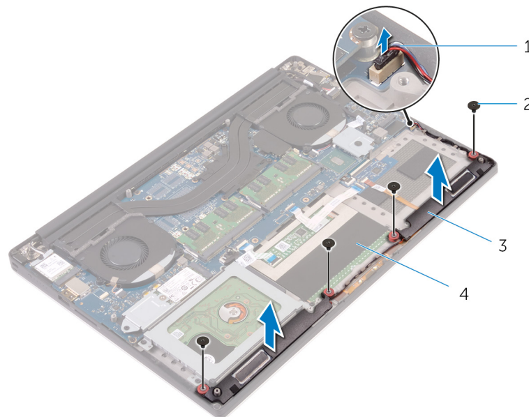
Figura 15. Rimozione degli altoparlanti
