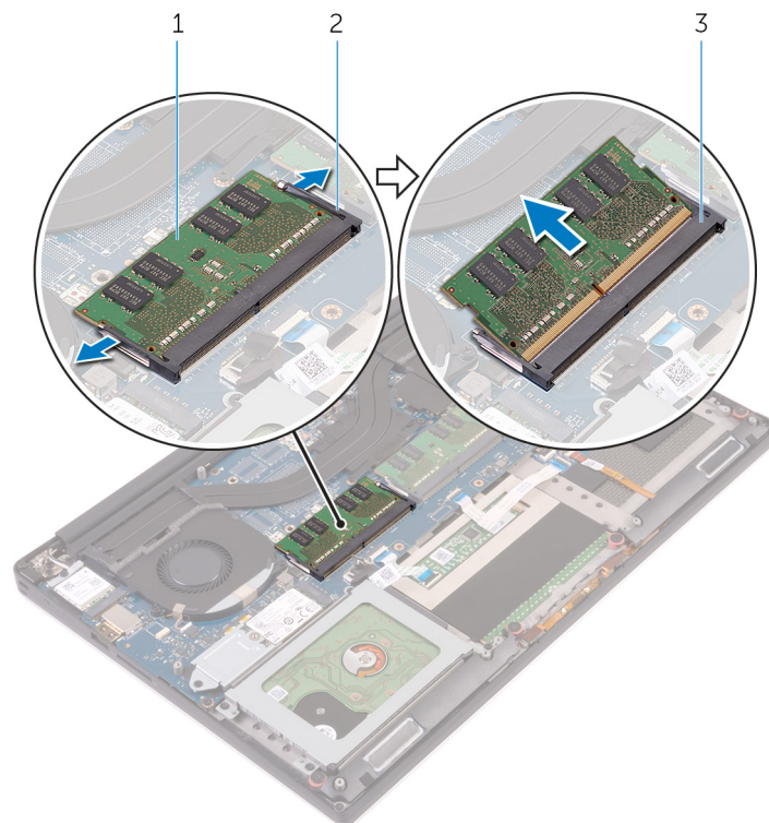
Figura 5. Rimozione dei moduli di memoria
