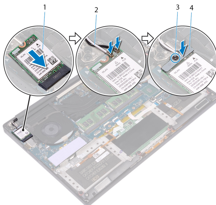
Figura 17. Ricollocamento della scheda per reti senza fili.
