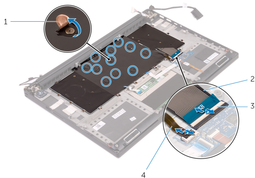
איור 27. ניתוק של כבל המקלדת וכבל התאורה האחורית של המקלדת
