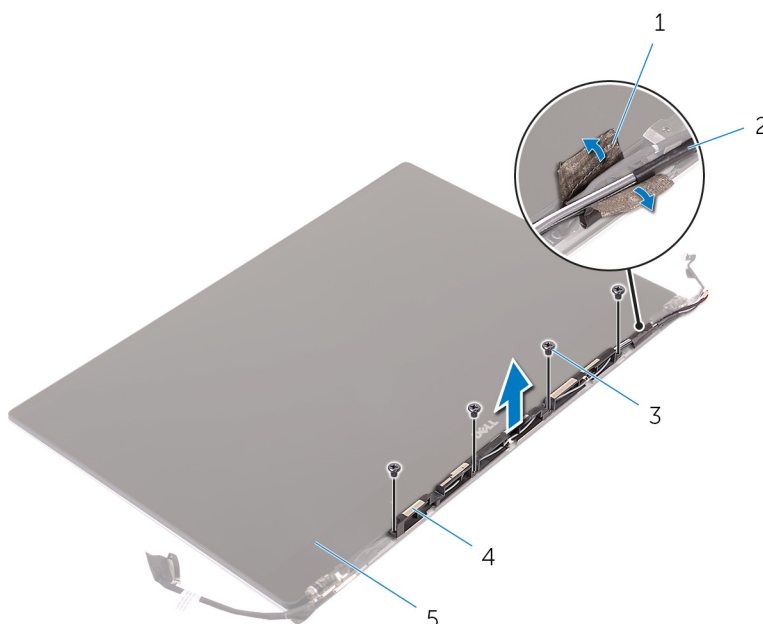
Figure 35. Retrait du module d'antenne
