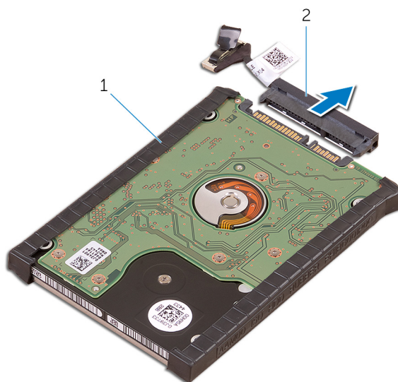
Figure 9. Déconnexion de l'assemblage du disque dur de son interposeur
