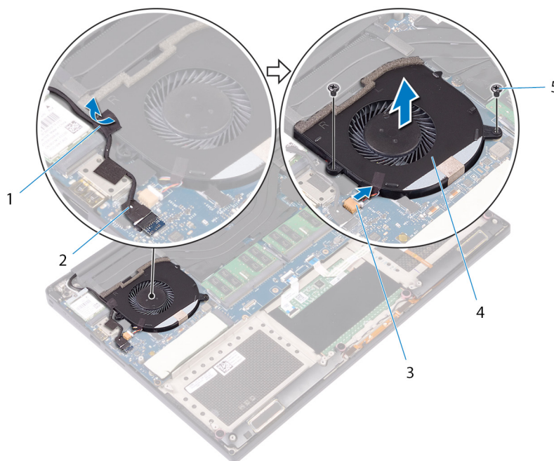
Figure 18. Retrait du ventilateur de droite
