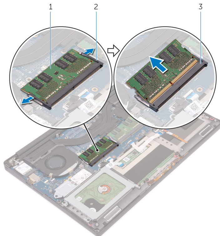
Figure 5. Retrait les modules de mémoire
