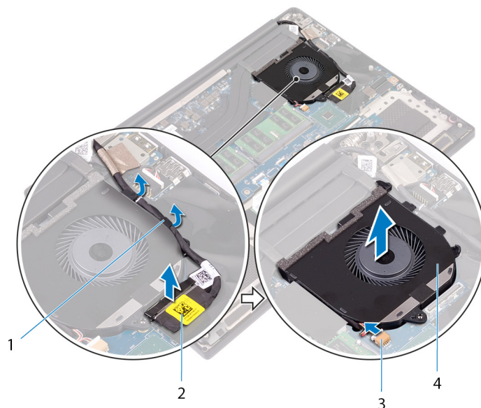
Figure 20. Retrait du ventilateur de gauche
