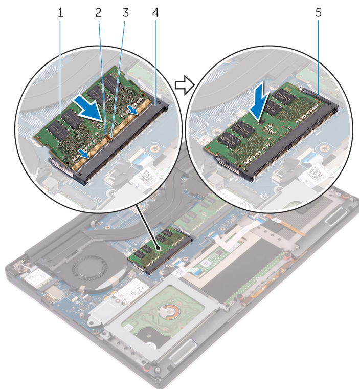
Figure 6. Remise en place des modules de mémoire
