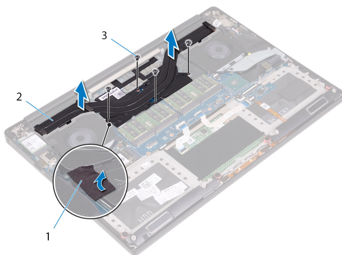
Figure 21. Retrait du dissipateur de chaleur
