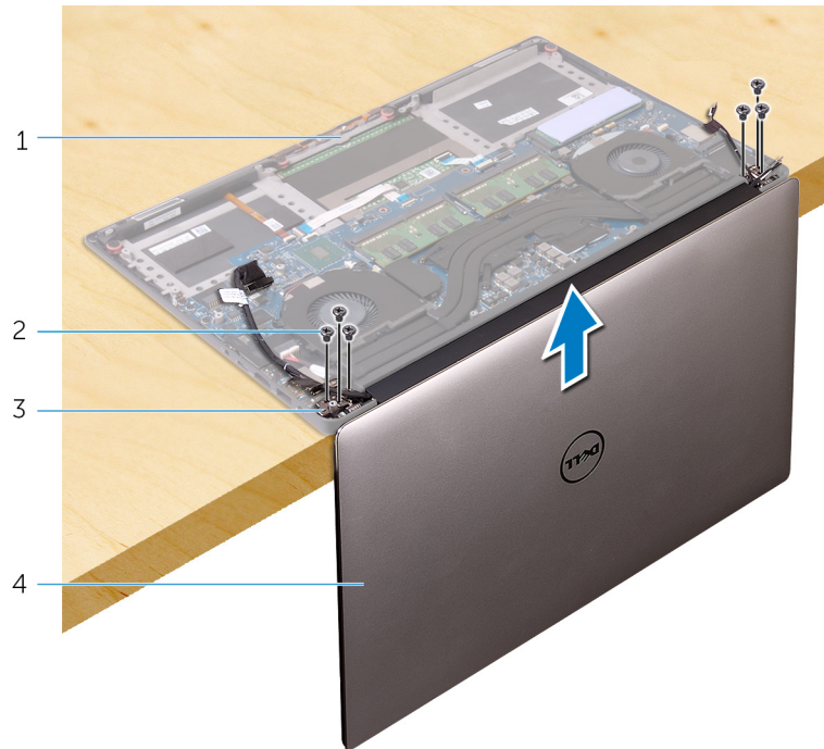
Figure 30. Retirez les vis qui fixent les charnières de l'écran à l'assemblage du repose-mains
