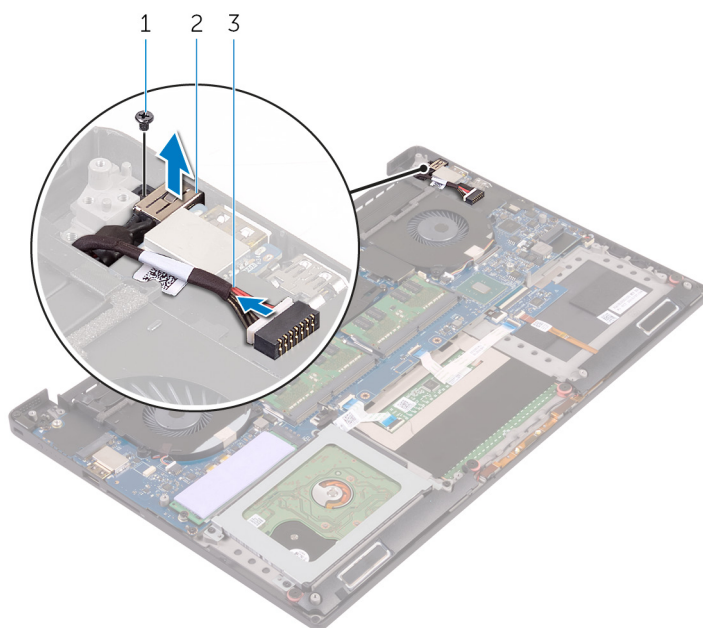
Figure 32. Retrait du port d'adaptateur d'alimentation
