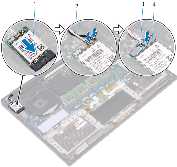
Figure 17. Remise en place de la carte sans fil
