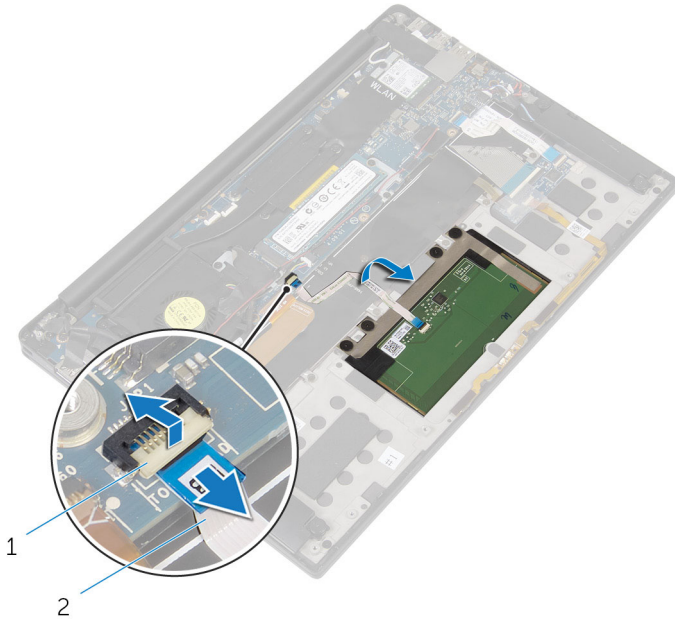
그림 13. 터치패드 케이블 분리
