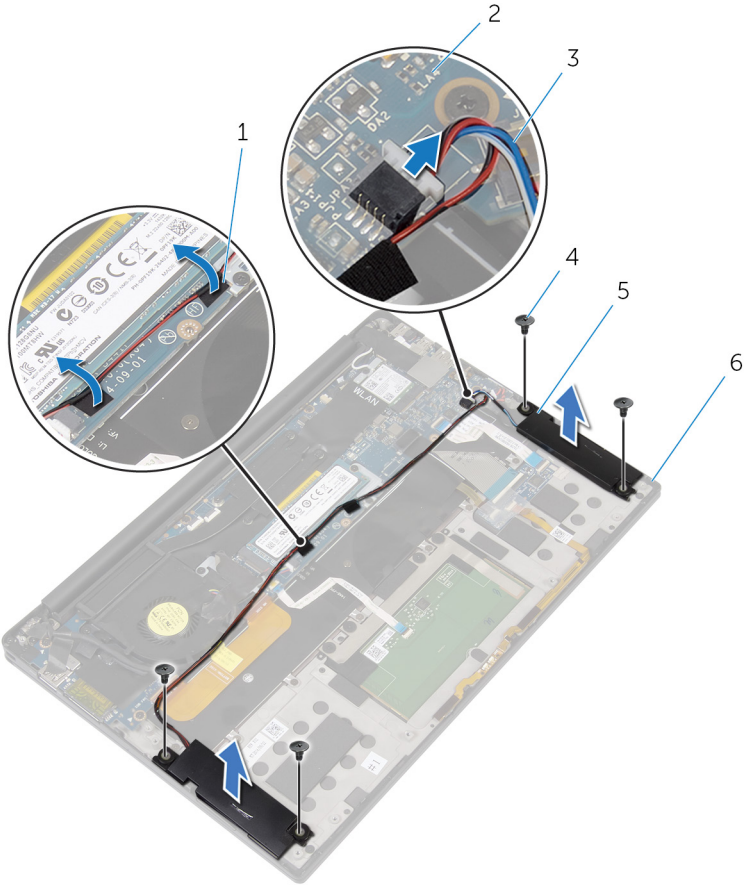
그림 9 . 스피커 분리
