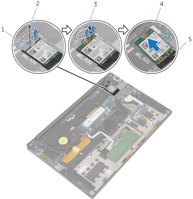
그림 7. 무선 카드 분리
