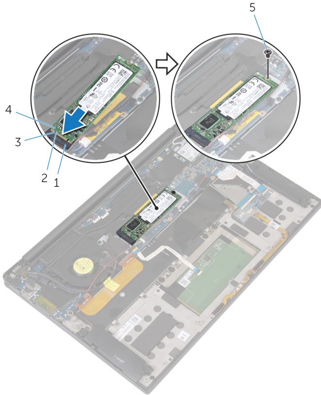
그림 6. 솔리드 상태 드라이브 장착
