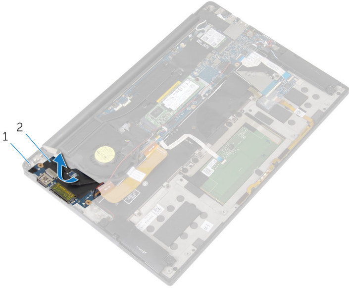
그림 17 . I/O 보드 분리
