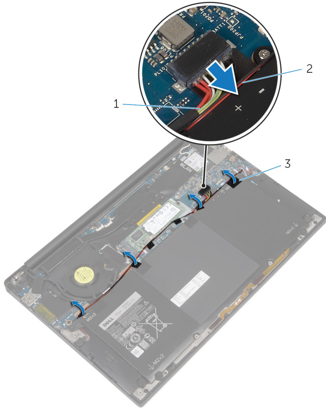
그림 3. 배터리 분리
