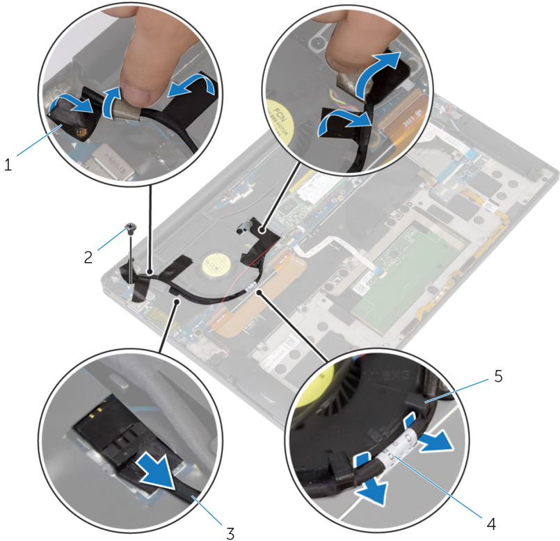
그림 19 . 디스플레이 조립품 분리
