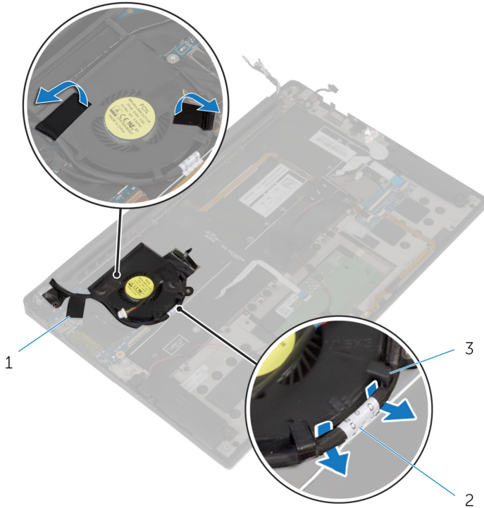
그림 30 . 팬 분리
