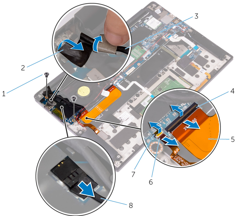
그림 16 . I/O 보드 분리
