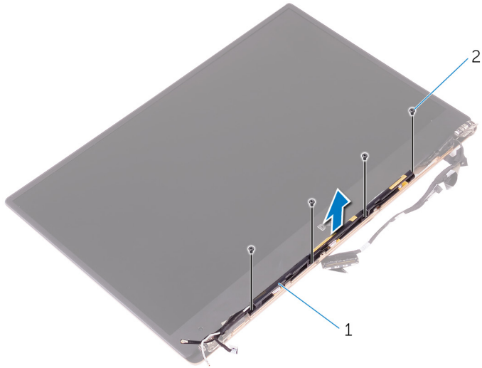
그림 24. 안테나 분리
