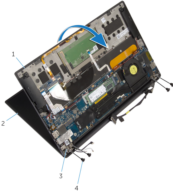
그림 21. 디스플레이 조립품 분리
