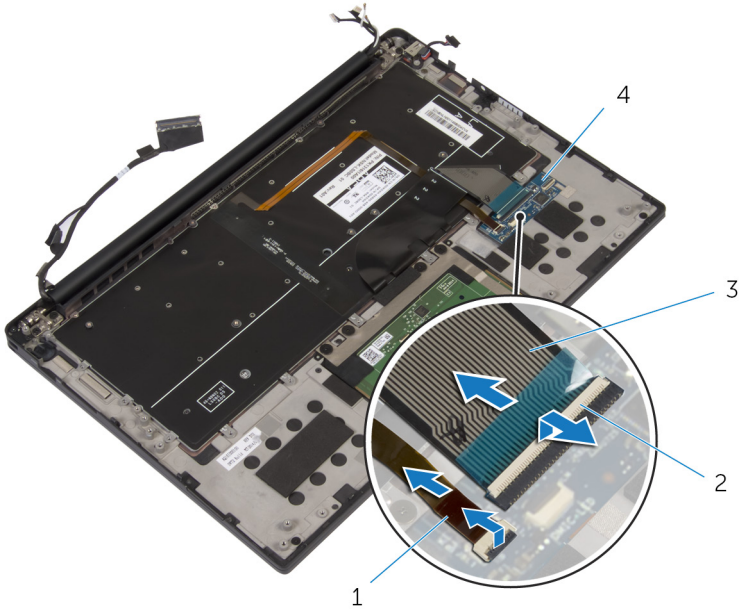
그림 32. 키보드 분리
