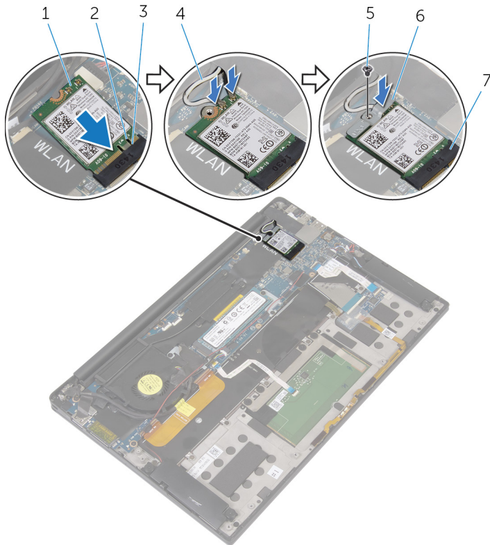
그림 8. 무선 카드 장착
