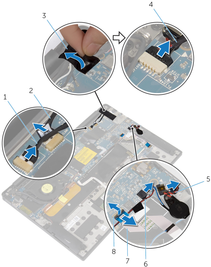
그림 25 . 시스템 보드 제거
