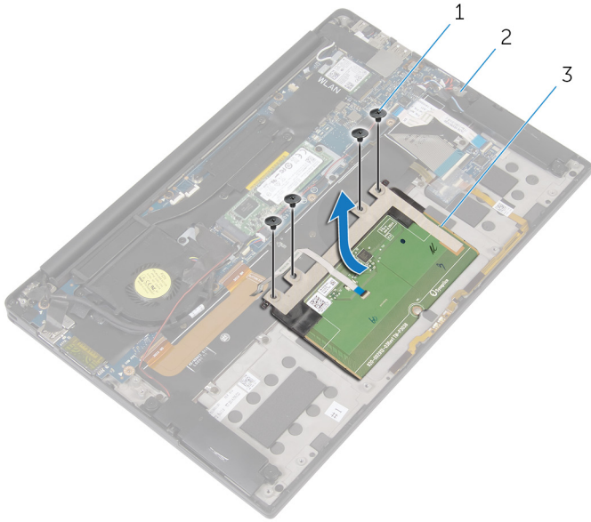
그림 14 . 터치패드 분리
