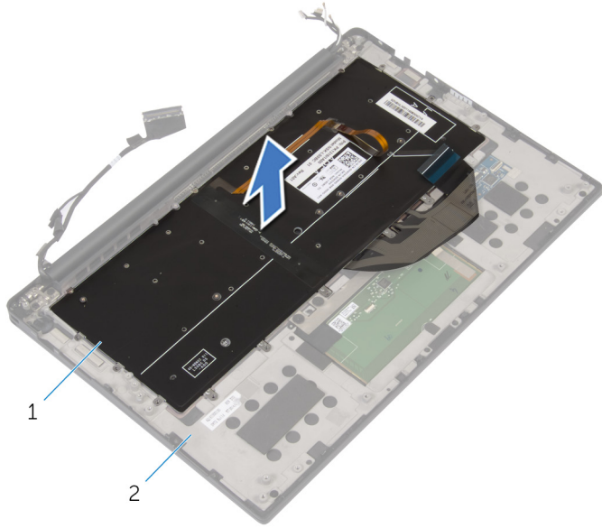
그림 34. 키보드 분리
