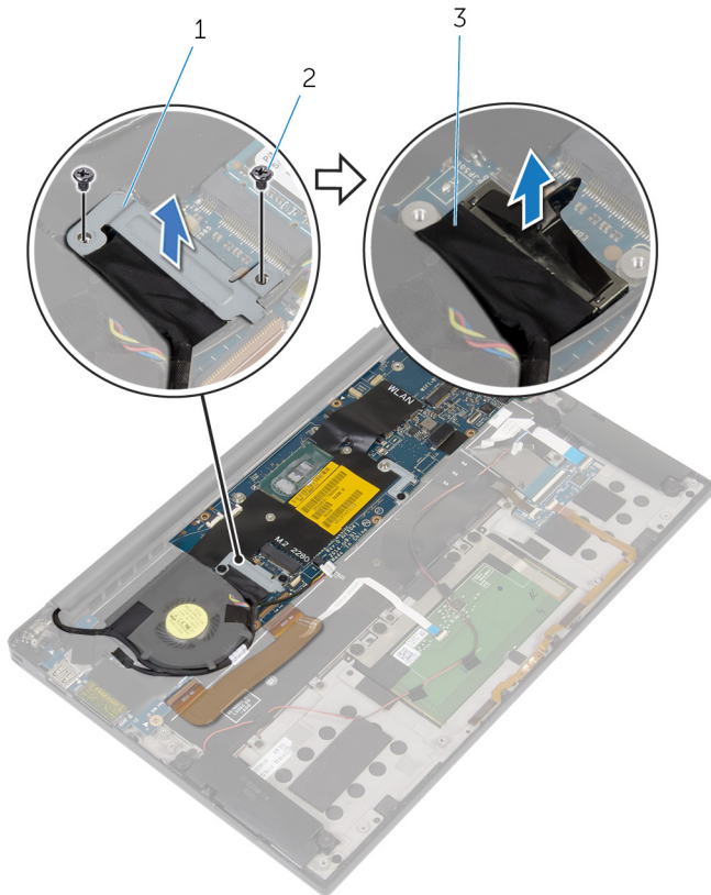
그림 27. 시스템 보드 제거
