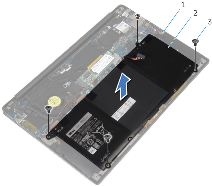
그림 4. 배터리 분리
