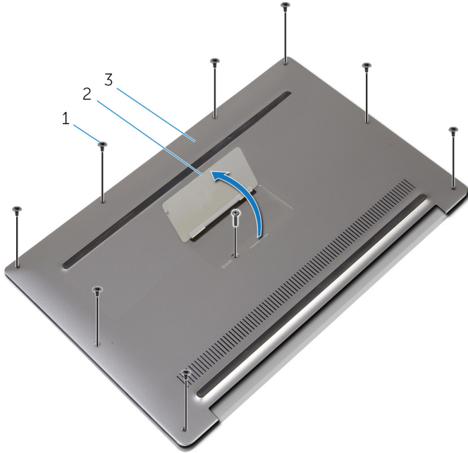
그림 1. 베이스 덮개 분리
