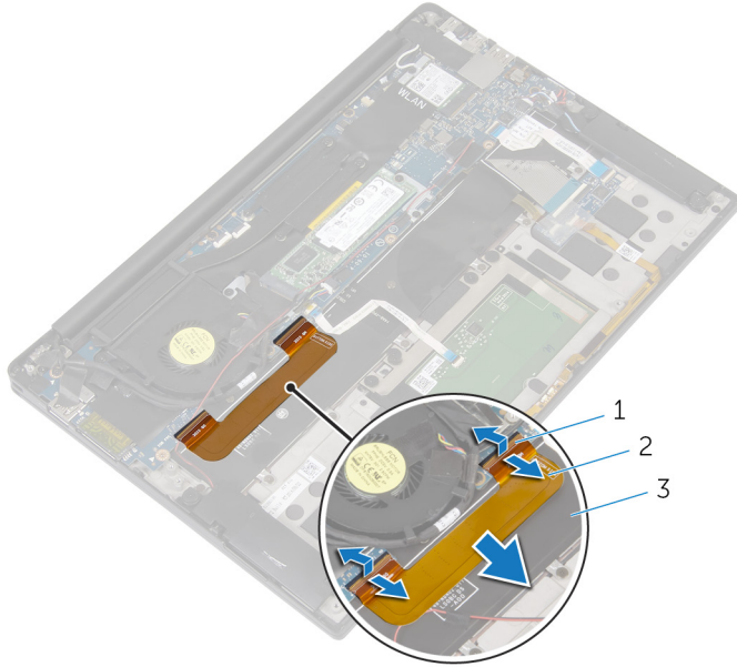
그림 15 . I/O 보드 케이블 분리
