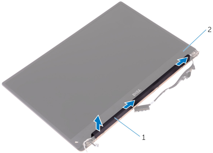
그림 23. 디스플레이 힌지 덮개 분리
