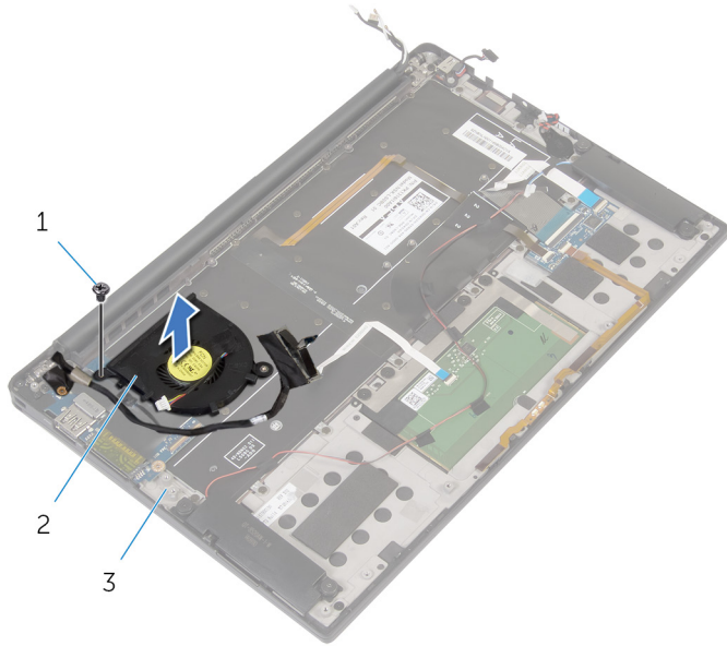
그림 31. 팬 분리
