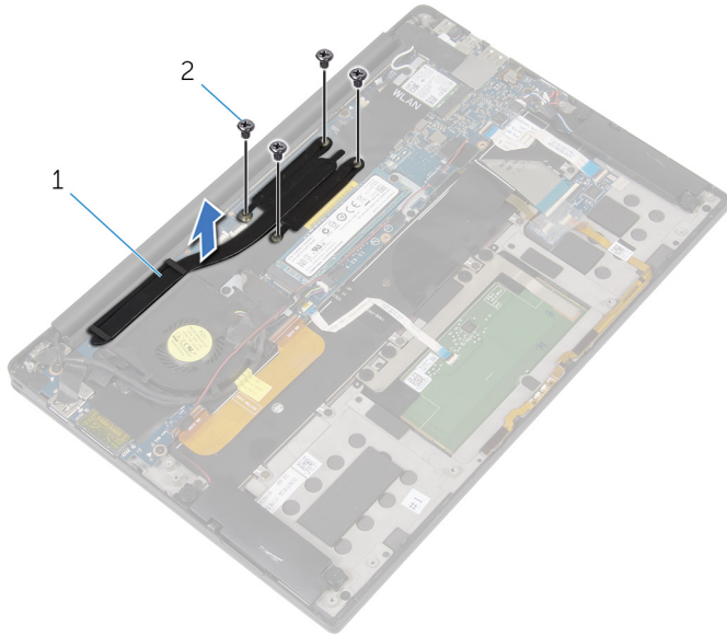
그림 11. 방열판 분리
