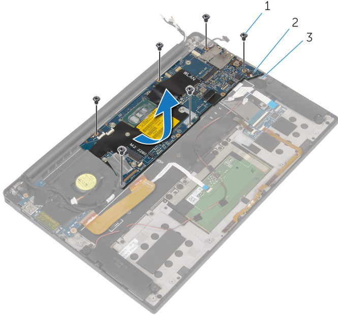
그림 28. 시스템 보드 제거
