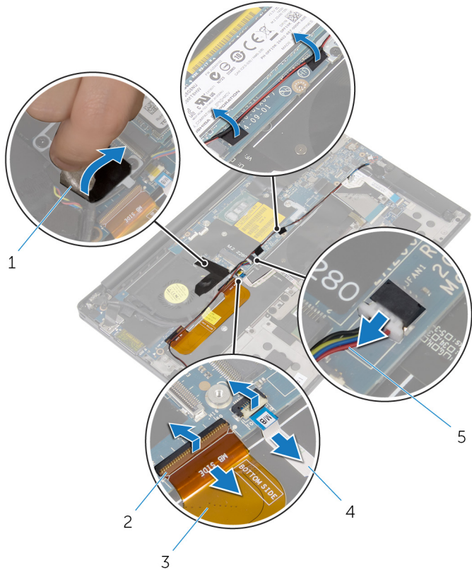
그림 26 . 시스템 보드 제거
