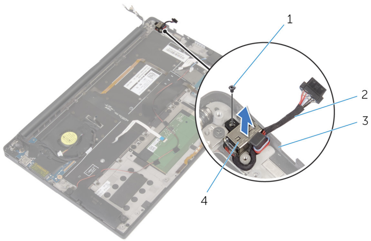
그림 29. 전원 어댑터 포트 분리
