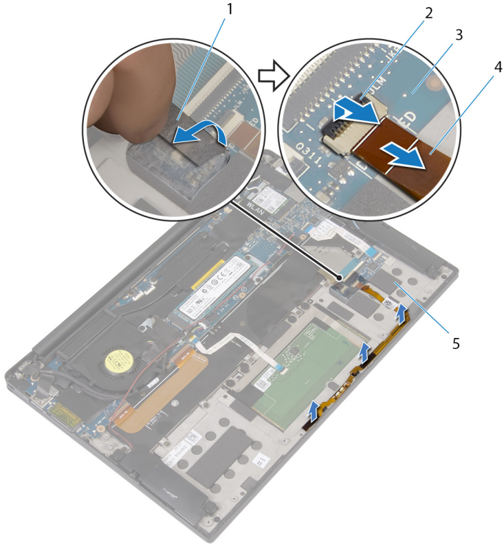
그림 12. 배터리 상태 표시등 케이블(마이크 포함) 제거
