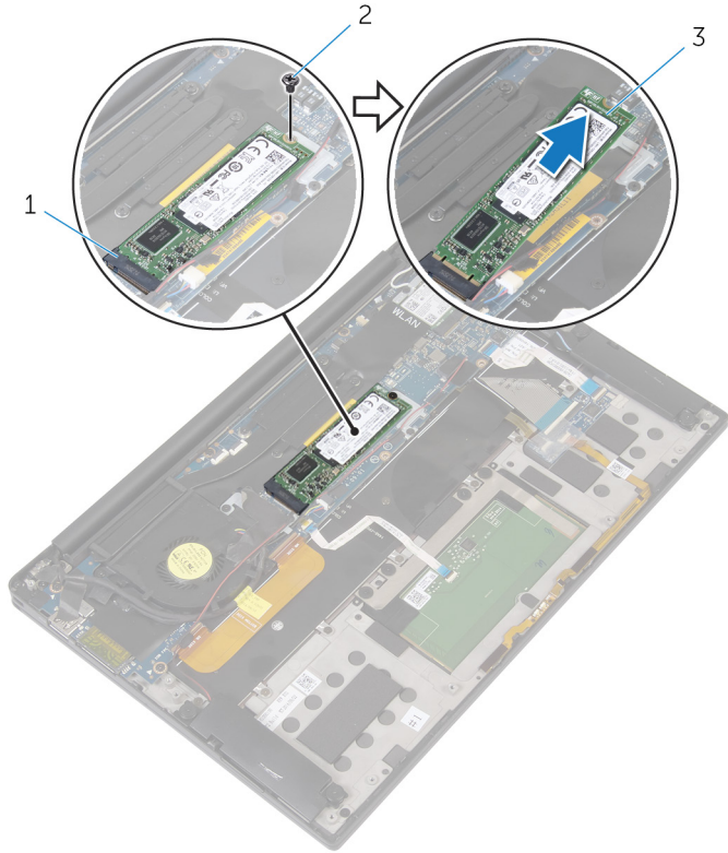
그림 5. 솔리드 상태 드라이브 분리
