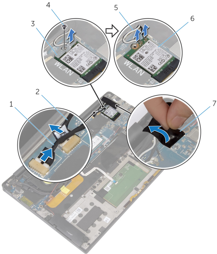
그림 18. 디스플레이 조립품 분리
