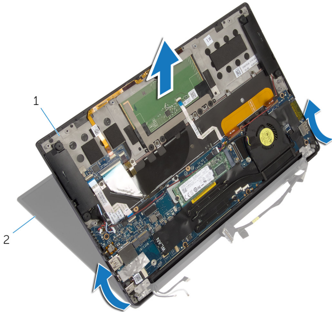
그림 22. 디스플레이 조립품 분리
