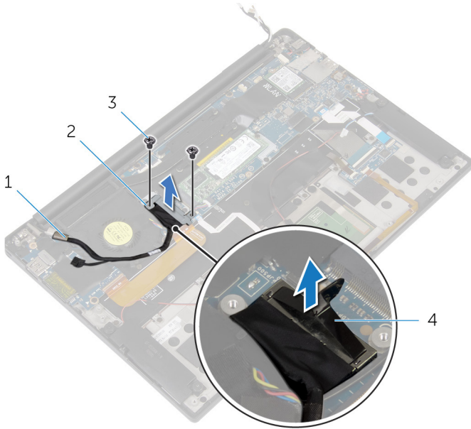
그림 20 . 디스플레이 조립품 분리
