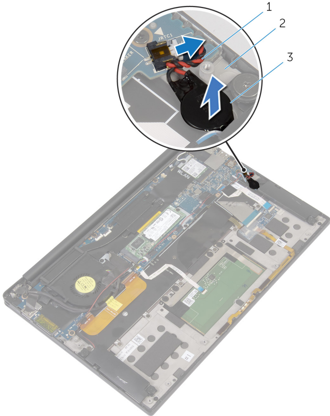
그림 10. 코인 셀 배터리 분리
