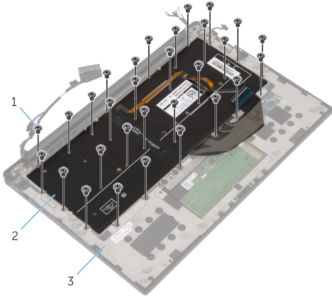
그림 33. 키보드 분리
