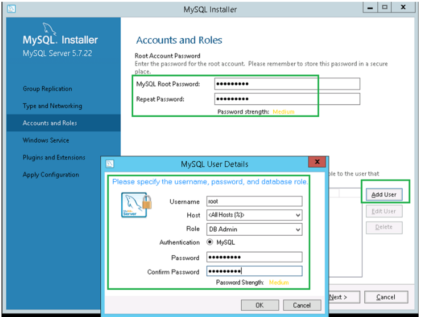
图 29: 添加用户
