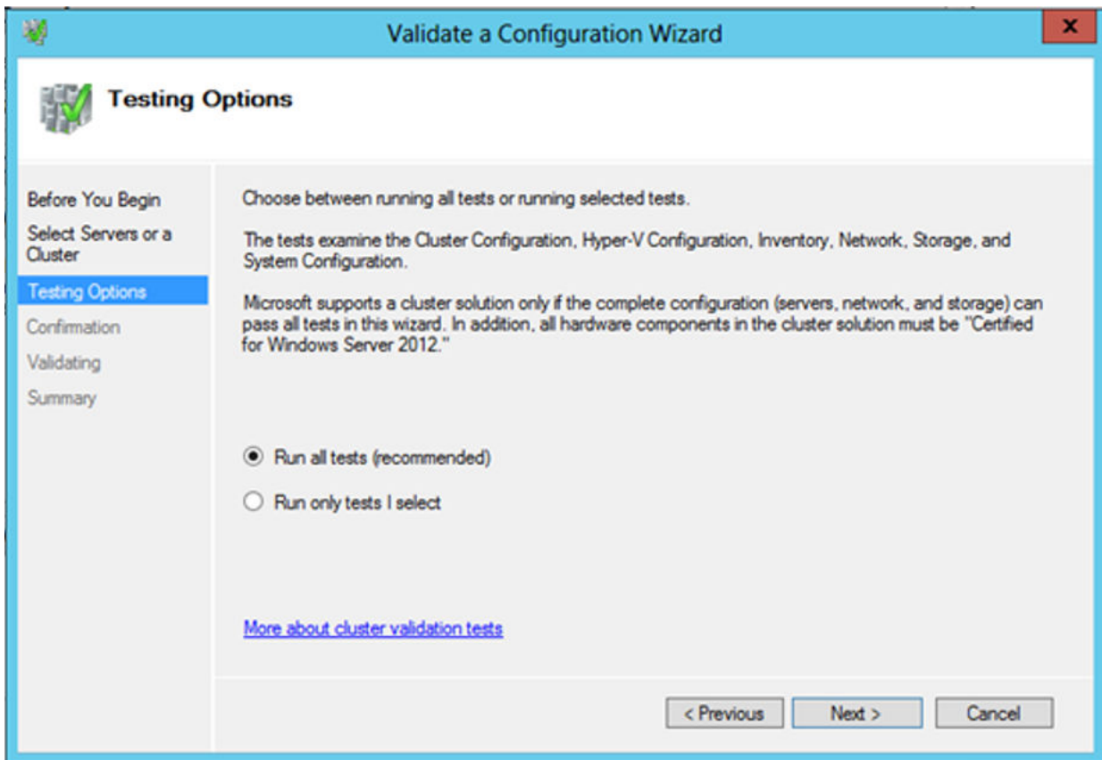
图 9: 测试选项
