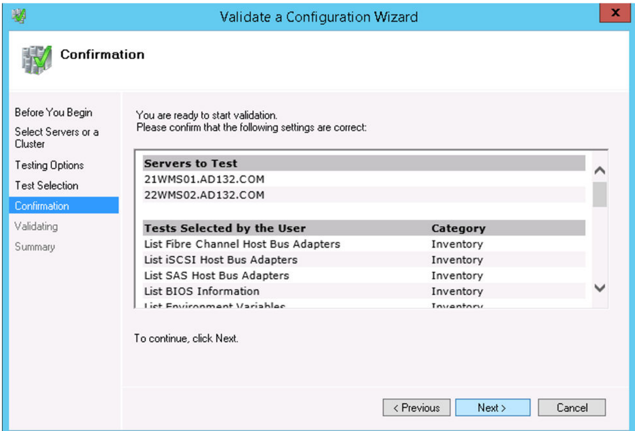
图 10: 确认
