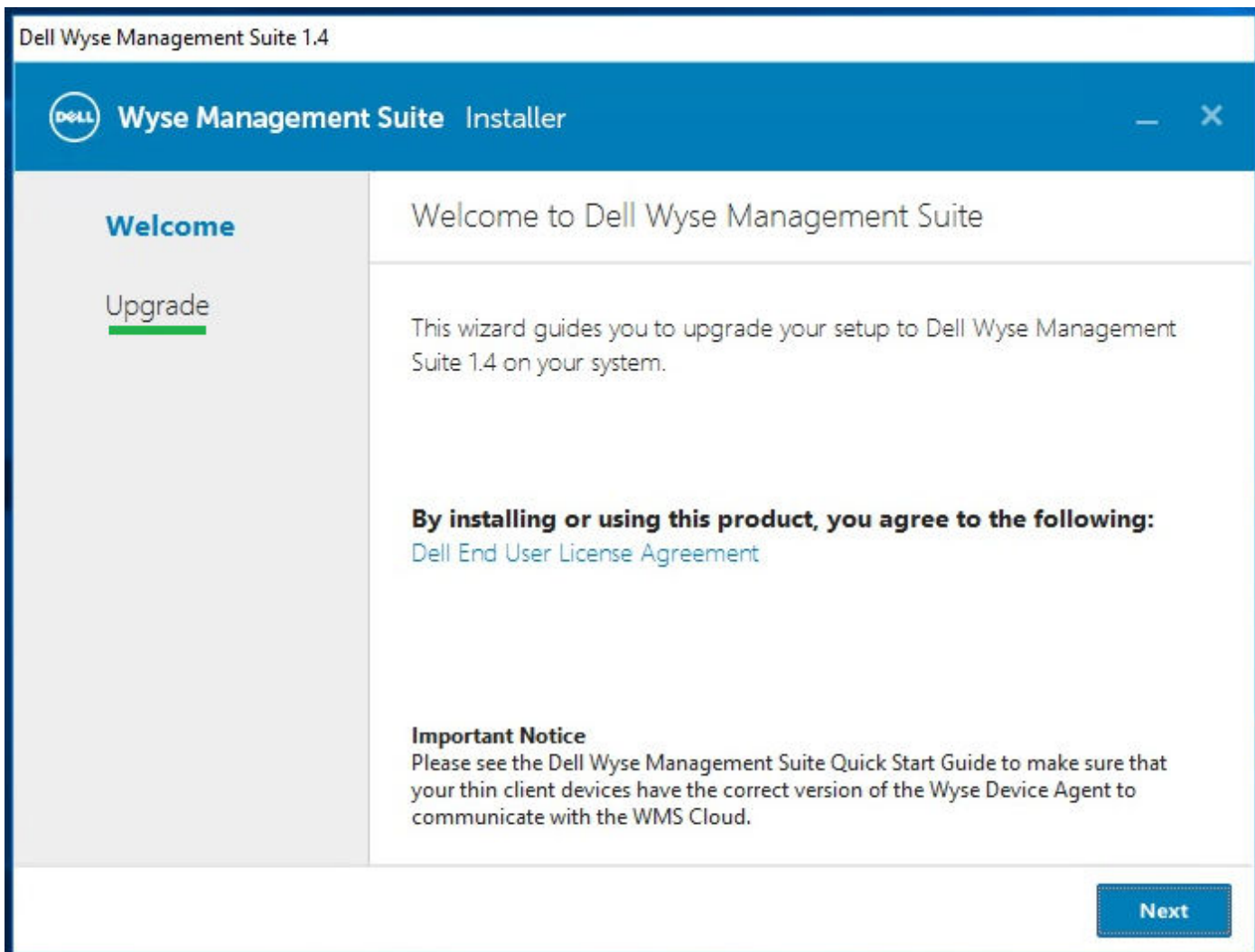
图 75: 欢迎屏幕
