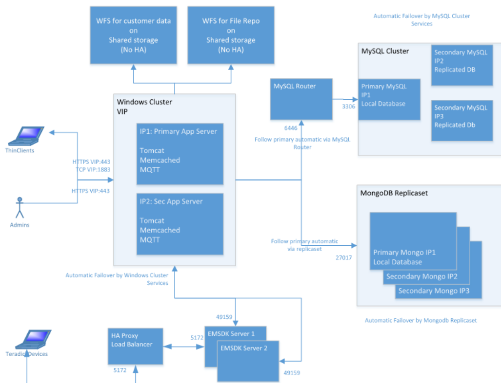
Ilustración 1. Arquitectura de alta disponibilidad
