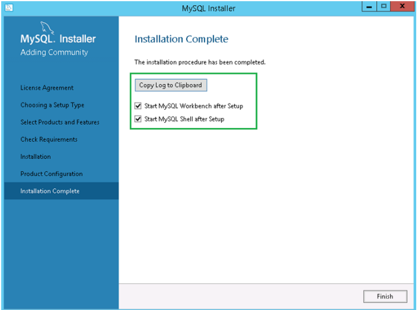
그림 36 . 설치 완료
