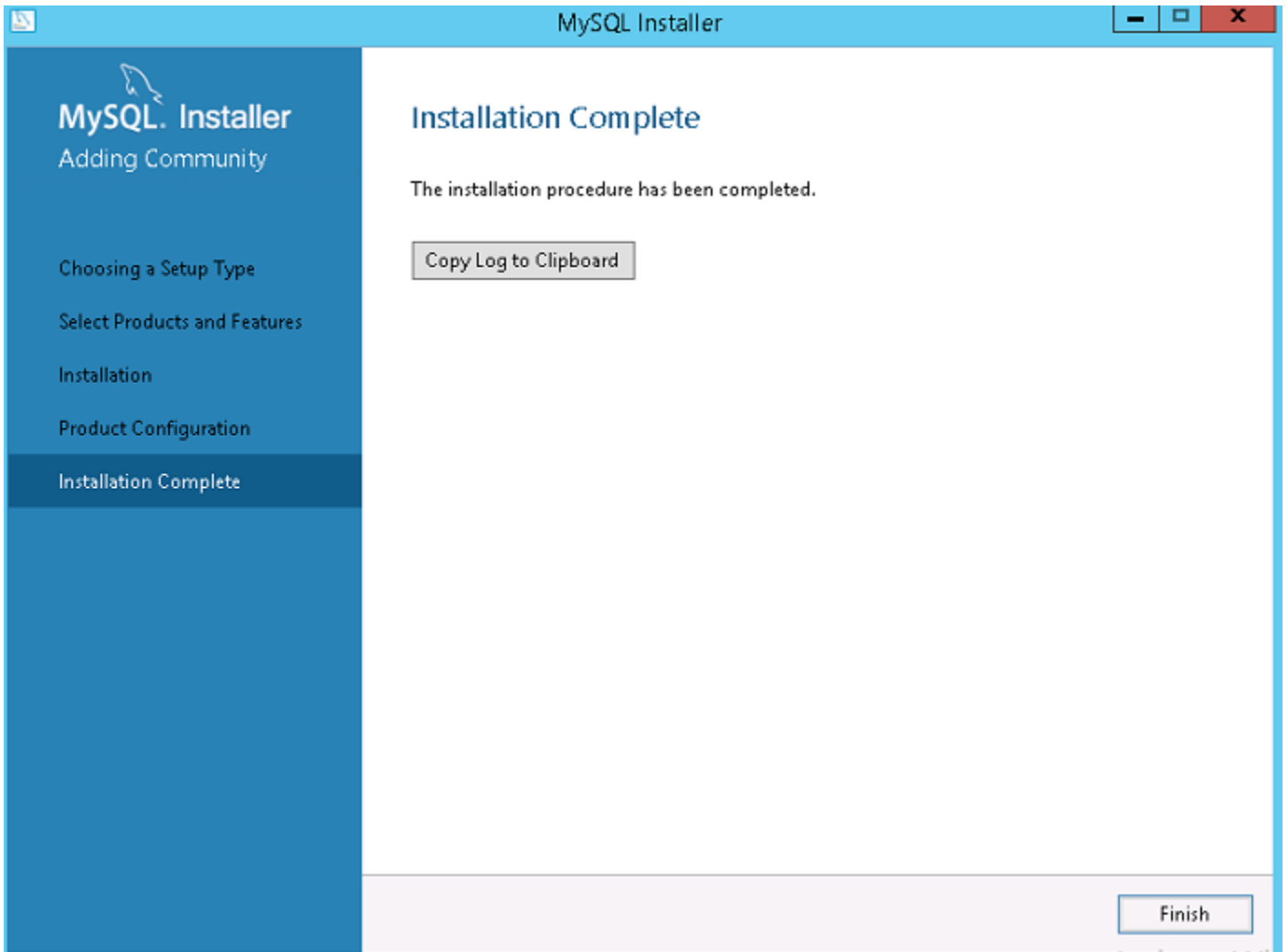
그림 52 . 설치 완료
