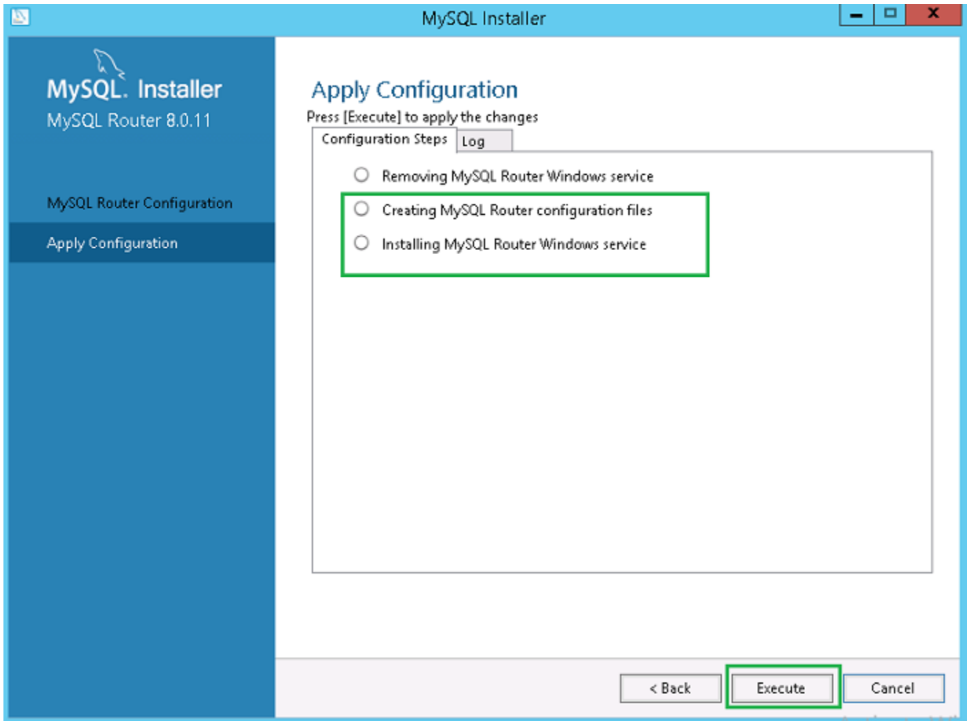
그림 49 . 구성 적용
