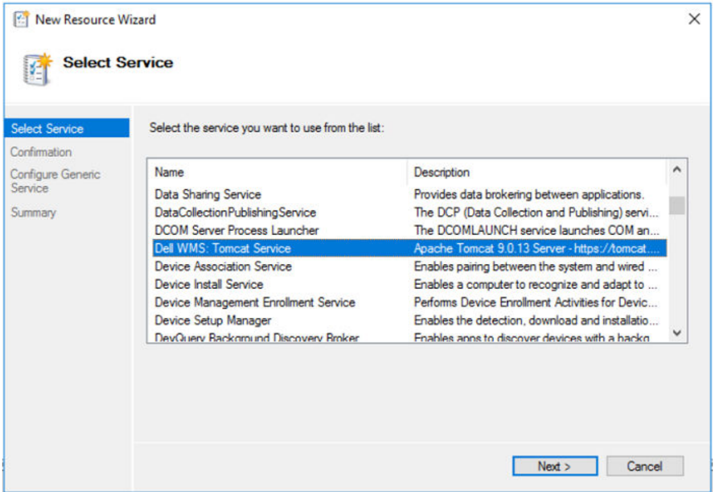
그림 4. 서비스 선택
