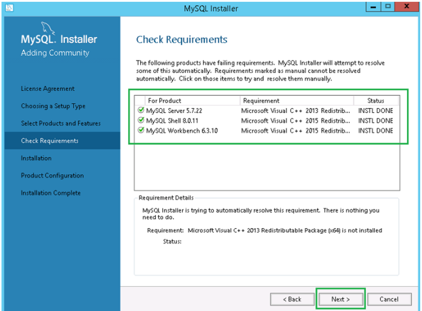
그림 23 . 요구 사항
