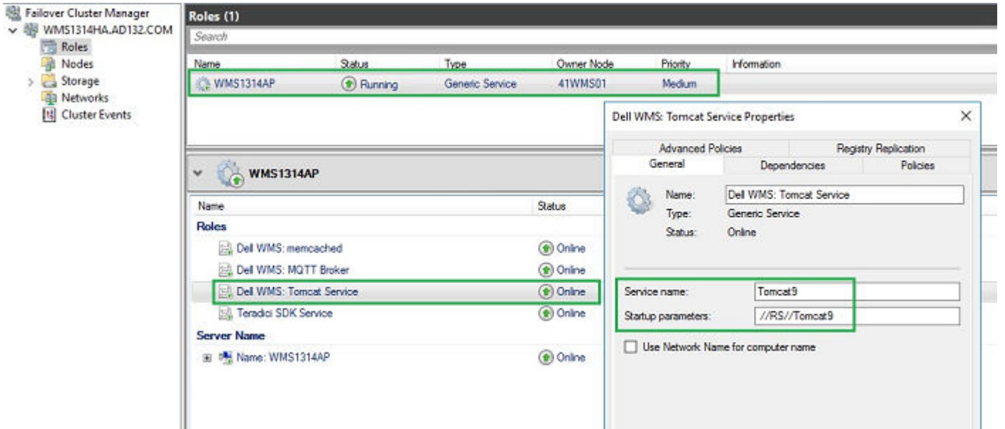
그림 70 . Tomcat 9 서비스
