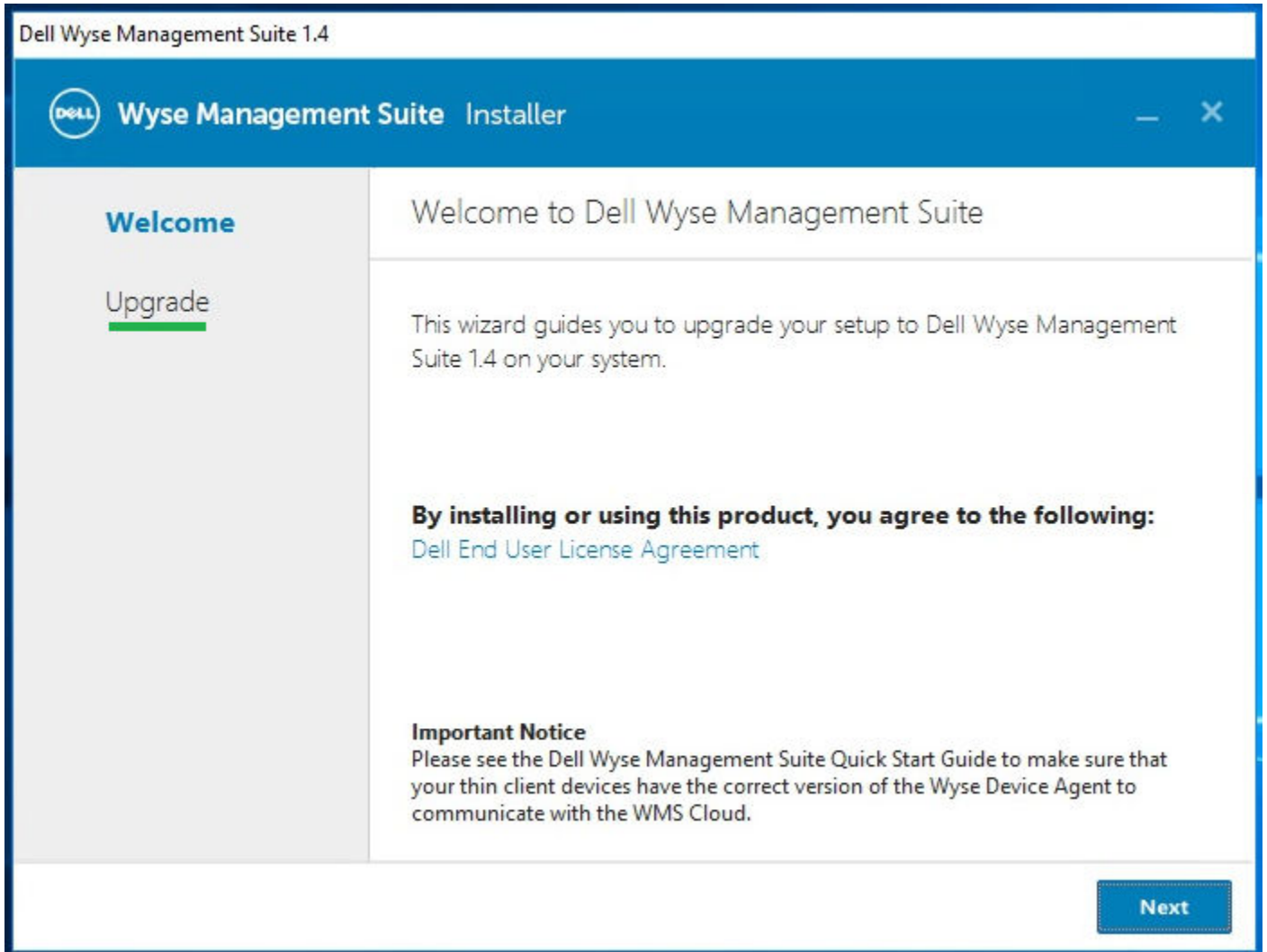
그림 63 . Welcome 화면
