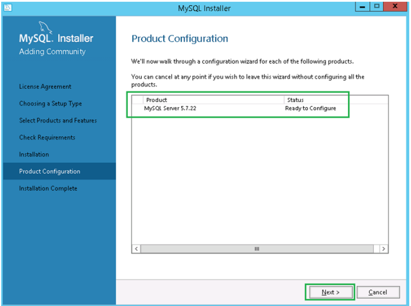
그림 26 . 제품 구성
