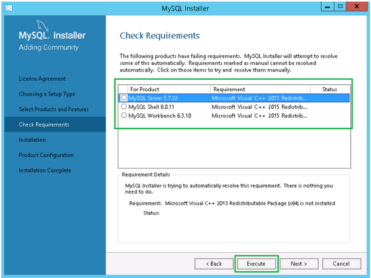
그림 21. 요구 사항
