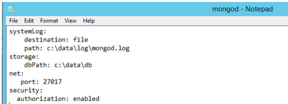
그림 56 . mongod.cfg 편집
