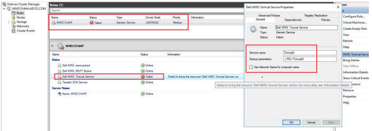
Figure 67. Point d'accès
