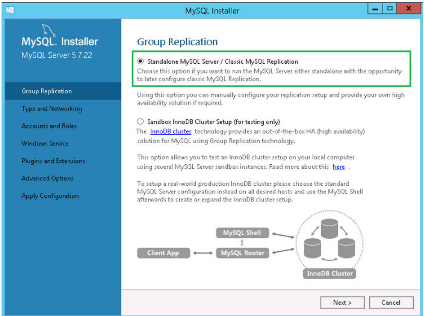
Figura 27. Replicación de grupos
