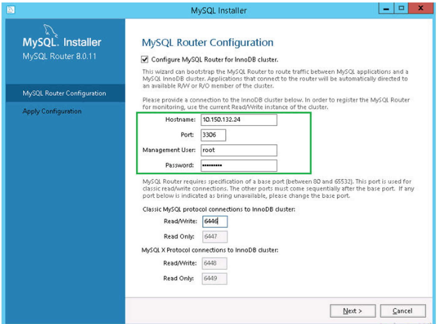
Figura 48. Configuración del enrutador de MySQL
