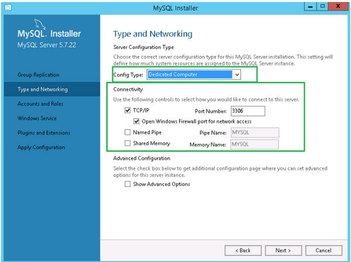
Figura 28. Tipo y redes
