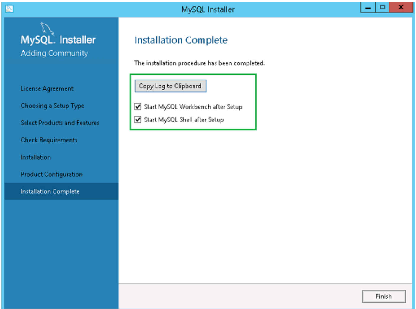
Figura 36. Instalación completa
