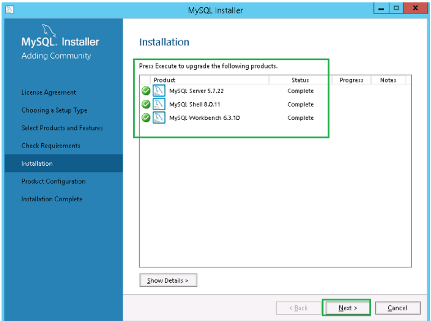
Figura 25. Instalación
