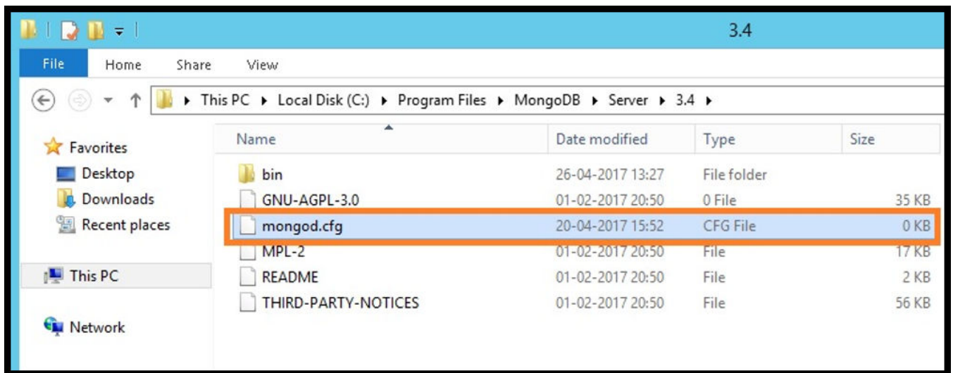
Figura 55. Archivo mongod.cfg
