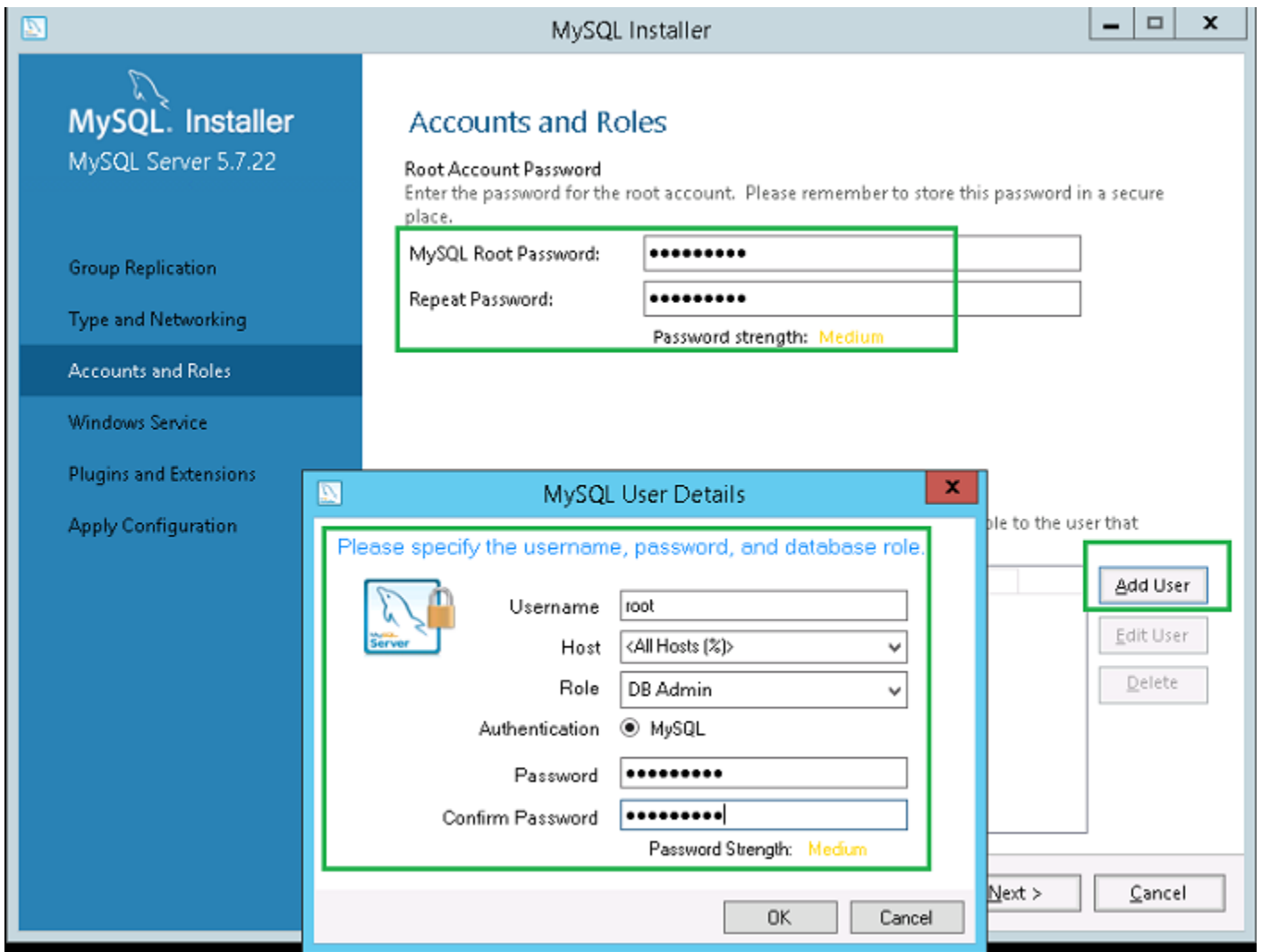
Figura 29. Agregar usuario
