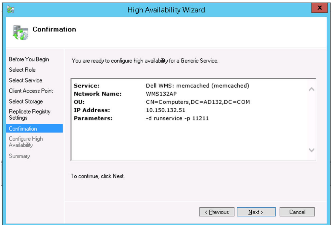
Figura 5. Confirmación
