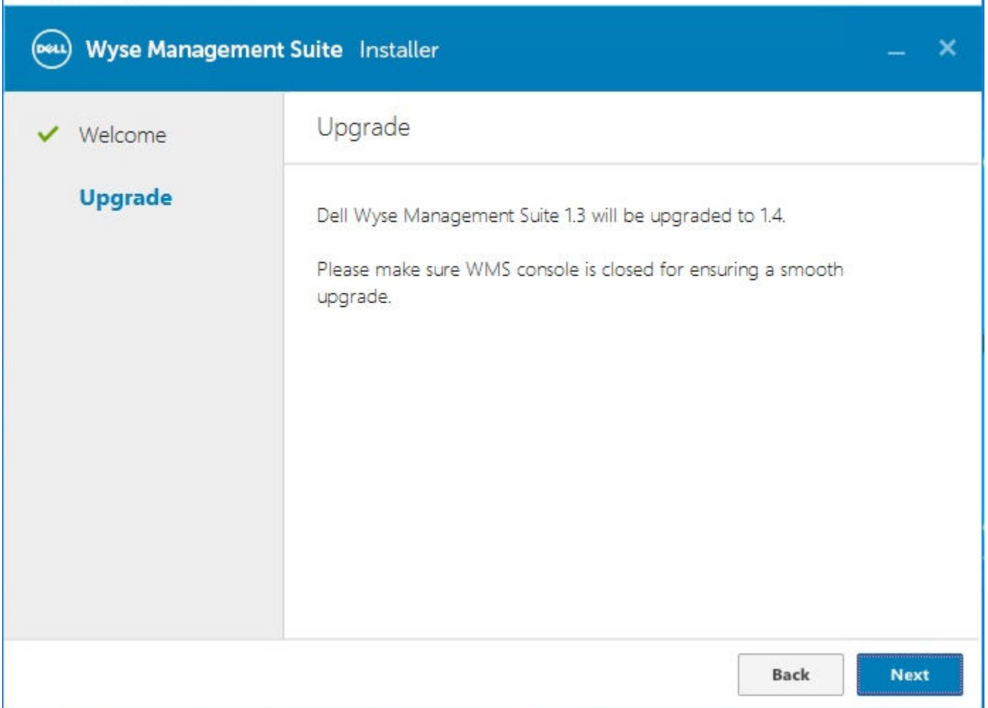
Figura 64. Actualización
