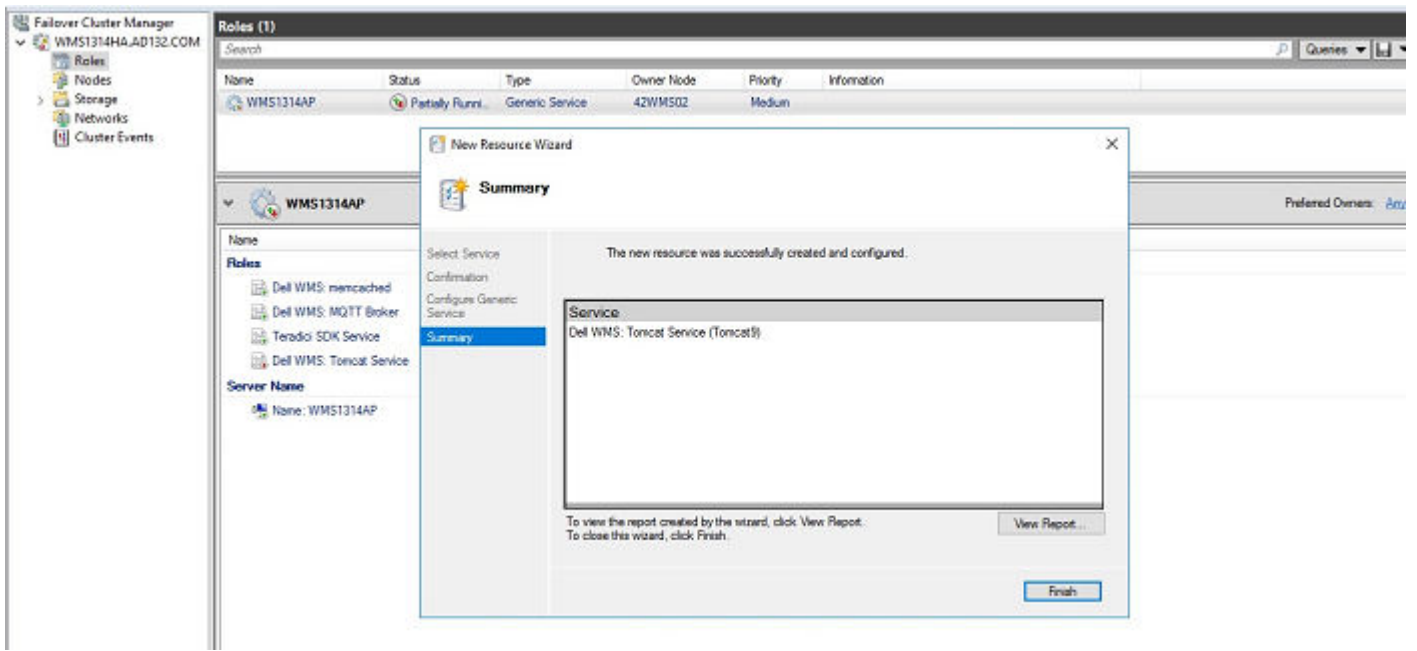
Figura 69. Servicio Tomcat-9
