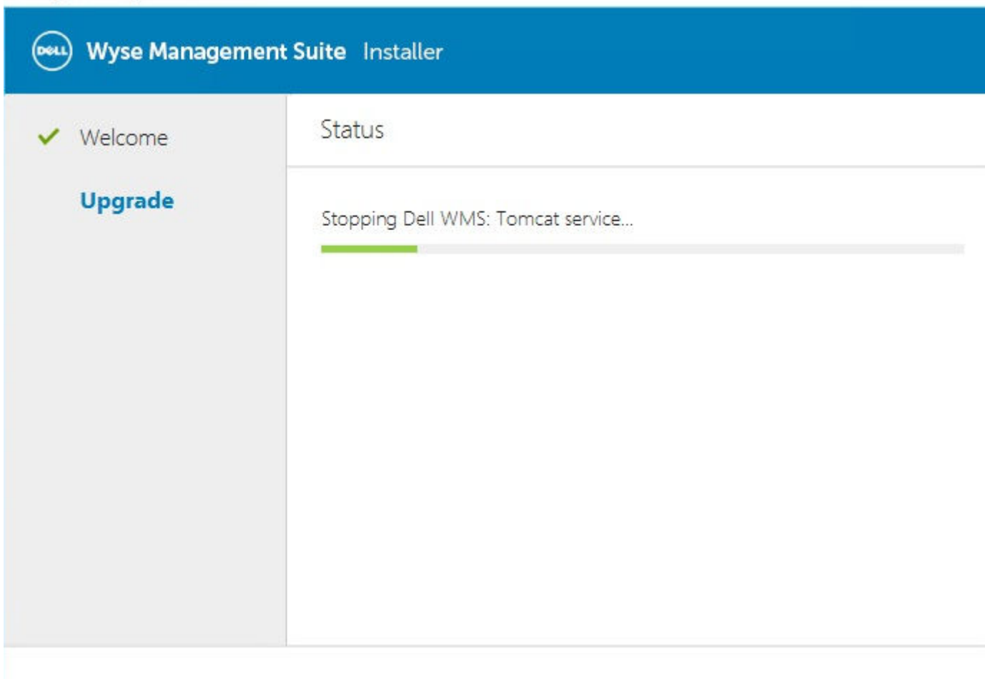
Figura 65. Actualización
