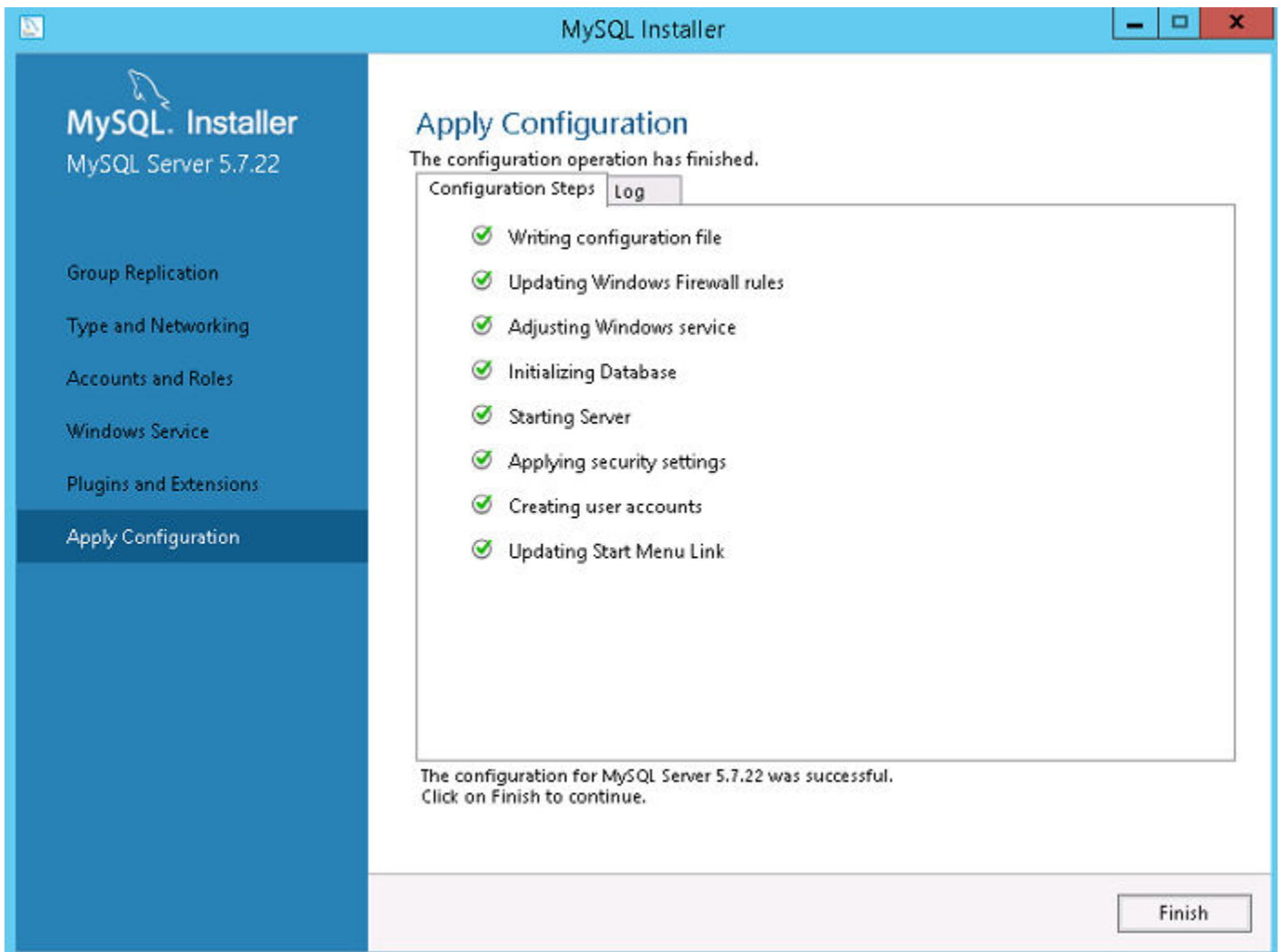
Figura 34. Aplicar configuraciones
