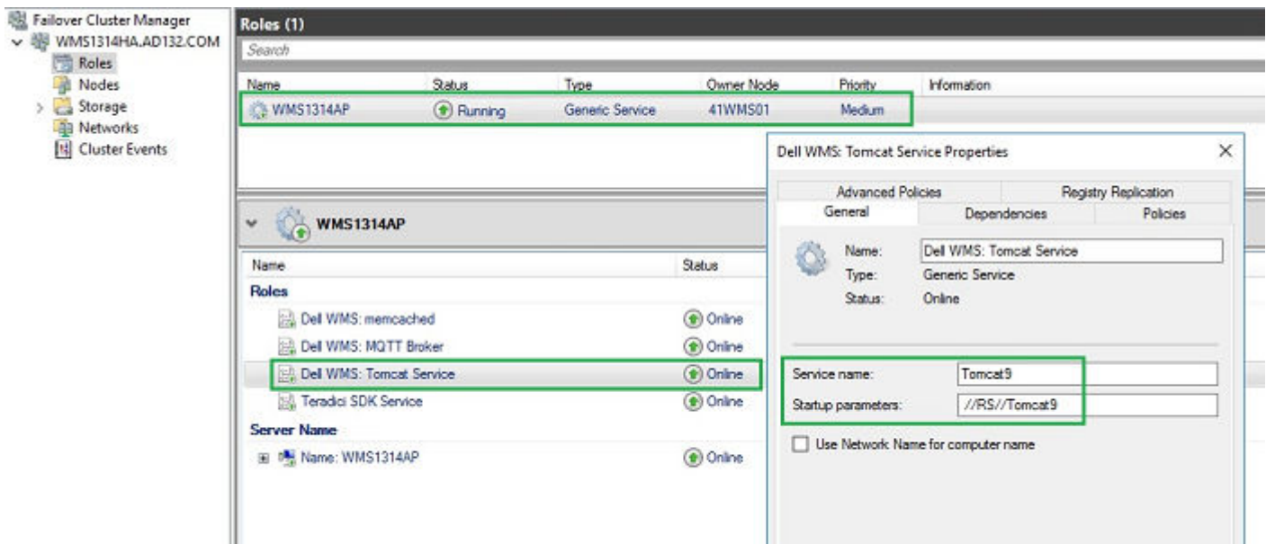
Figura 70. Servicio Tomcat 9
