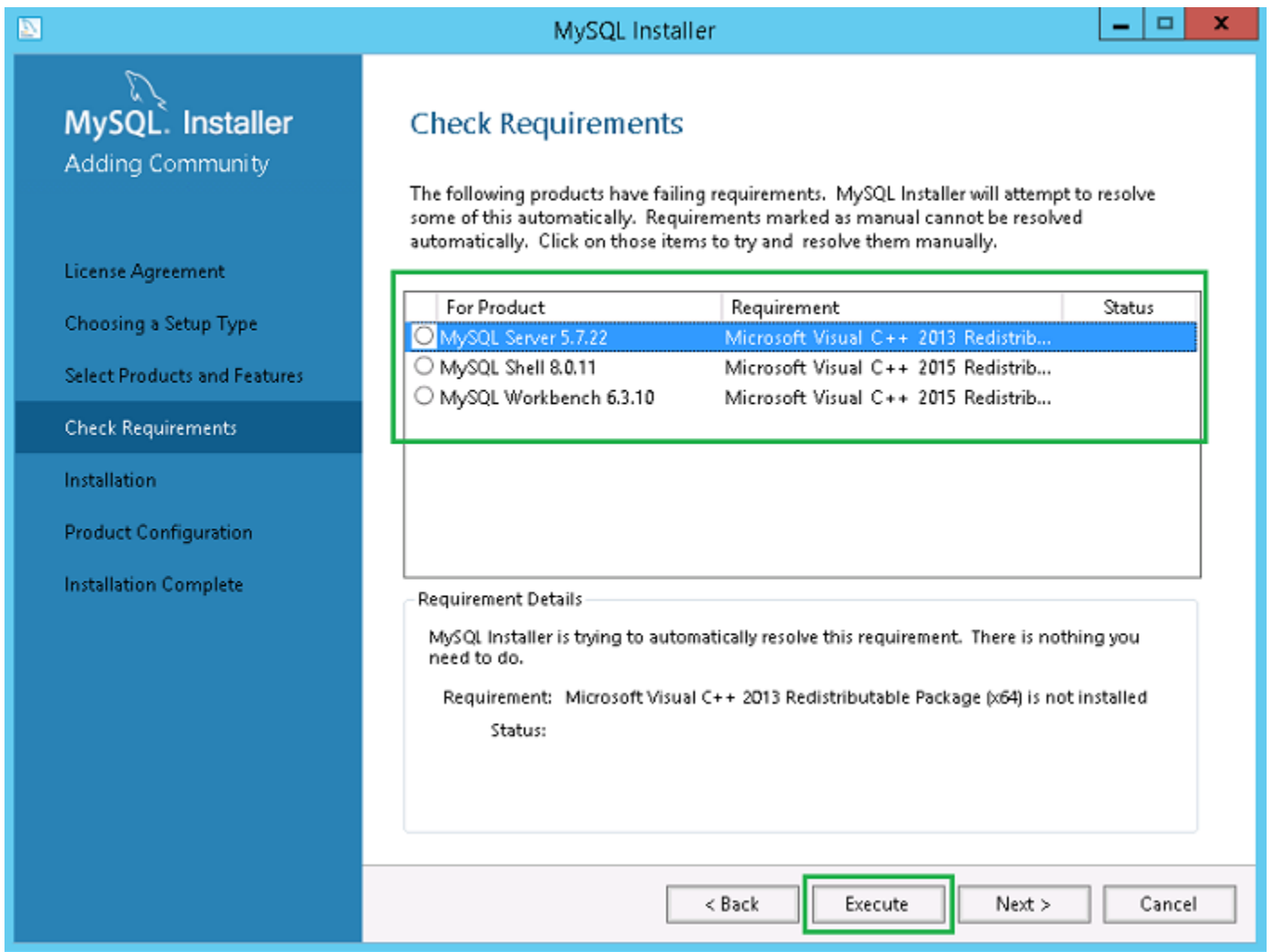
Figura 21. Requisitos
