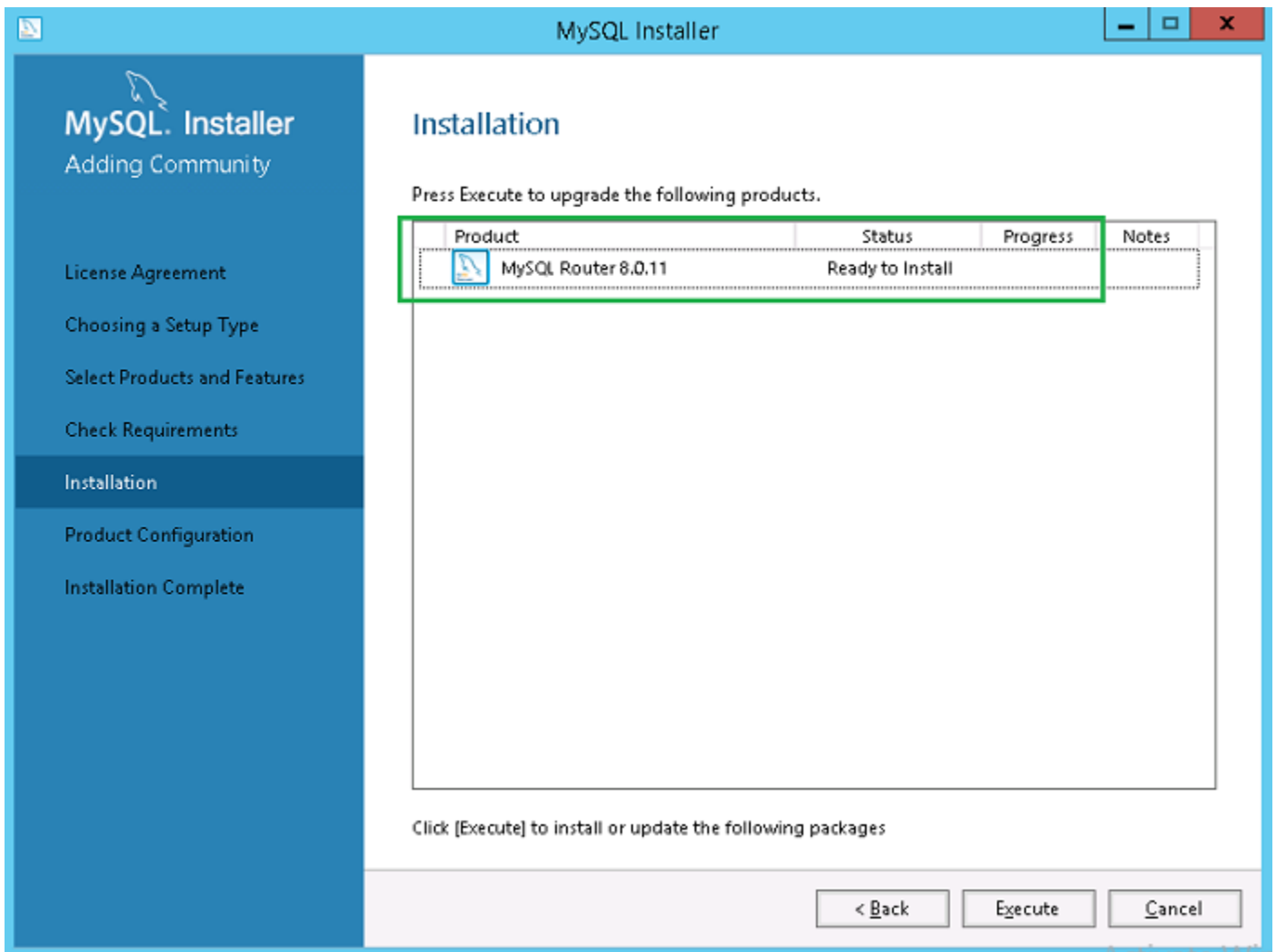
Figura 45. Instalación
