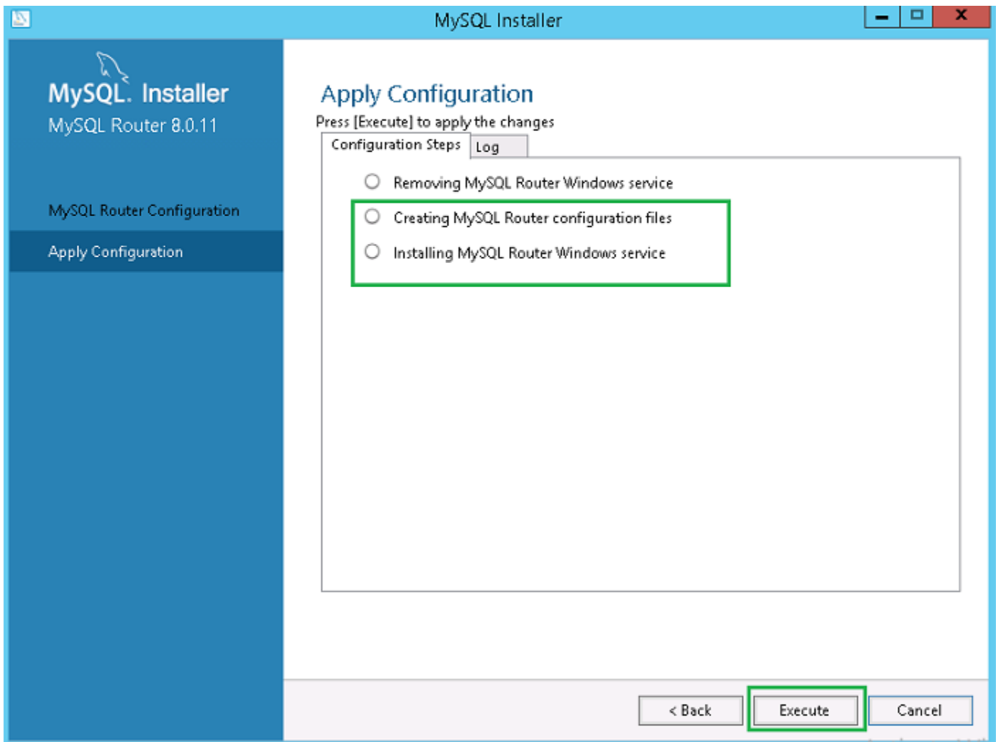
Figura 49. Aplicar configuración
