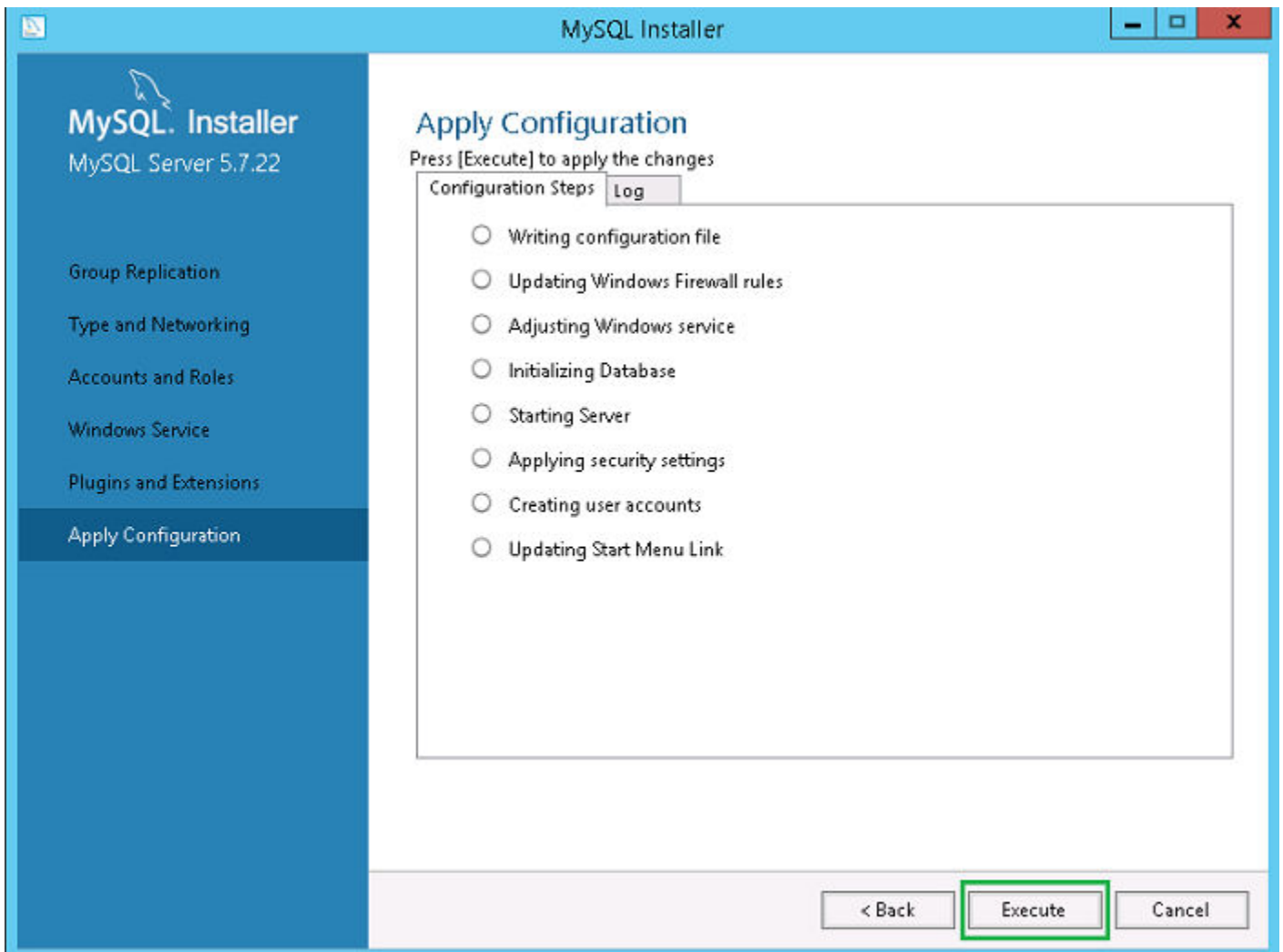
Figura 33. Aplicar configuraciones
