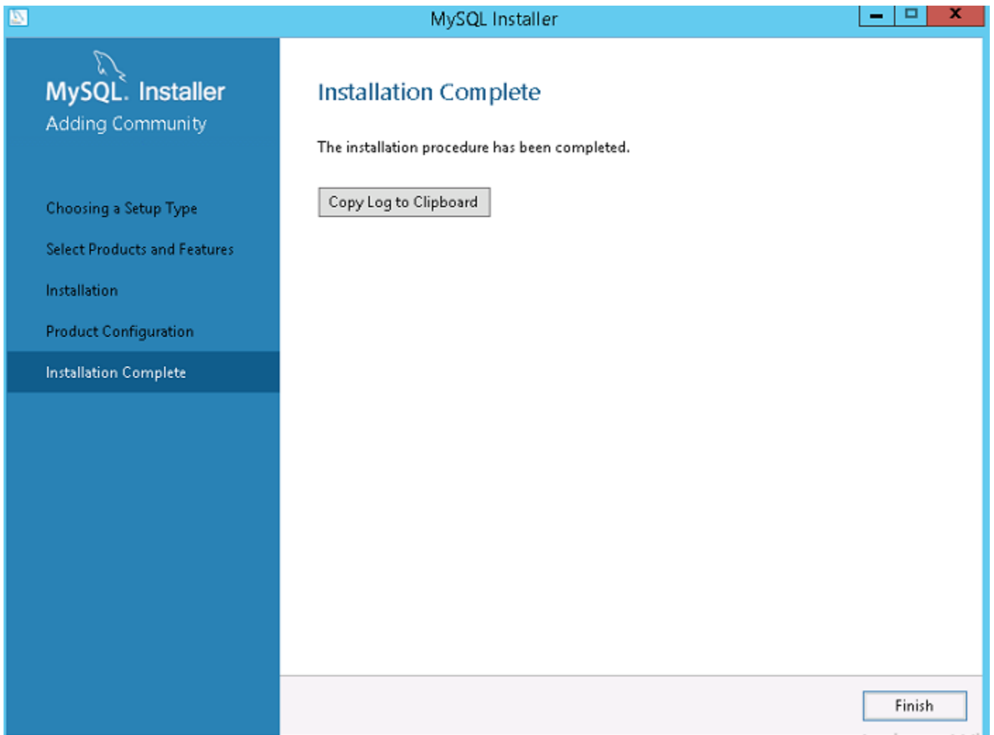
Figura 52. Instalación completa
