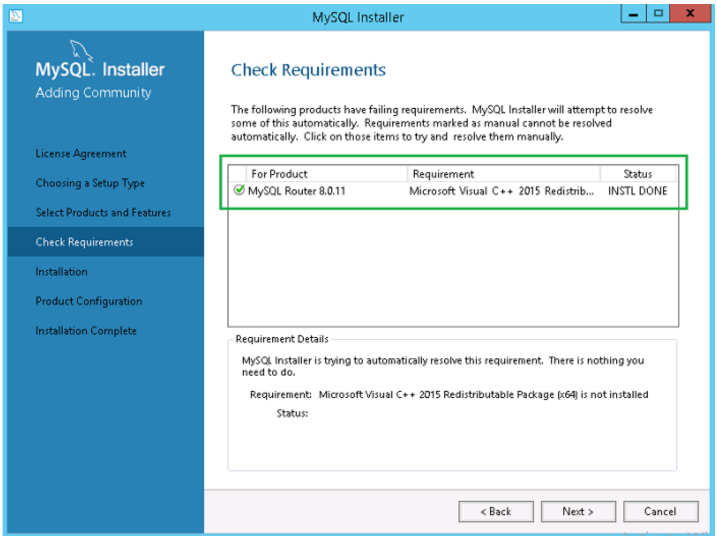
Figura 44. Verificar requisitos
