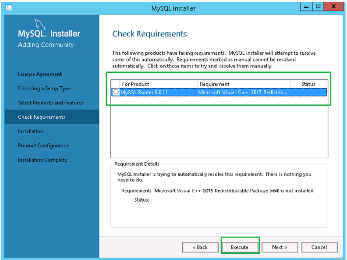
Figura 42. Verificar requisitos
