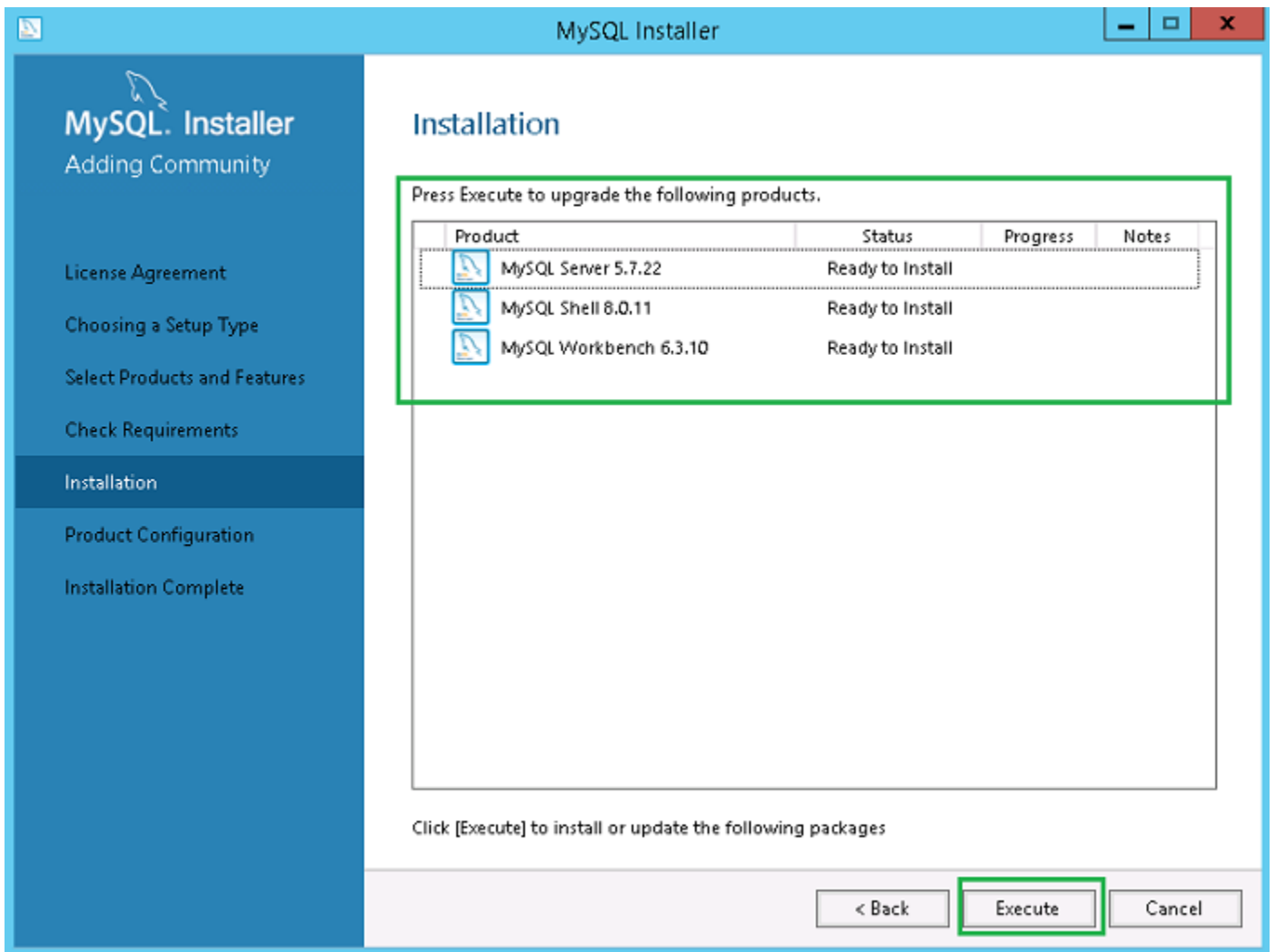
Figura 24. Instalación
