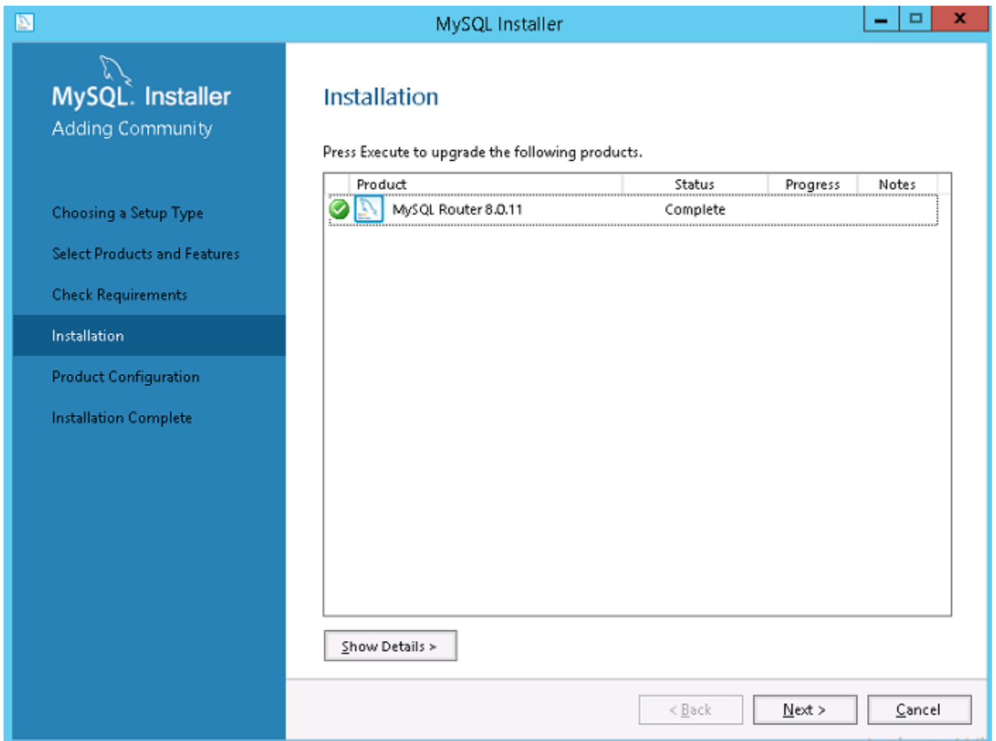
Figura 46. Instalación
