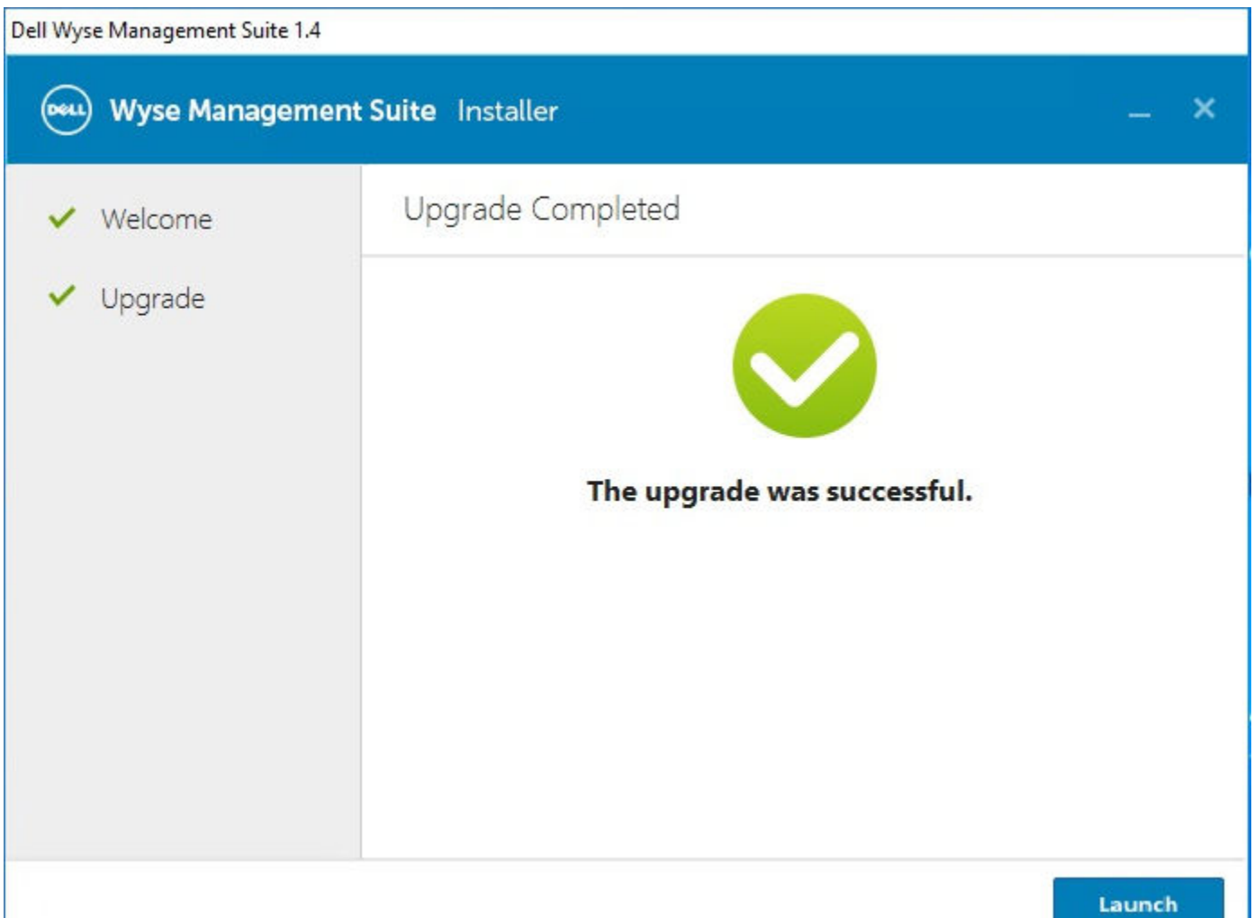
Figura 66. Iniciar
