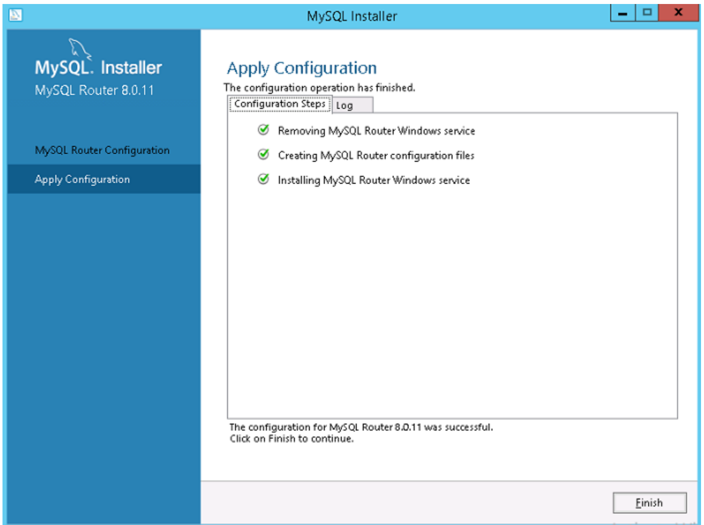
Figura 50. Aplicar configuraciones
