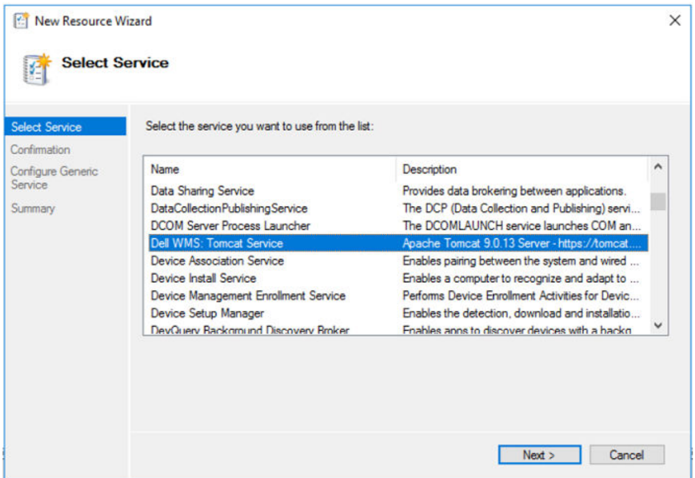
Figura 17. Seleccionar servicio
