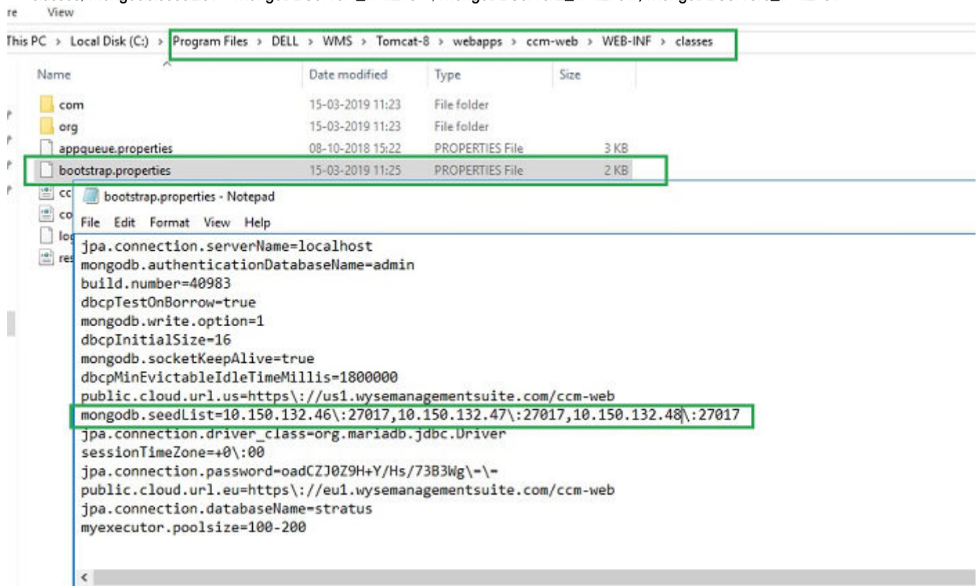
Figura 62. Prerrequisito
