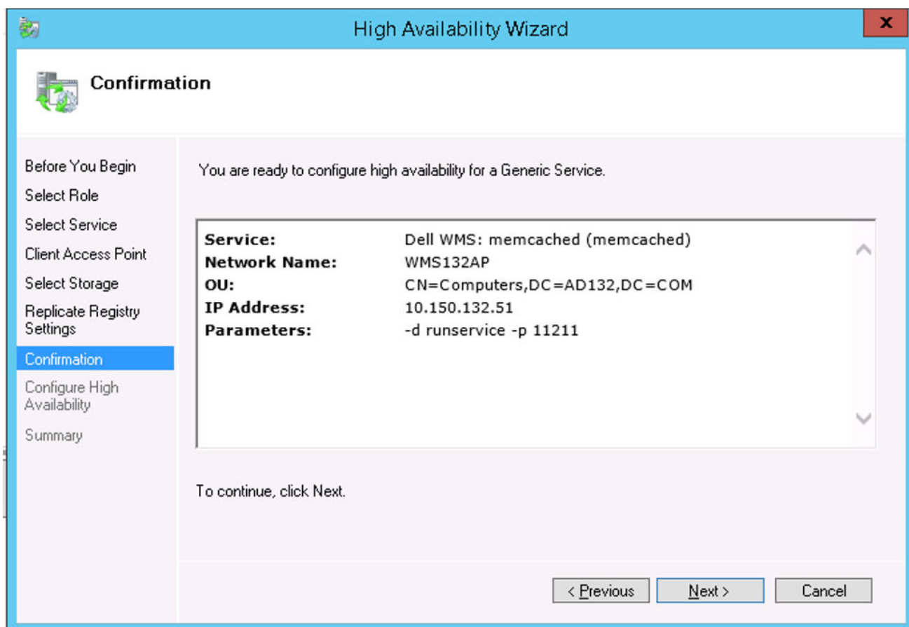
Figura 18. Confirmación
