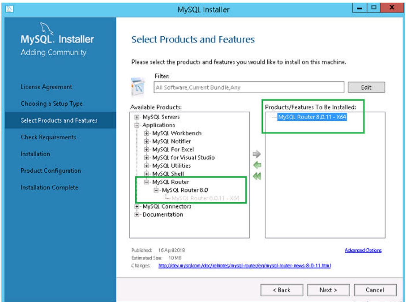
Figura 41. Seleccionar productos y funciones
