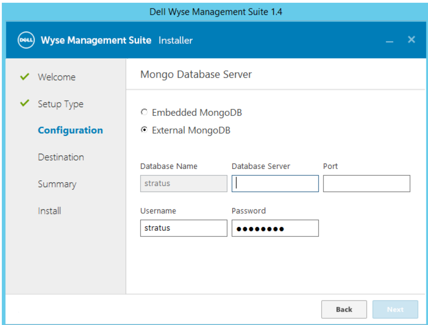
図 20. External MongoDB
