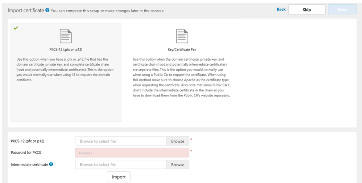
図 14. PKCS-12
