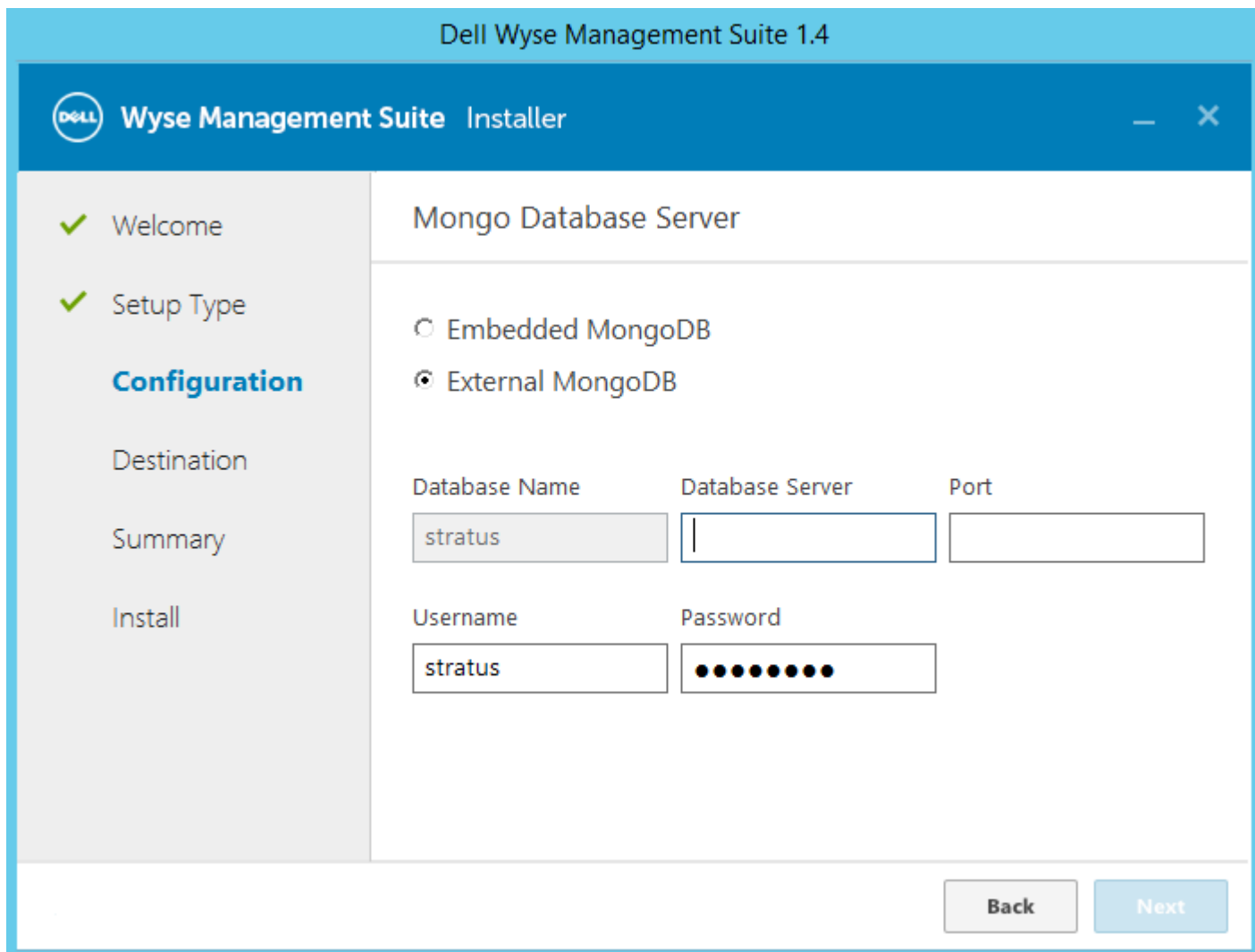
Figura 20. MongoDB externo
