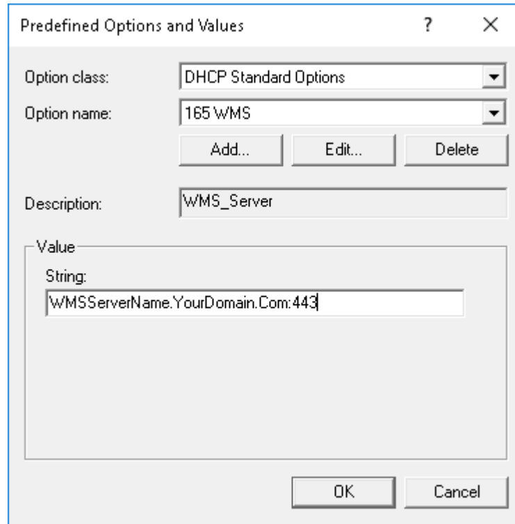
Abbildung 27. Option-Tag 165 Wyse Management Suite Server-URL
