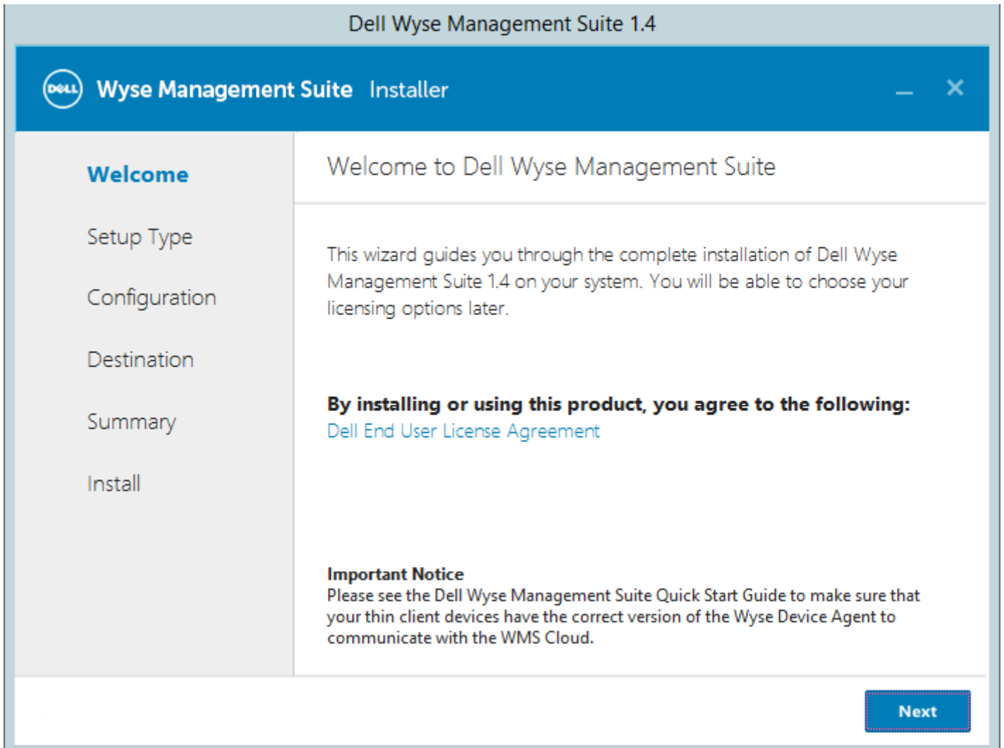
Abbildung 1. Willkommen-Bildschirm
