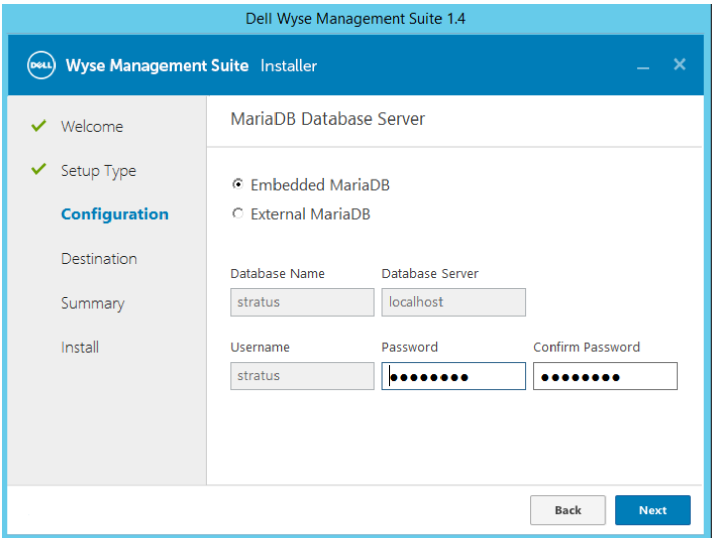
Abbildung 21. Integrierte MariaDB
