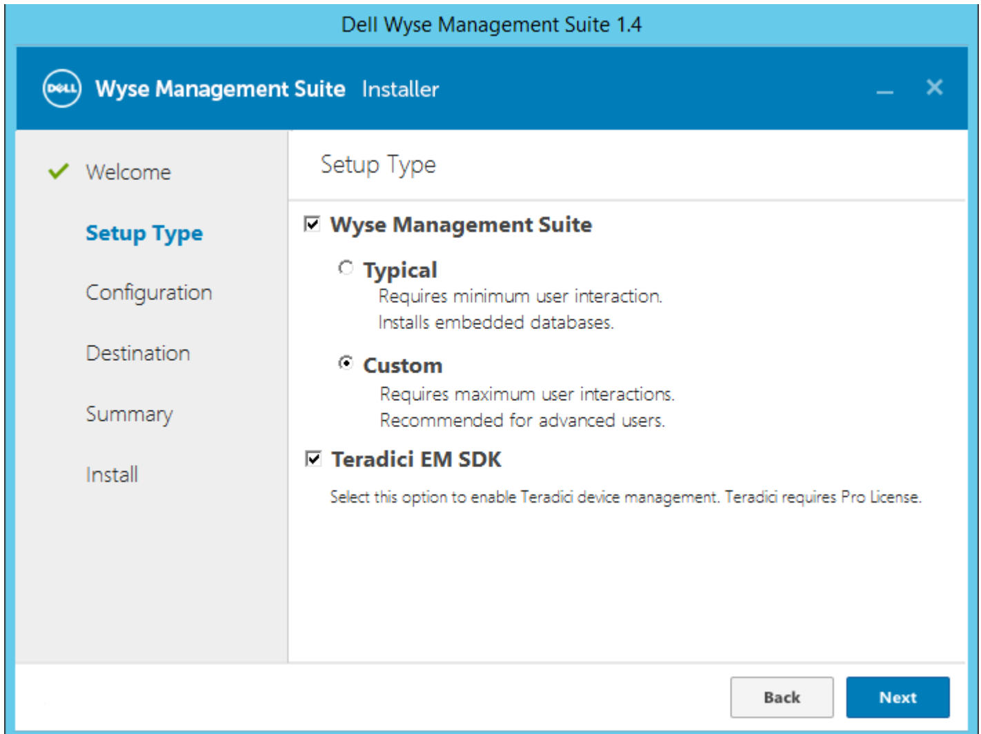
Abbildung 18. Setup-Typ
