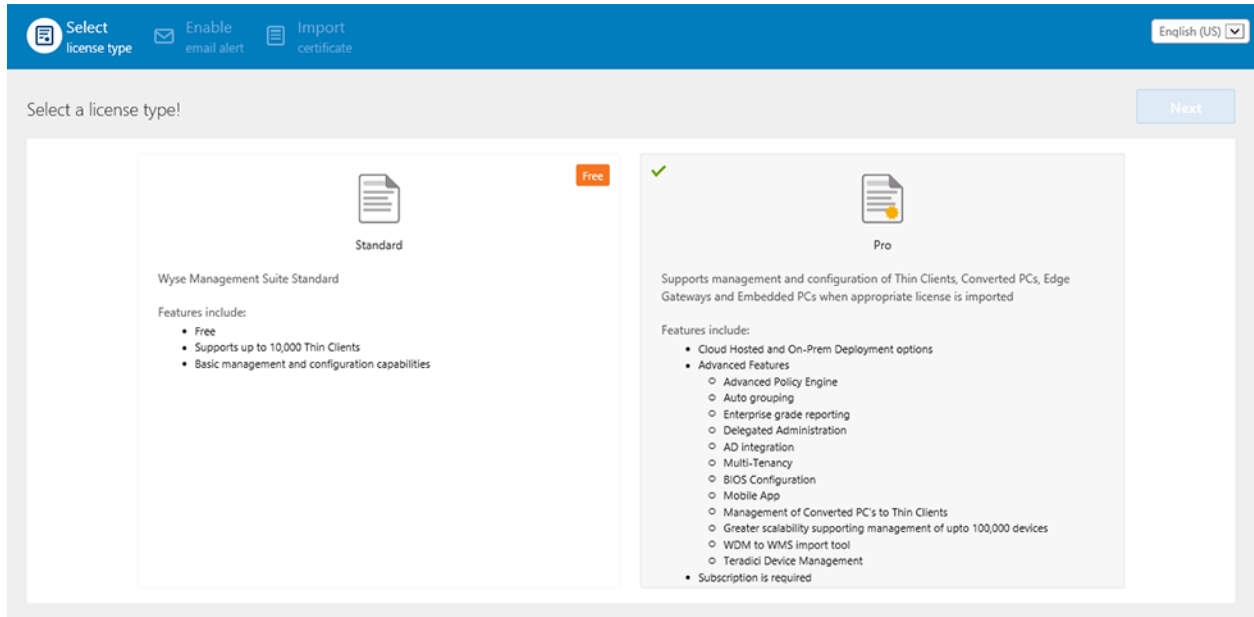
Abbildung 9. Lizenztyp
