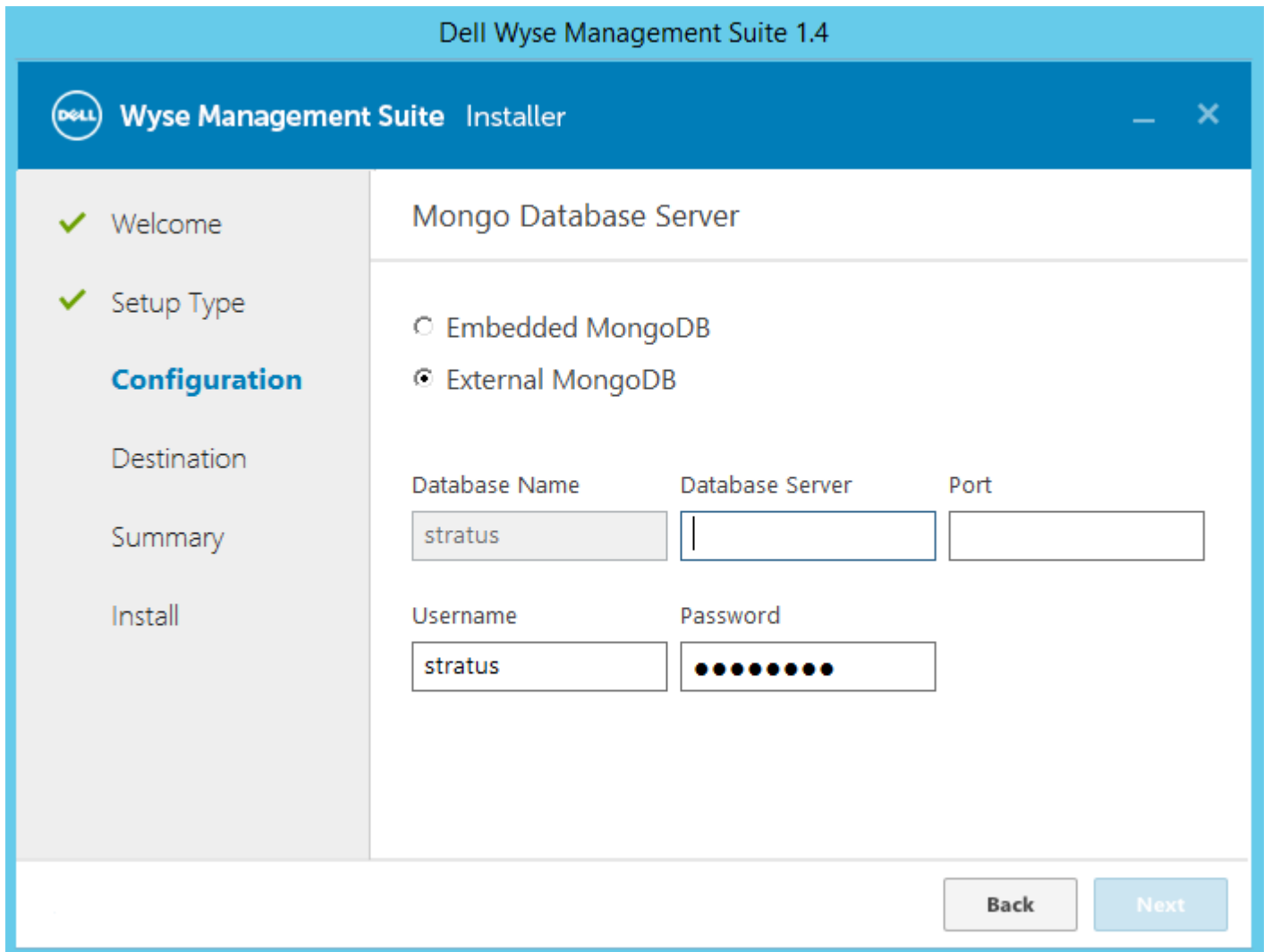
Abbildung 20. Externe MongoDB
