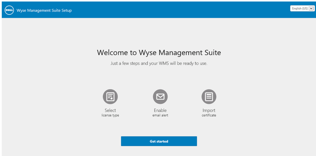
Abbildung 8. Startseite
