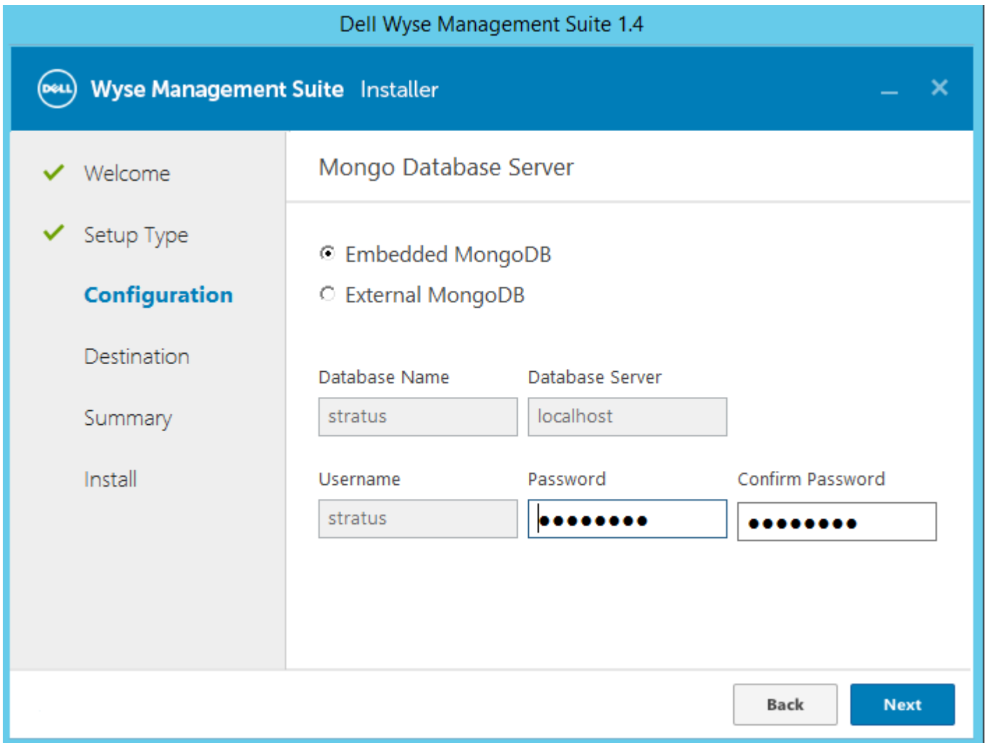
Abbildung 19. Integrierter Mongo-Datenbankserver
