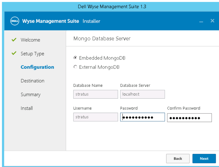
Abbildung 19. Integrierter Mongo-Datenbankserver
