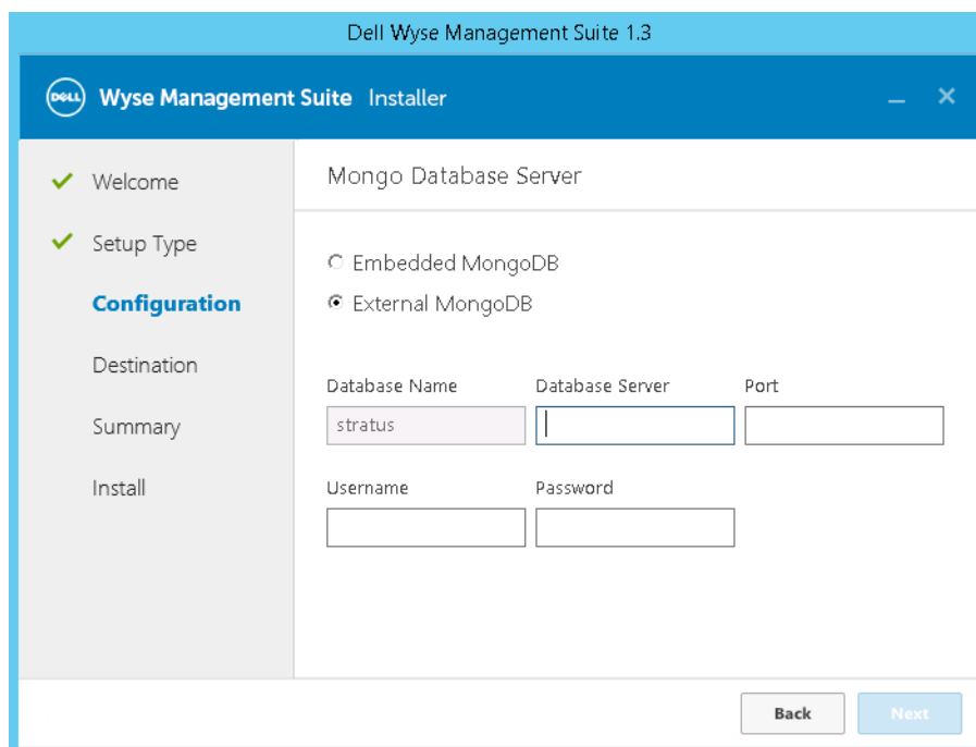
Abbildung 20. Externe MongoDB
