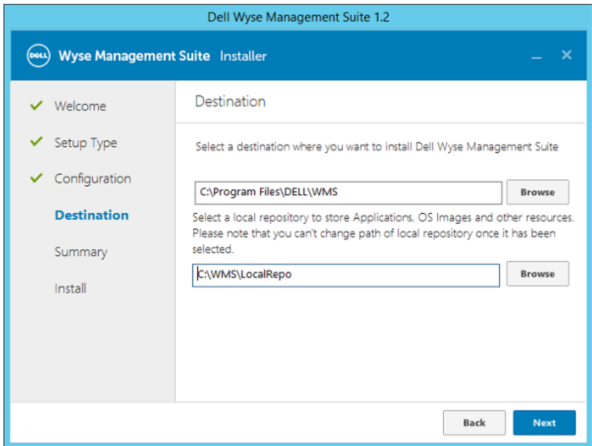
Abbildung 5. Ziel
