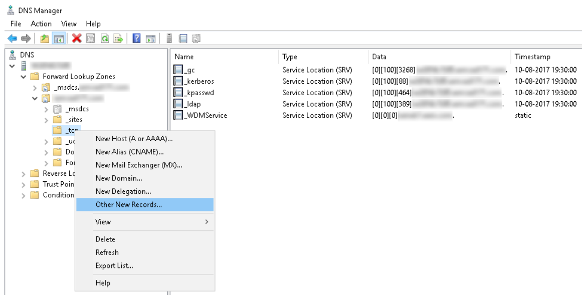
Ilustración 31. Administrador DNS
