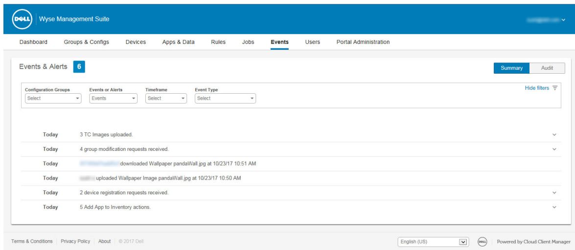
Abbildung 9. Ereignisse
