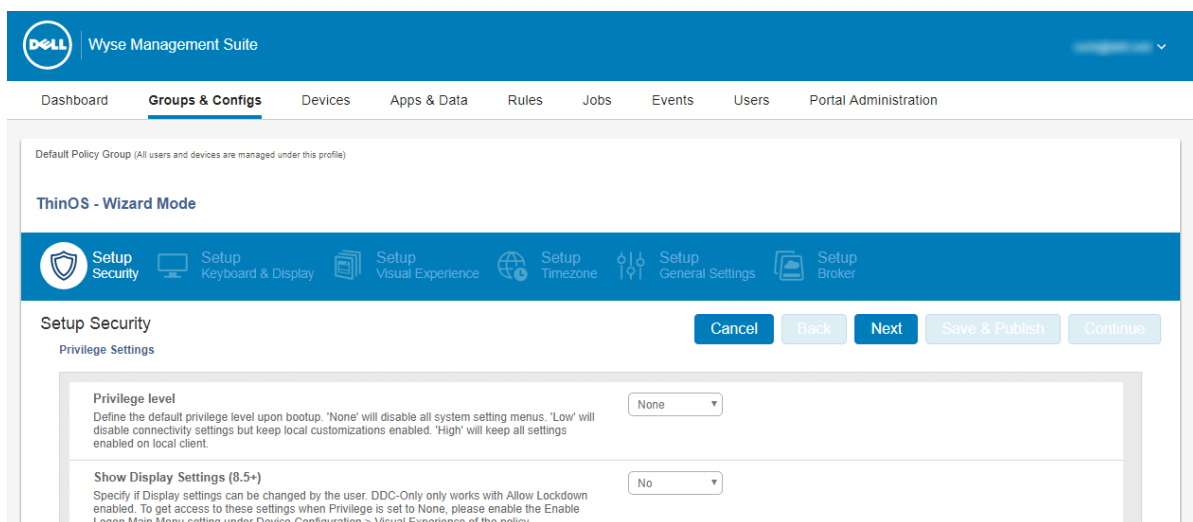
Abbildung 3. ThinOS – Assistentenmodus
