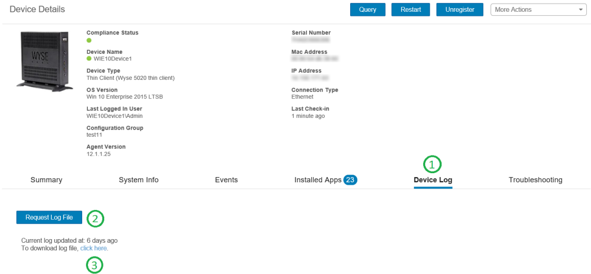
그림 7. 로그 파일 가져오기
