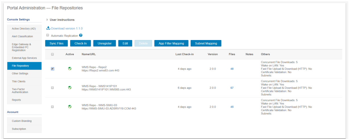
그림 11. 파일 리포지토리
