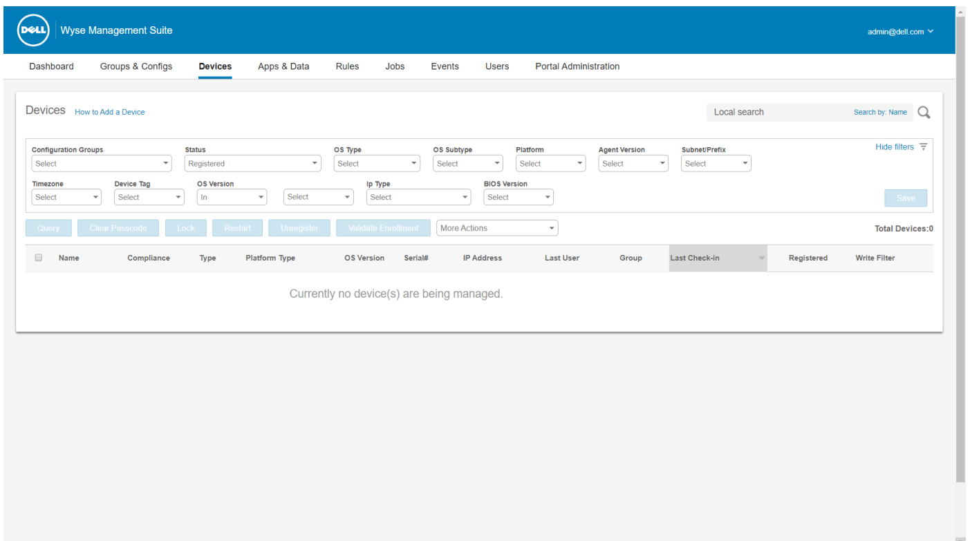
그림 4. 디바이스 페이지
