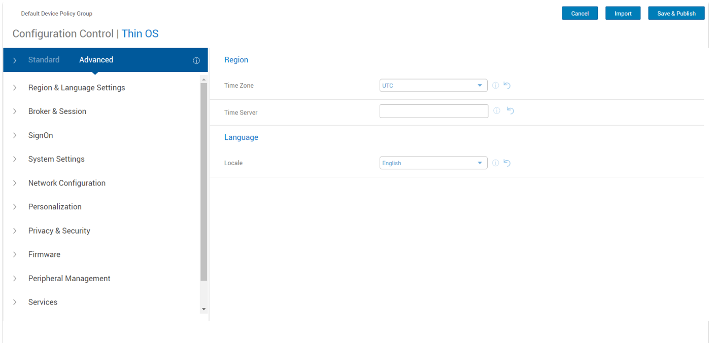
그림 3. 고급 옵션
