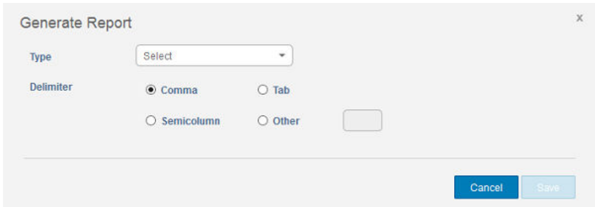
图 17: 生成报告
