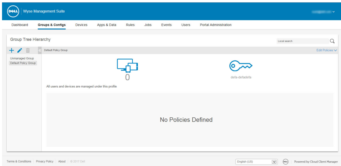
图 2: 组和配置
