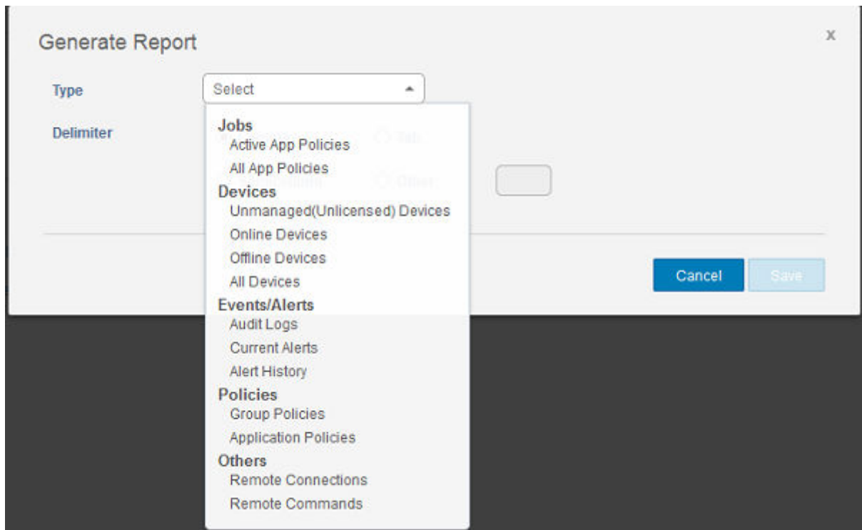
图 18: 报告类型
