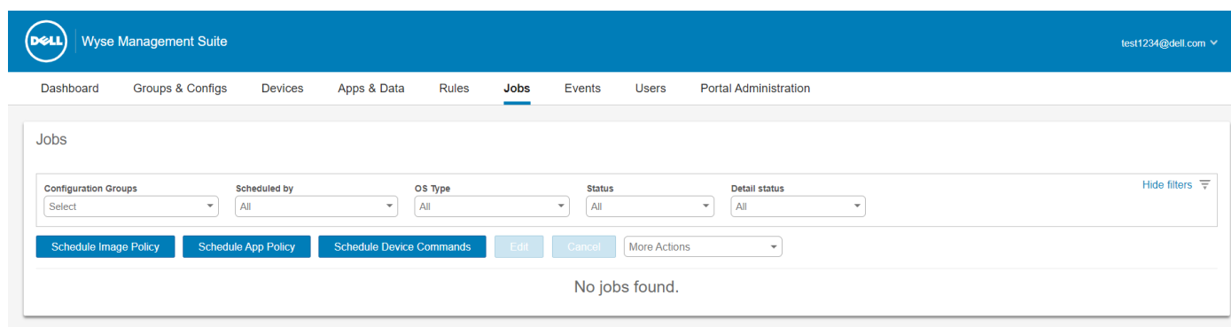
Abbildung 12. Seite „Jobs“
