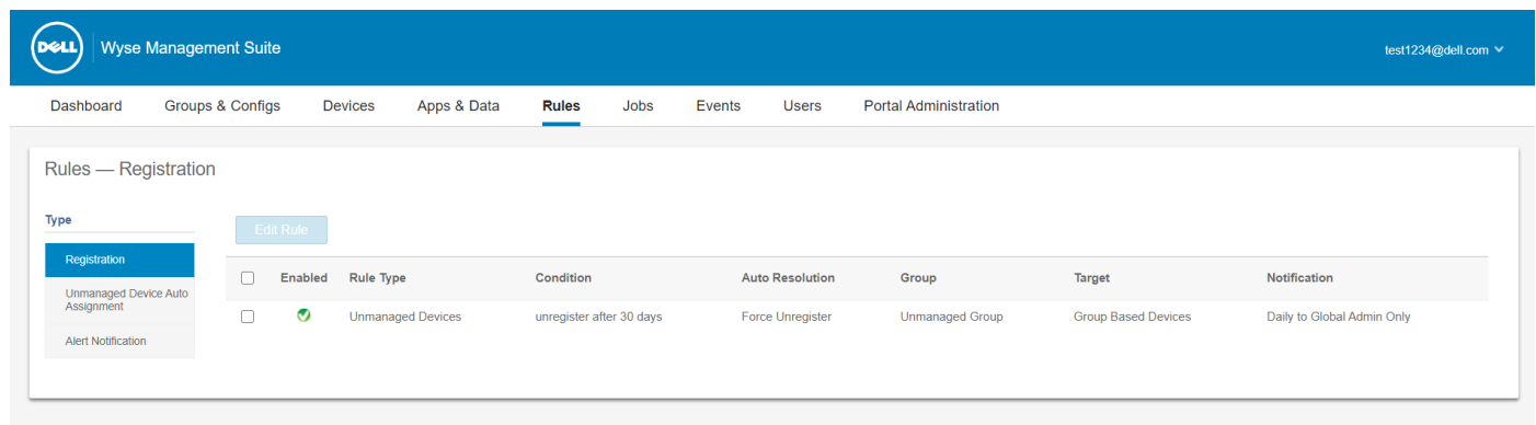
Abbildung 11. Seite „Regeln“
