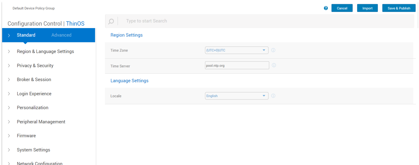
Abbildung 5. Konfigurationssteuerung | ThinOS
