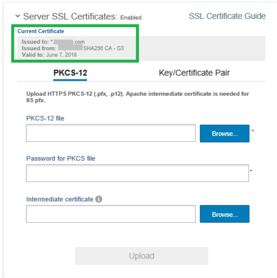
그림 19 . SSL 인증서 활성화
