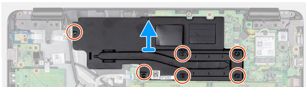
6x M2x3
