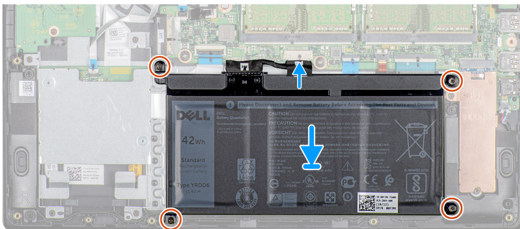
4x M2x3
