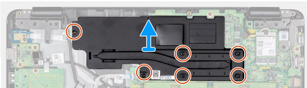
6x M2x3
