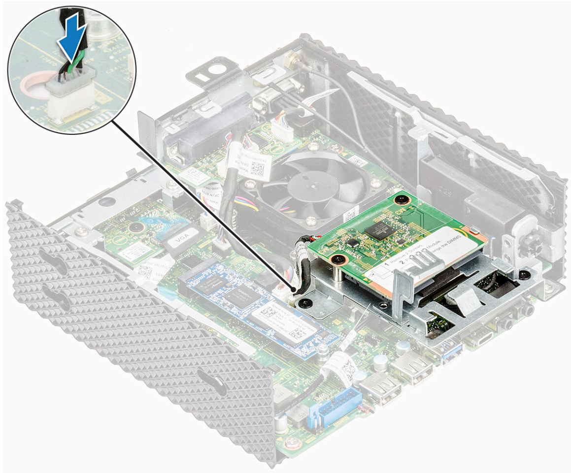
Figur 21. Koble til CAC-kabelen
