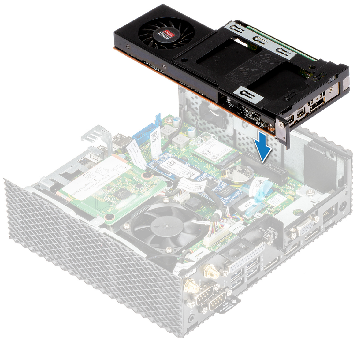
Figur 15. Juster PCIe-modulen
