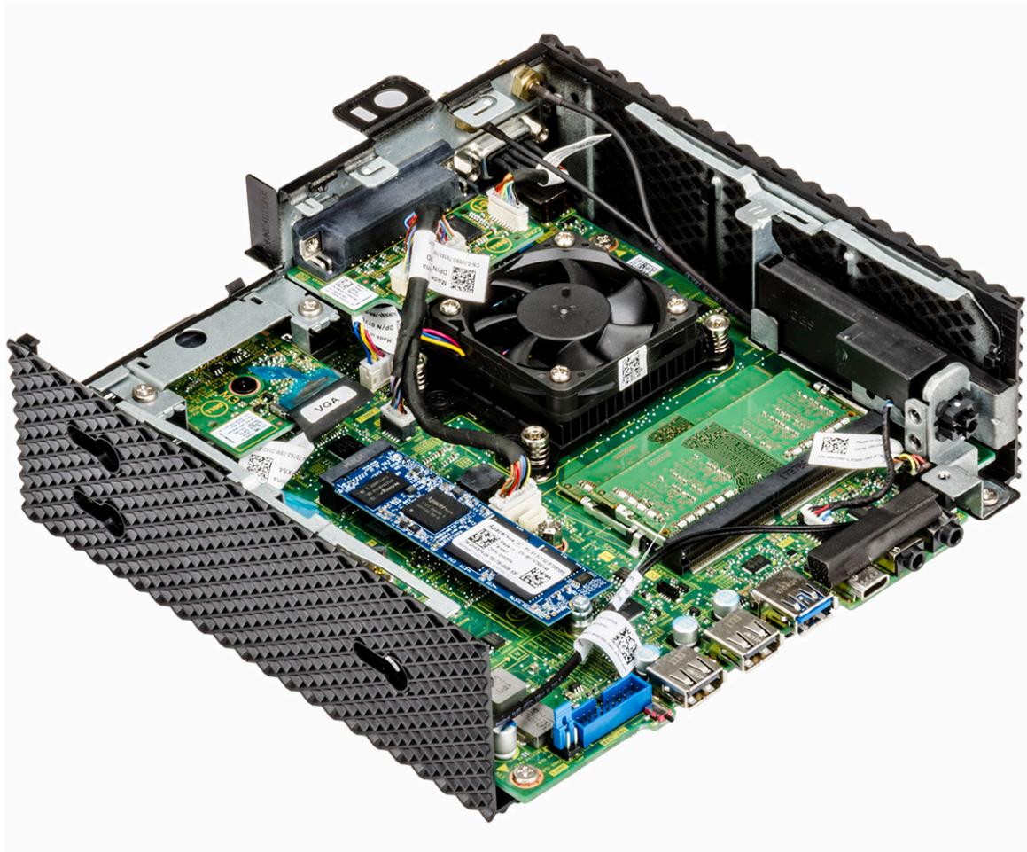
Figur 19. CAC-leseren er fjernet
