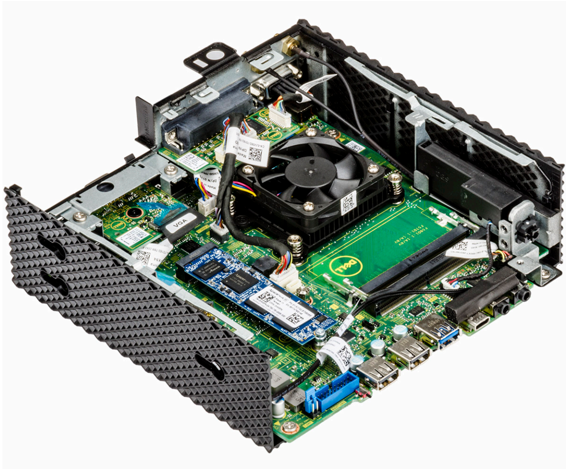
Figur 23. Minnekortene er fjernet
