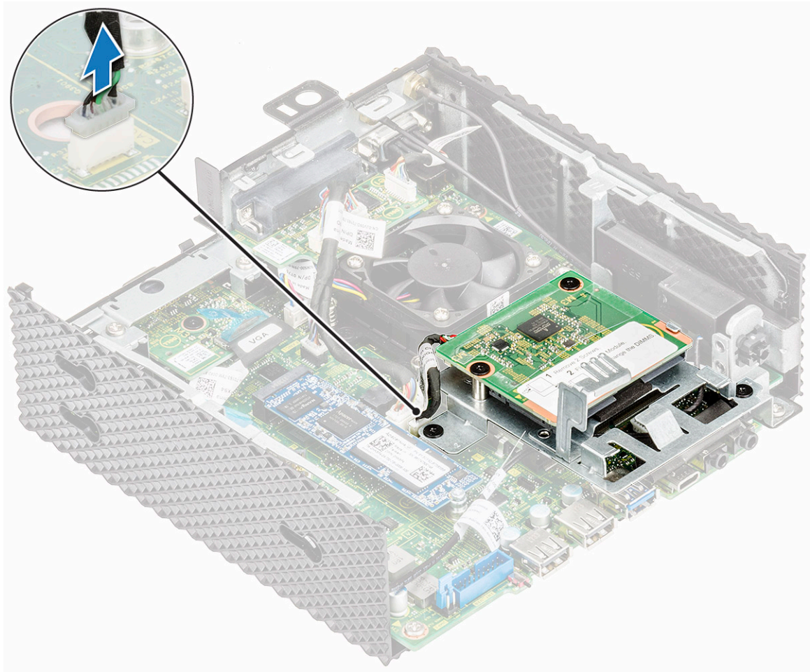
Figur 17. Koble fra kabelen
