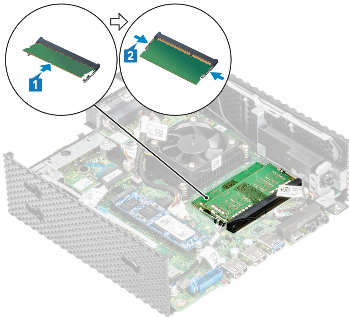
Figur 24. Installere minnemodulen
