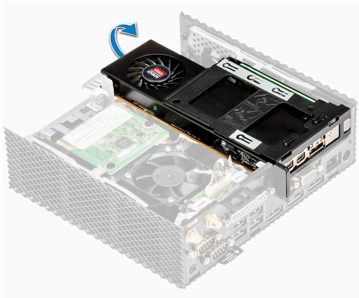
Figur 13. Ta ut PCIe-modulen
