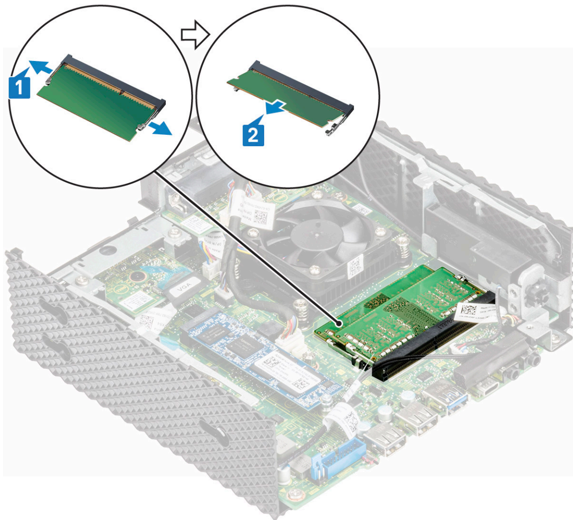
Figur 22. Ta ut minnemodulen
